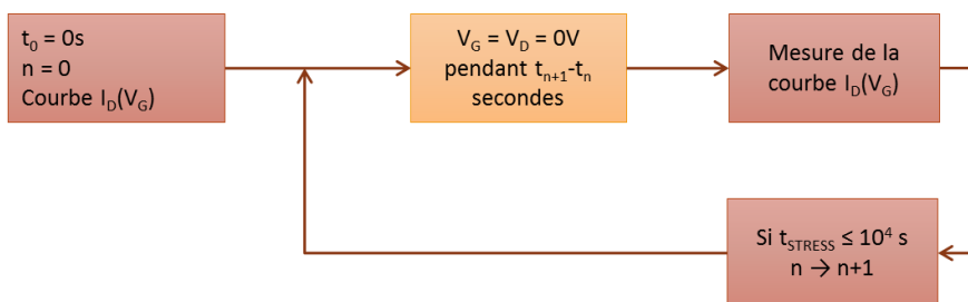
Figure 2-25 : Représentation schématique d'un stress électrique « nul » avec V_{G\_STRESS} = V_{D\_STRESS} = 0V .
