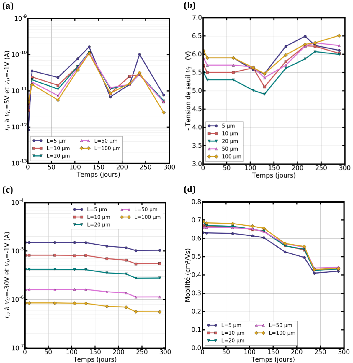
Figure 2-28 : Evolution (a) du courant I_{OFF} ( V_G=+5V , V_D=-1V ), (b) de la tension de seuil V_T , (c) du courant I_{ON} ( V_G=-30V , V_D=-1V ) et (d) de la mobilité \mu des OTFTs du module A au cours du temps, en stockage dans le noir, à l'air et température contrôlée, pour différentes longueurs de canal. W = 2000 \mu m , L varie entre 5 et 100 \mu m .
