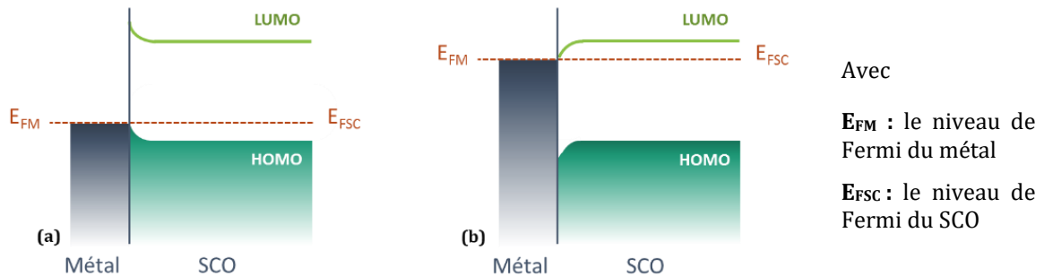
Figure 1-10 : Alignement des niveaux d'énergie lors d'un contact métal/semi-conducteur organique (a) de type p et (b) de type n – adapté de [7].
