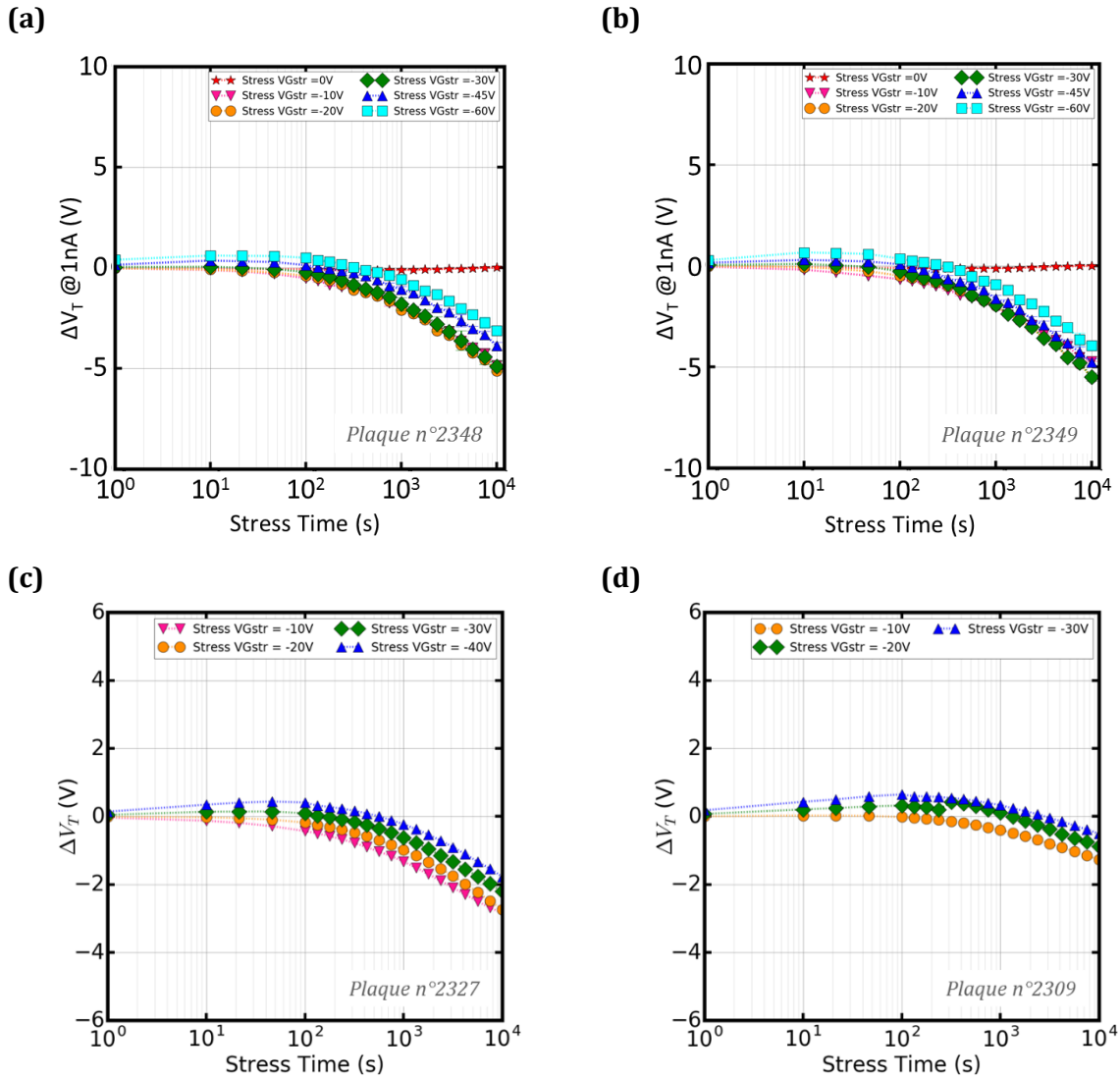
Figure VI-1 : Evolution de \Delta V_T lors du stress électrique sur des P-OTFTs avec une grille en encre argent imprimée par sérigraphie provenant de plaques (a), (b) Backplane avec W=500\mu m et L=20\mu m et (c), (d) Polaris avec W=4000\mu m et L=20\mu m .
