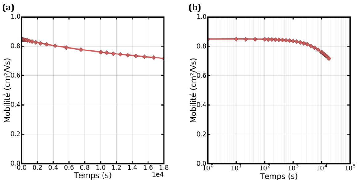
Figure 2-33 : Evolution de la mobilité d'un transistor pendant 5h d'exposition à la lumière du microscope (a) en échelle linéaire et (b) en échelle logarithmique. W = 500 μm, L = 20 μm.
