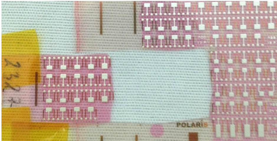
Figure 2-31 : Photos de transistors constatant l'évolution de couleur du semi-conducteur au cours du temps. A gauche, le module B stocké dans une boîte à part, à droite le reste de la même plaque également stockée dans le noir mais utilisée ponctuellement pour des mesures annexes et donc plus exposée à la lumière.
