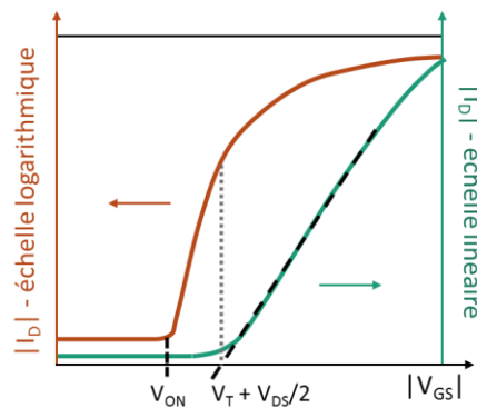
Figure 1-14 : Extractions des tensions V_T et V_{ON} à partir des courbes de transfert en échelle linéaire et semi logarithmique.
