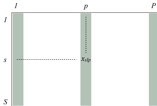
Figure 22: Matrice contenant les partitions finales sur les stimuli fournies par les évaluateurs. La valeur x_{slp} correspond à la description du groupe auquel appartient le stimulus s pour l'évaluateur p à la fin de la tâche de Tri Séquentiel Agglomératif (c.-à-d. lors de la présentation du l -ème sous ensemble).
