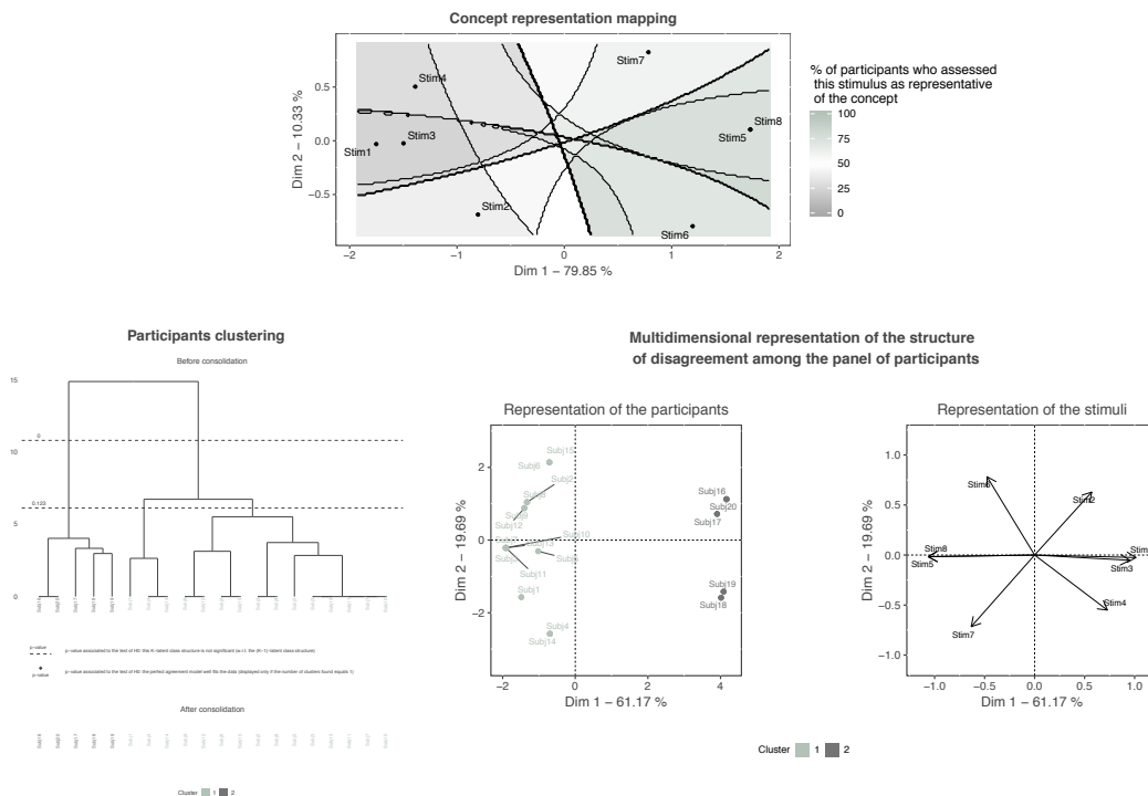
Figure 92: Jeu de données pédagogique du package BinQmet : Sorties graphiques de la fonction AnalyseBinQmet . Les résultats du haut sont ceux de la procédure statistique orientée stimuli et les résultats du bas sont ceux de la procédure statistique orientée évaluateurs.
