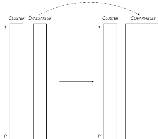
Figure 87: Jeu de données utilisé pour la description des clusters par des covariables sur les évaluateurs. Il présente les clusters des évaluateurs et les valeurs prises par les covariables disponibles sur les évaluateurs.
