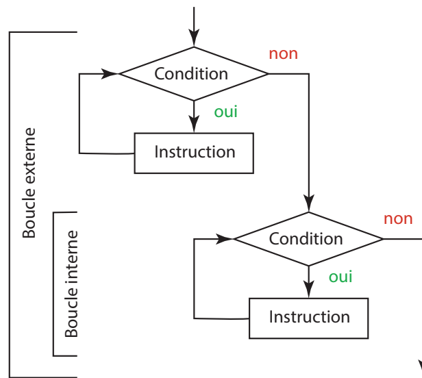
Figure 9.19 – Boucles imbriquées
