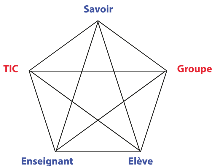
Figure 6.8 – Pentaèdre didactique
