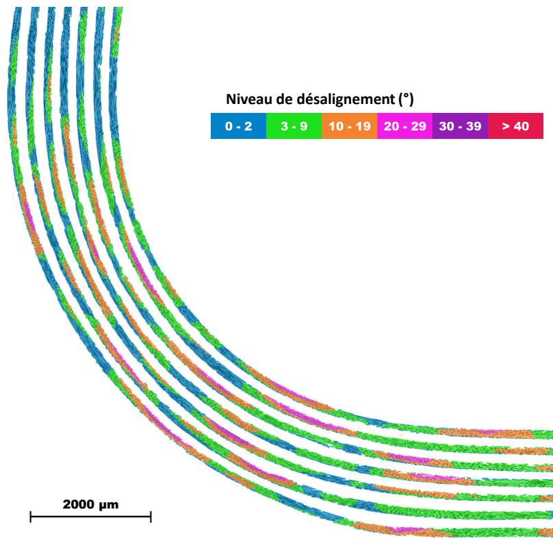
Figure B.2 – Désalignement des plis orientés à 0° dans une cornière thermo-pliée R7/R9
