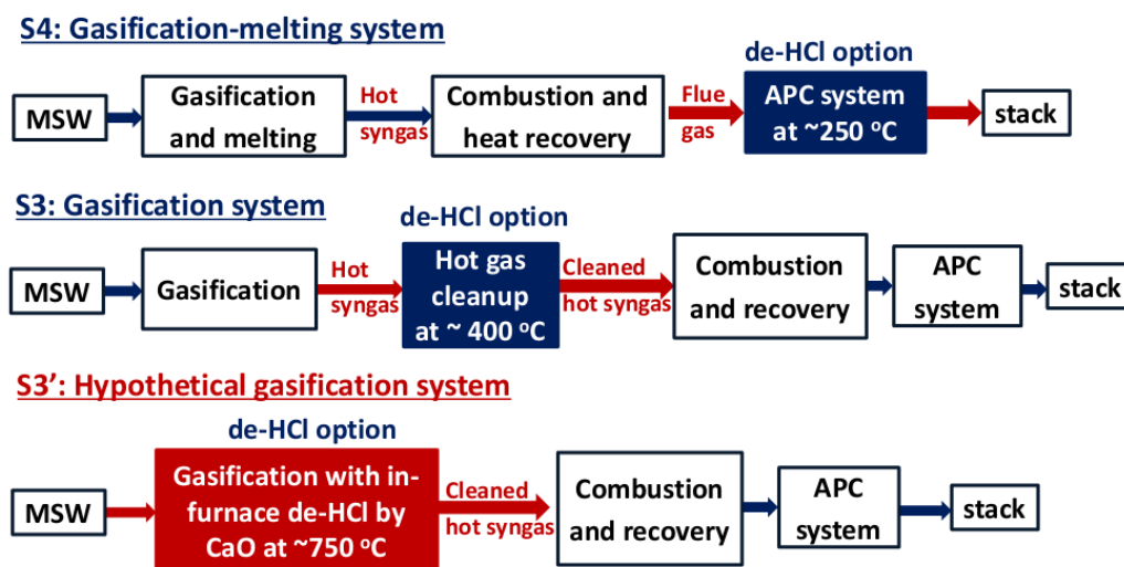
Figure 7.0.2 Présentation des 3 scénarios couplant le traitement thermique des résidus solides avec l'abattement du chlore, par méthode ex-situ ou in-situ : S4, gazéification avec fusion des cendres puis traitement du chlore ex-situ à basse température (APC) ; S3, gazéification puis épuration du chlore ex-situ à haute température ; et S3', gazéification et abattement du chlore in-situ en présence du réactif CaO
