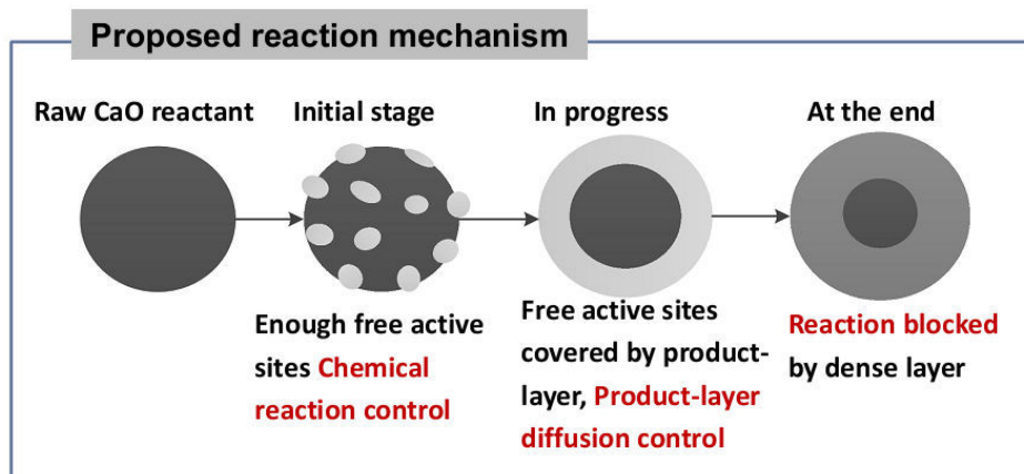
Figure 3.0.1 Mécanisme de réaction entre CaO et HCl proposé : le premier régime correspond à une limitation de la cinétique par la réaction hétérogène de surface, laquelle conduit à la formation de \text{CaCl}_2 (en gris clair). Plus la réaction avance, plus le réactif CaO est converti en \text{CaCl}_2 qui représente une couche s'épaississant à la surface du CaO qui n'a pas encore réagi. Ceci traduit que la diffusion de HCl à l'intérieur de cette couche ainsi formée devient l'étape limitante du processus. L'augmentation de densité de la couche, observée notamment par microscopie électronique à balayage, bloque la réaction en inhibant la diffusion.
