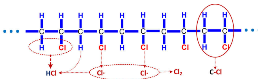
Figure 5.0.1 Mécanisme de formation des composés chlorés lors de la pyrolyse du PVC
