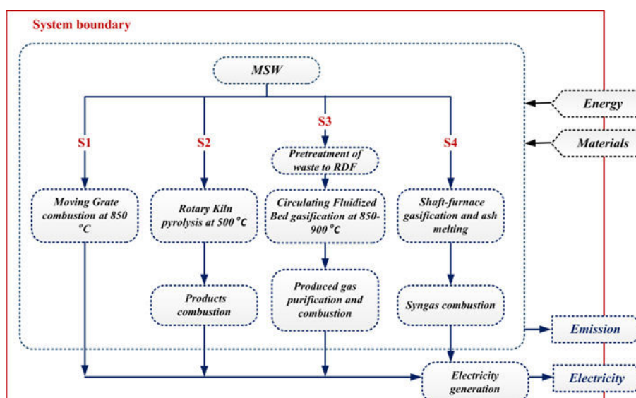
Figure 7.0. 1 Périmètre d'étude des 4 scénarios évalués: S1 = incinération, S2 = pyrolyse, S3 = gazéification et S4 = gazéification et fusion de cendres
