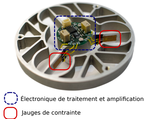
Figure 2.8: Capteur de force
