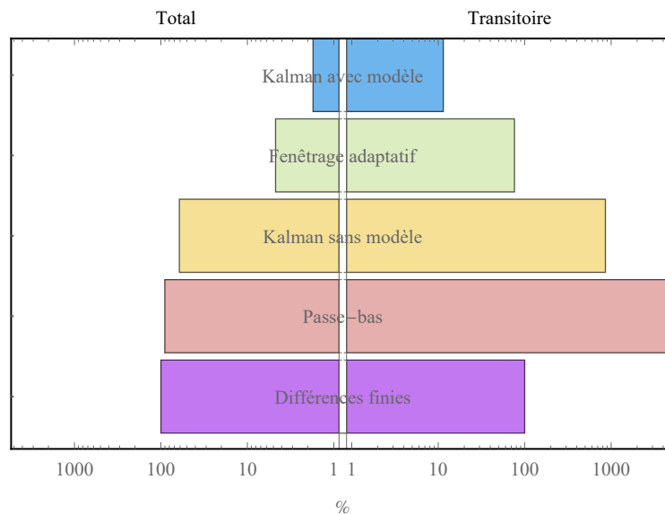
Figure 2.6: Histogramme de synthèse sur les méthodes d'estimation de vitesse
