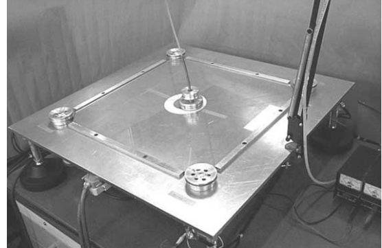
(b) Interface Feriba3 (GALLINA, ROSATI et ROSSI, 2001)
