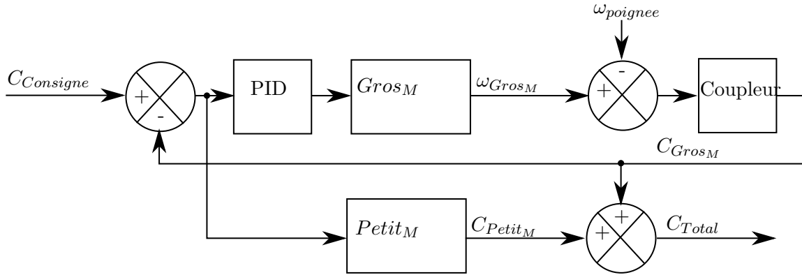
Figure 1.14: Schéma de fonctionnement de l'interface
