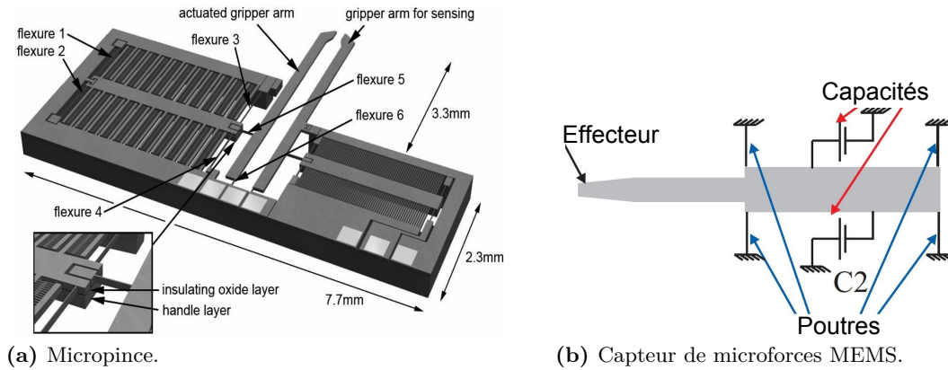
Figure B.13: Capteurs de forces capacitifs.
