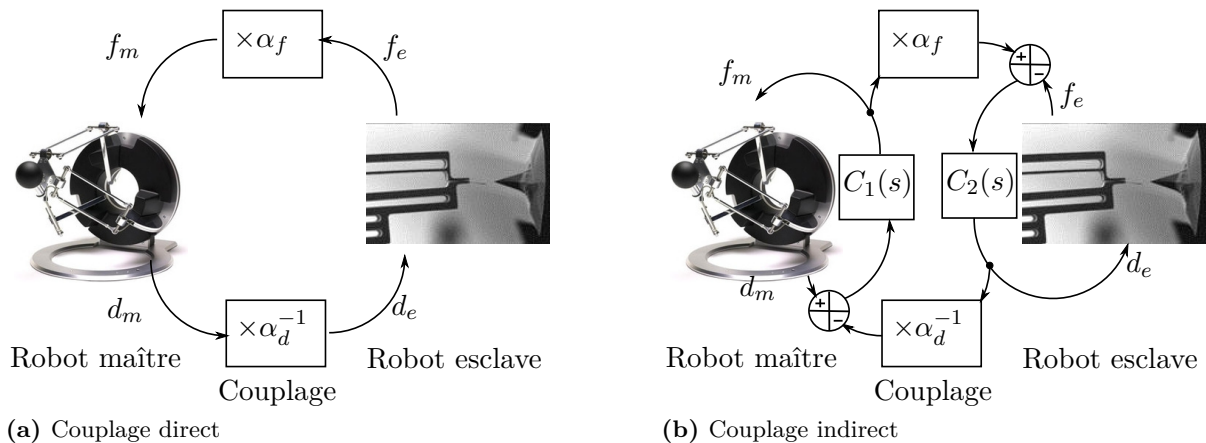
Figure 1.7: Schémas de couplage
