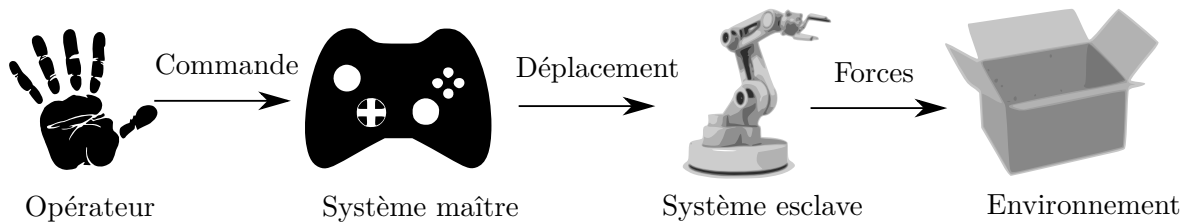
Figure 1.2: Chaîne de téléopération sans retour
