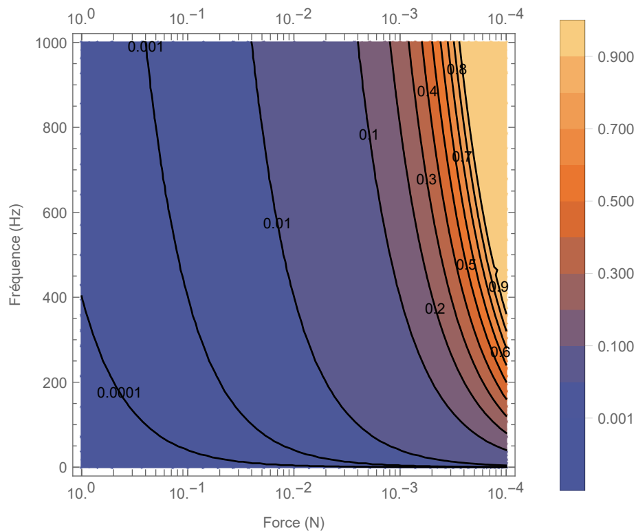
Figure 3.13: Tracé de l'erreur en fonction de la force et de la fréquence
