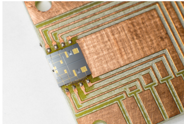
Figure 3.9: Deuxième prototype monté sur un PCB
