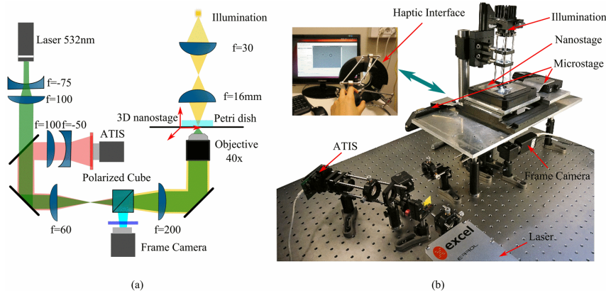
Figure B.6: Pinces optiques utilisées à l'ISIR
