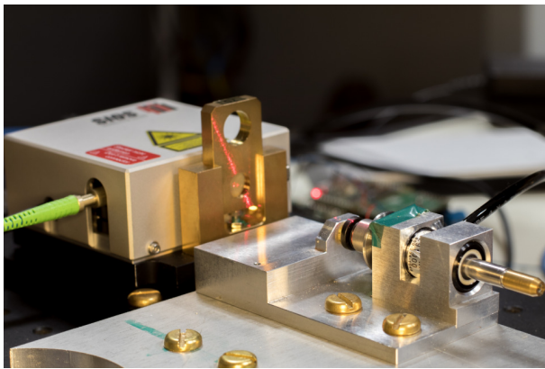
(a) Capteur monté avec l'interféromètre
