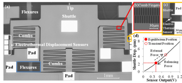
Figure B.20: Capteur développé en version MEMS (COSKUN et al., 2014)
