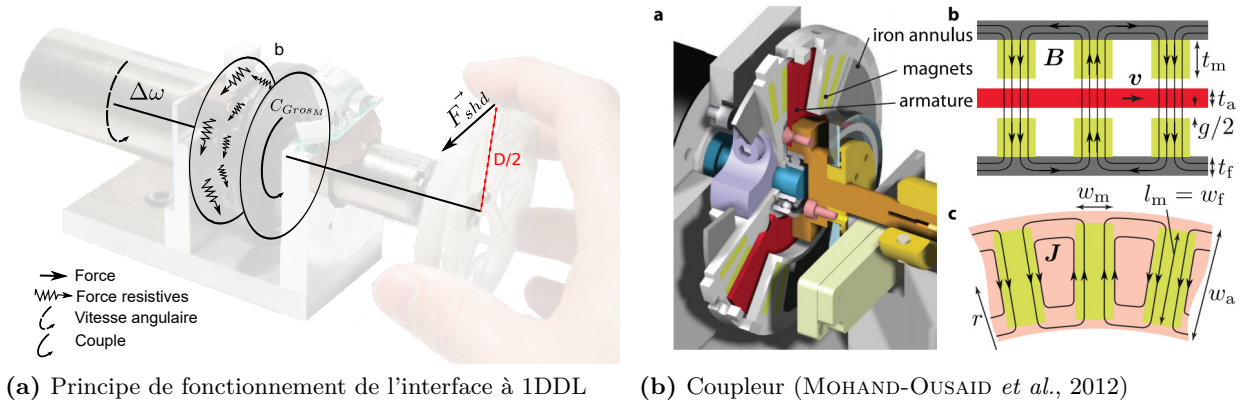
Figure 1.15: Détails de la transmission des efforts
