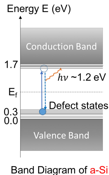
Figure 5: Diagramme des états électroniques dans le a-Si:H qui explique les expériences de photoluminescence.
