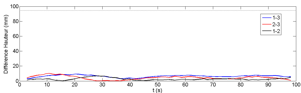
FIGURE B.4 – Différences de hauteur de houle sans courant
