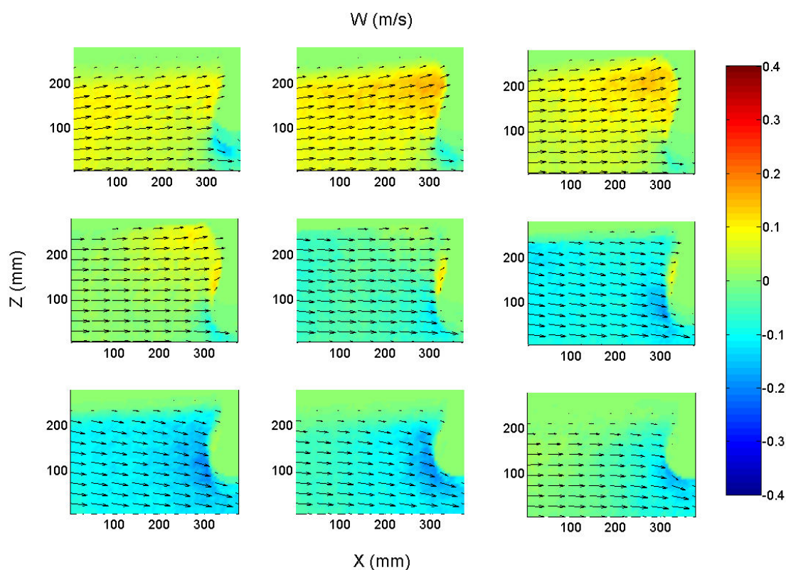
FIGURE 5.32 – Moyennes de phase sur toute la séquence de la configuration 4, dans le plan de symétrie de la maquette
