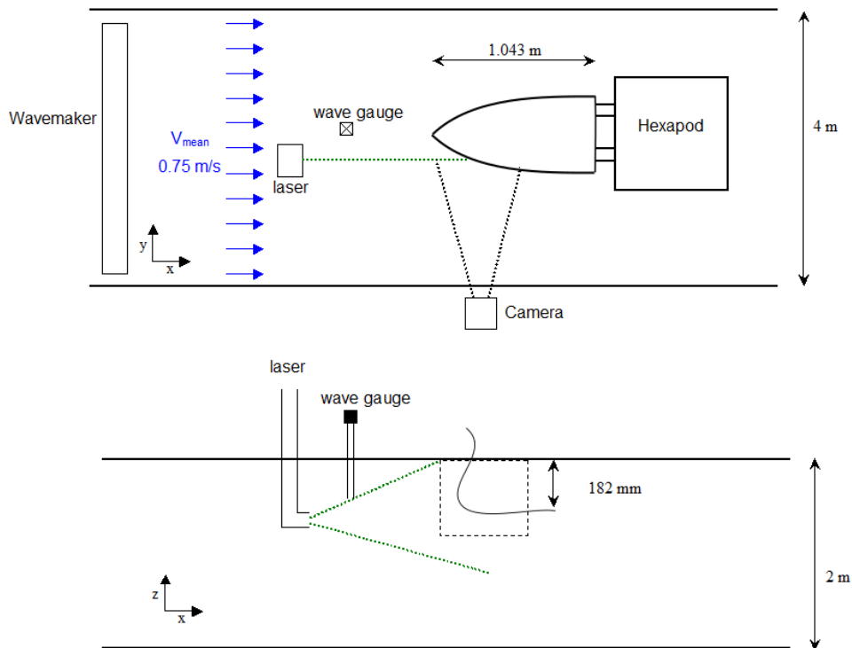
FIGURE 3.6 – Schémas du montage expérimental. [Haut] Vue du dessus. [Bas] Vue de profil.
