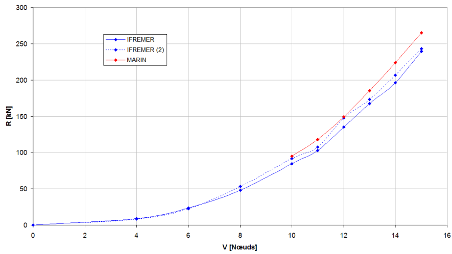
FIGURE A.3 – Comparaison des mesures de résistance à l’avancement du Pourquoi pas ? effectuées à MARIN et à l’Ifremer
