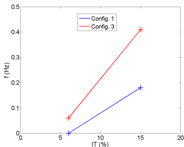
FIGURE 4.26 – Influence de l'intensité turbulente sur la fréquence d'apparition des nuages de bulles
