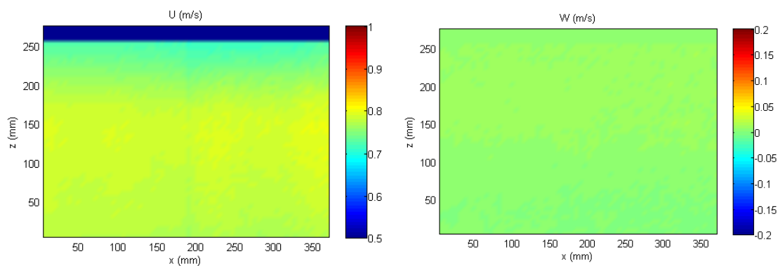
FIGURE 5.1 – Champs de vitesses moyennes sans générateur de houle. [Gauche] Vitesse longitudinale. [Droite] Vitesse verticale.
