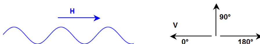
FIGURE 2.23 – Schéma de définition des angles de cap par rapport à la houle
