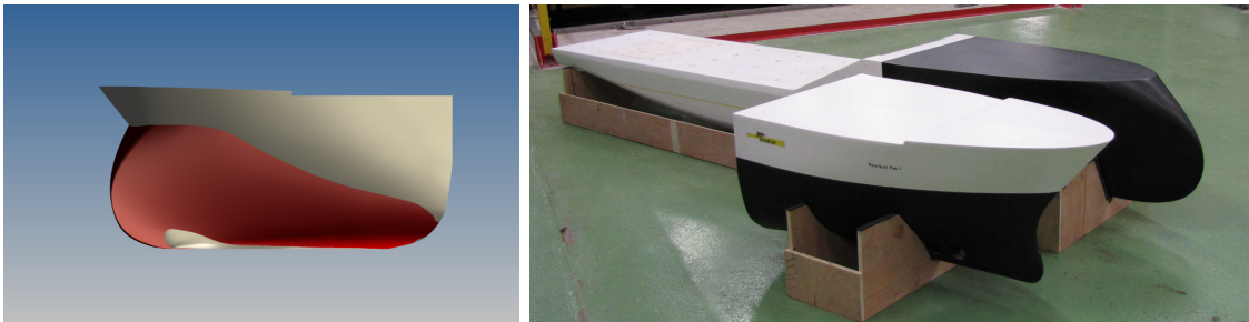
FIGURE 6.2 – Comparaison des formes du Pourquoi pas ? avec les formes du navire équivalent à étrave inversée
