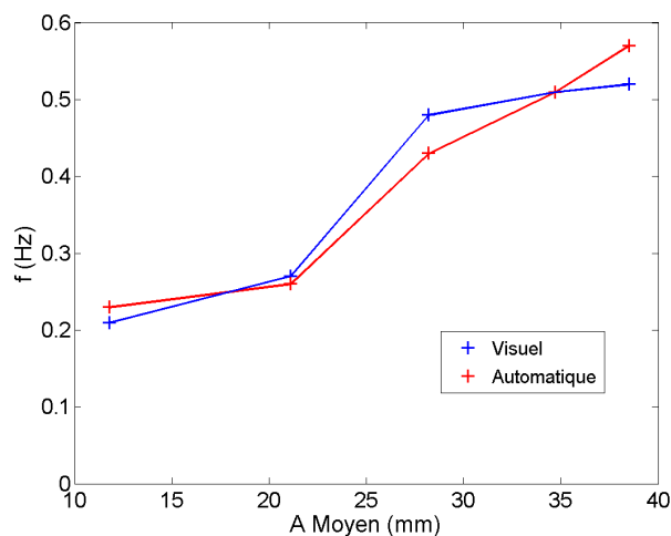
FIGURE 4.12 – Comparaison des fréquences d’apparition des nuages de bulles obtenues visuellement ou par détection automatique
