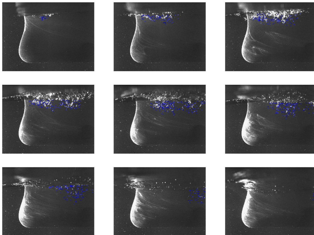
FIGURE 4.10 – Séquence d'un nuage de bulle par déferlement (configuration 2 avec courant et houle). Les aérations détéctées sont marquées en bleu.
