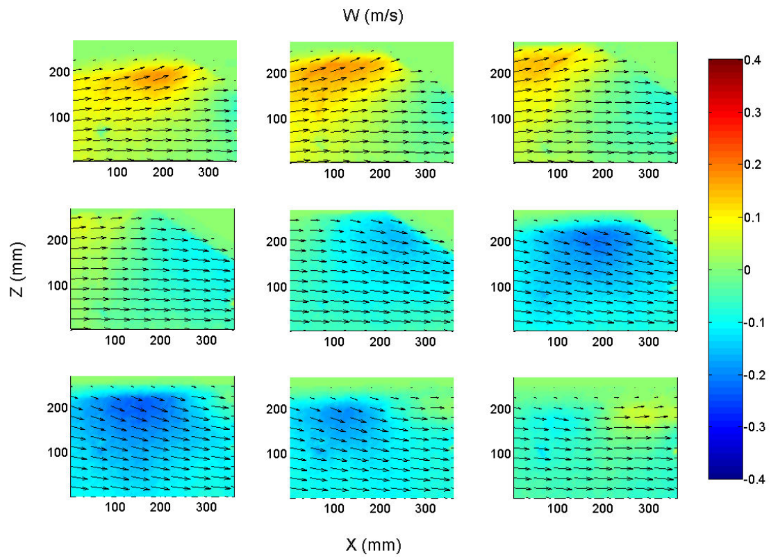
FIGURE 5.33 – Moyennes de phase sur toute la séquence de la configuration 4, dans le plan à y = 100 mm
