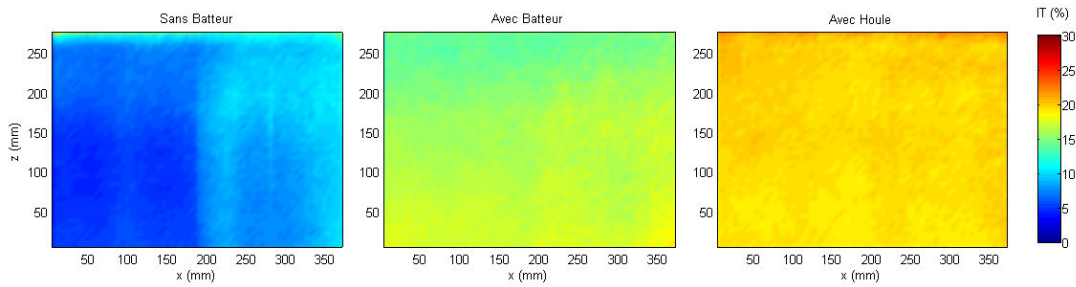
FIGURE 5.9 – Intensité turbulente pour les trois configurations. [Gauche] Générateur relevé. [Centre] Générateur immergé, sans houle. [Droite] Avec houle.
