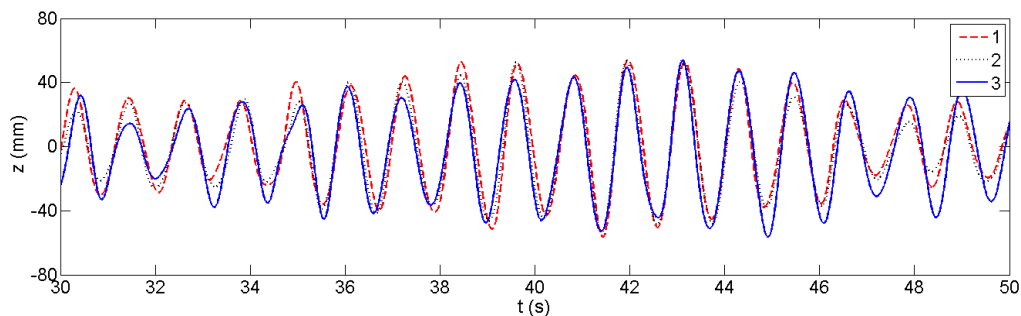
FIGURE B.5 – Superposition des signaux de houle avec courant
