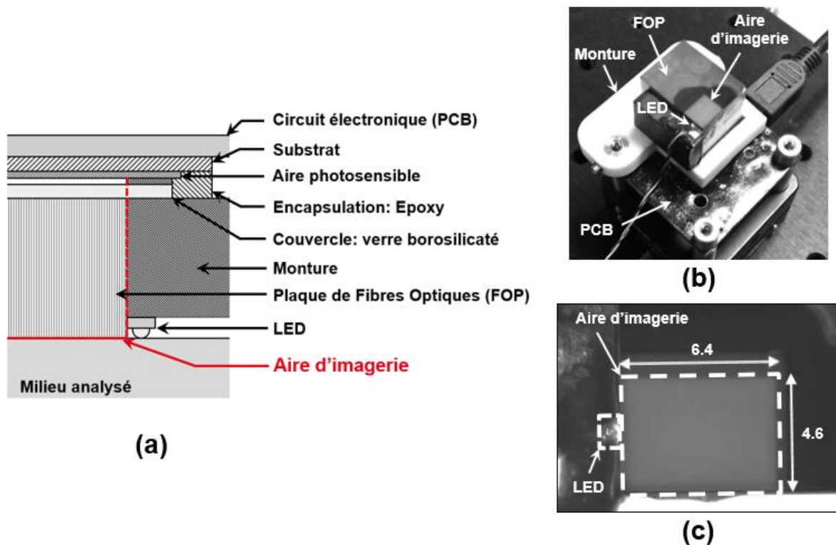
Fig. 2 (a) Structure schématique du système proposée pour l'imagerie de réflectance diffuse en contact. L'aire d'imagerie (ligne rouge) est déportée depuis l'aire photosensible du CMOS vers la surface du milieu analysé. (b) Photographie du prototype implémenté pour preuve de concept (c) Vue axiale du prototype. Les dimensions sont données en millimètres. L'aire d'imagerie délimitée par la ligne pointillée est vue à travers la plaque de fibres optiques (FOP).
