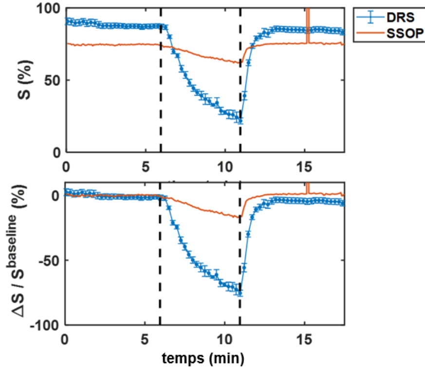
Fig. 11 Saturation tissulaire en oxygène ( StO_2 ) mesurée pendant l'expérience d'occlusion avec les systèmes srDRS et SSOP. Les barres d'erreur correspondent à l'écart-type entre les valeurs obtenues à partir de différentes mesures du fantôme de calibration.
