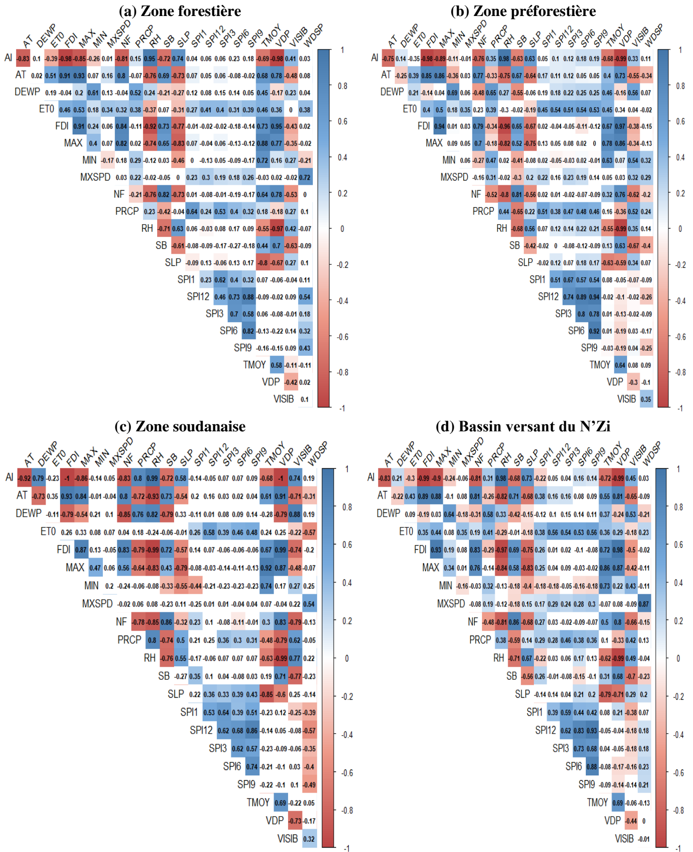
Figure 5-14 : Corrélogramme des variables pyrologiques et climatiques au niveau de la (a) zone forestière, (b) zone préforestière, (c) zone soudanaise et (d) l'ensemble du BVN
