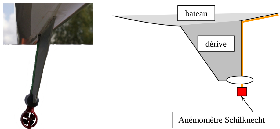
FIGURE 8.1 – Positionnement de l'anémomètre Schiltknecht sur la dérive du bateau d'aviron
