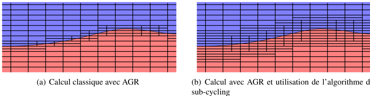
FIGURE 4.3 – Visualisation du nombre de couches de cellules raffinées autour de la surface libre dans (a) le cas classique et (b) le cas d'un calcul utilisant l'algorithme de sub-cycling.
