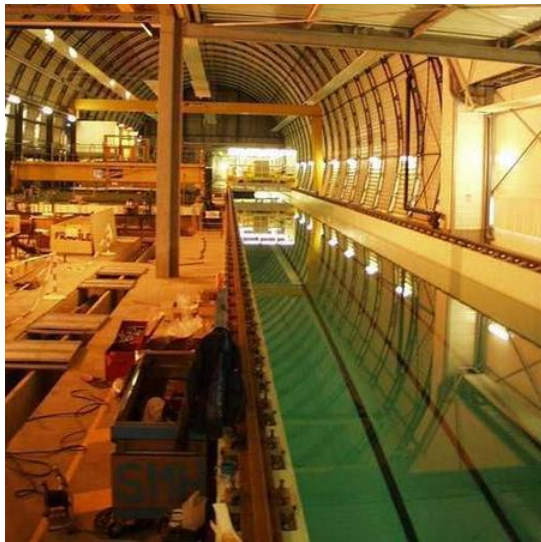
(a) bassin de traction
