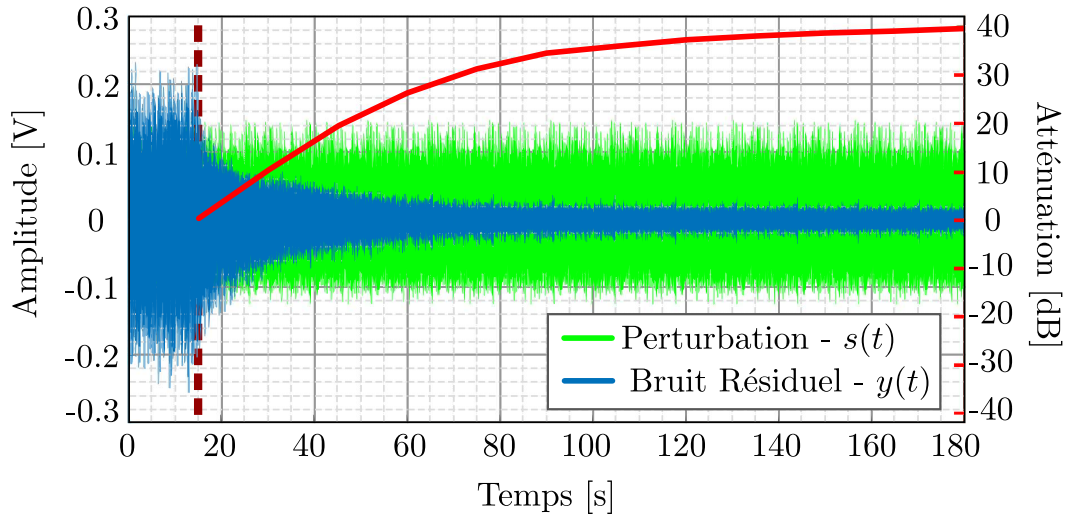
FIGURE 1.17. Performance du compensateur IIR. Le côté droit montre le niveau d'atténuation atteint à un moment donné.
