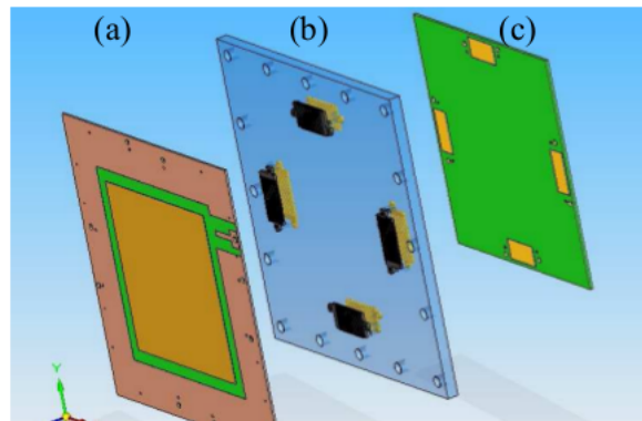
FIGURE 2.5 – Schéma de l'assemblage réalisé pour le détecteur \mu TPC entre le détecteur Micromegas et la carte électronique servant à la lecture de l'anode. Le PCB (a) supporte la Micromegas en son centre, la plaque (b) est un sandwich de PCB et de cuivre de 0,5 cm d'épaisseur garantissant la rigidité et assurant l'étanchéité, et le PCB (c) est la carte électronique [15].
