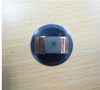
FIGURE 5.5 – Photographie de la cible de béryllium, après irradiation, utilisée sur l'installation AMANDE pour la mesure du spectre neutronique.
