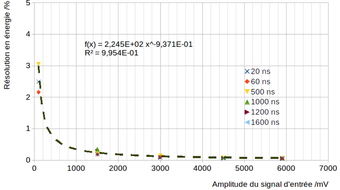
FIGURE 3.4 – Résolution en énergie de l'électronique de mesure du détecteur \mu TPC en fonction de l'amplitude du signal d'entrée pour différents temps de montée.
