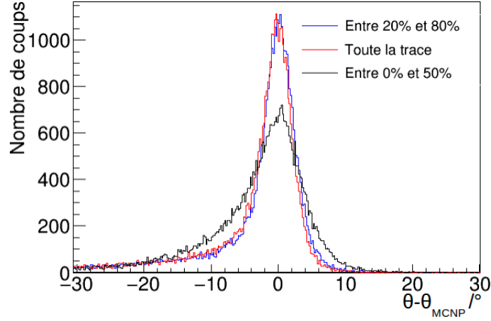
FIGURE 3.25 – Écart entre l'angle de diffusion reconstruit \theta , calculé à partir d'une analyse de la composante principale des barycentres de la trace, et l'angle de diffusion initial, fourni par MCNP, \theta_{MCNP} . La courbe rouge est le résultat d'une ACP sur toute la trace, la bleue entre 20% et 80% de la trace et la noire sur la première moitié de la trace.
