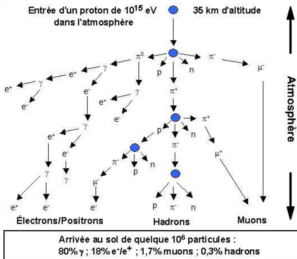
FIGURE 1.5 – Schéma de production des particules induites par le rayonnement cosmique [4].
