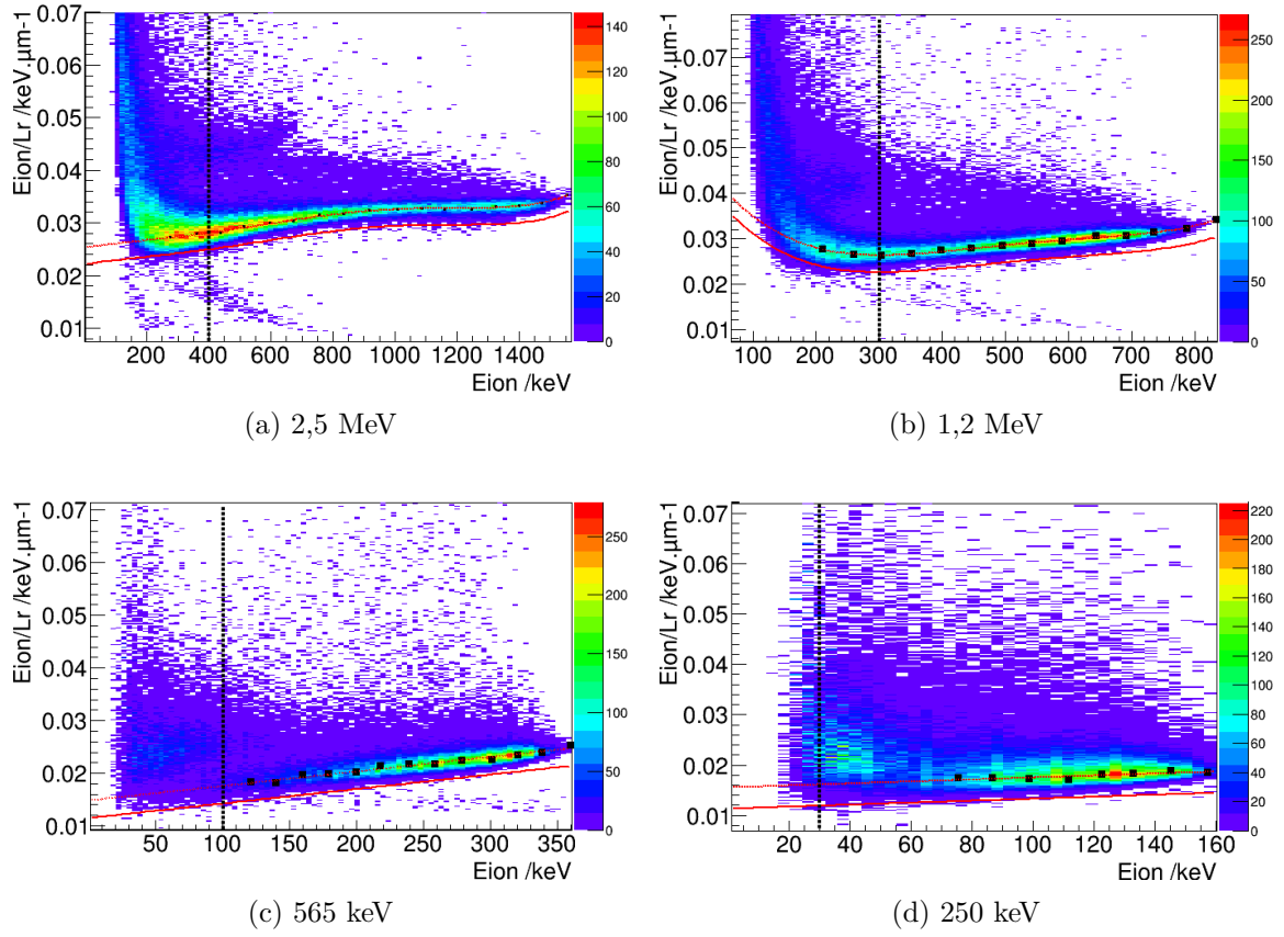
FIGURE 3.29 – Représentation des sélections d'événements effectuées sur le pouvoir d'arrêt moyen des noyaux de recul mesurés entre 250 keV et 2,5 MeV.
