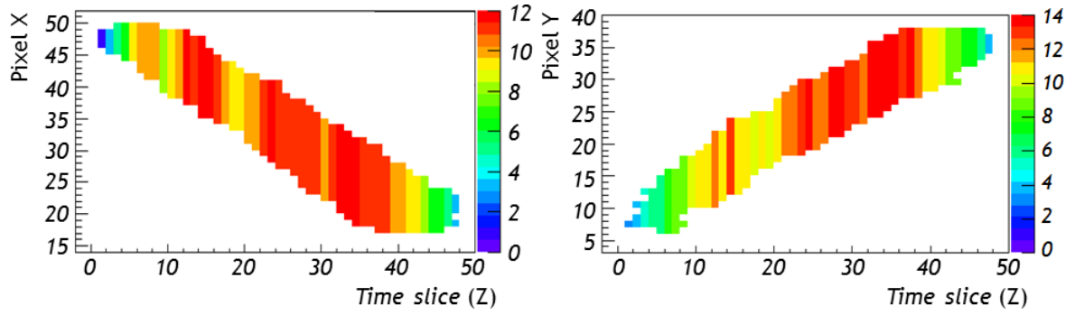
FIGURE 2.15 – Projections des pixels X déclenchés pour chaque time slice à gauche et des pixels Y pour chaque time slice à droite, d'un recul d'hélium-4 de 471 keV en ionisation mesuré avec le détecteur \mu TPC.
