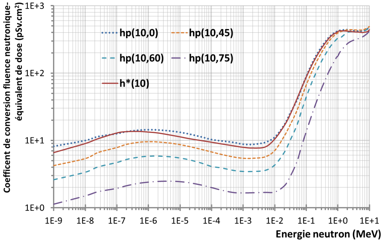
FIGURE 1.4 – Evolution des facteurs de conversion ambiant h^* et personnel h_p en fonction de l'énergie des neutrons, à une profondeur de 10 mm et pour différents angles d'incidence [3].
