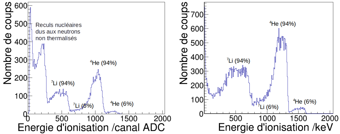
FIGURE 3.20 – Spectre en énergie déposée par ionisation dans le gaz ^4\text{He}+5\% \text{CO}_2 par les produits de la réaction de capture neutronique du ^{10}\text{B} , à gauche dans le cas expérimental et à droite dans le cas d'une simulation MCNP.
