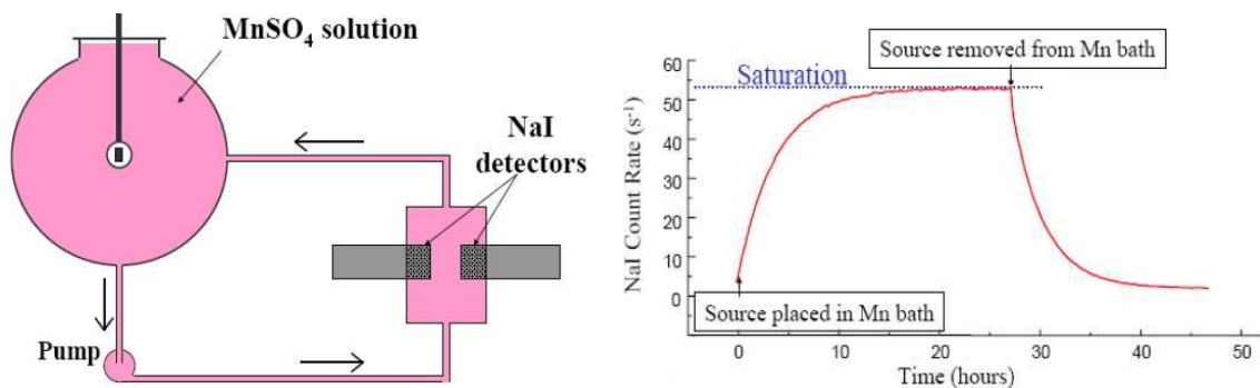
FIGURE 1.9 – Sur la figure de gauche est représenté le schéma de la chaîne de mesure du débit de dose d’une source nucléaire. Sur la figure de droite est représentée l’évolution du taux de comptage dans les détecteurs NaI en fonction du temps.
