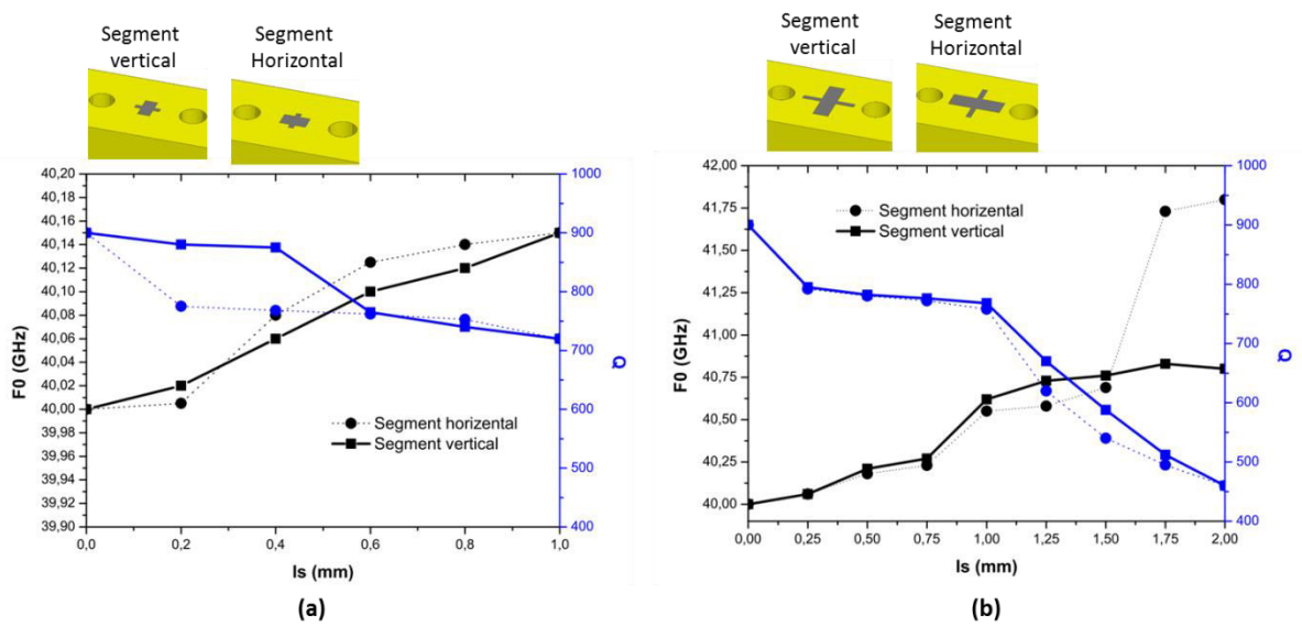
Figure 151 : Décalage fréquentiel et évolution du facteur de qualité en fonction de la largeur sur segment horizontal ou vertical d'une croix de côté égal à 1mm (a) et à 2 mm (b).
