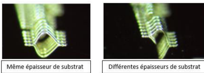
Figure III.94 : Photographies des câblages filaires type "bonding" utilisés à Thales Alenia Space.
