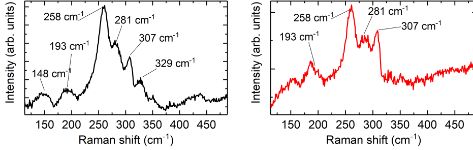
Figure B.22: Spectre Raman des flocons de franckite d'environ 90 nm épais avec des modes caractéristiques marqués en polarisation (a) parallèle et (b) perpendiculaire en moyennes sur toute la gamme des directions d'excitation.
