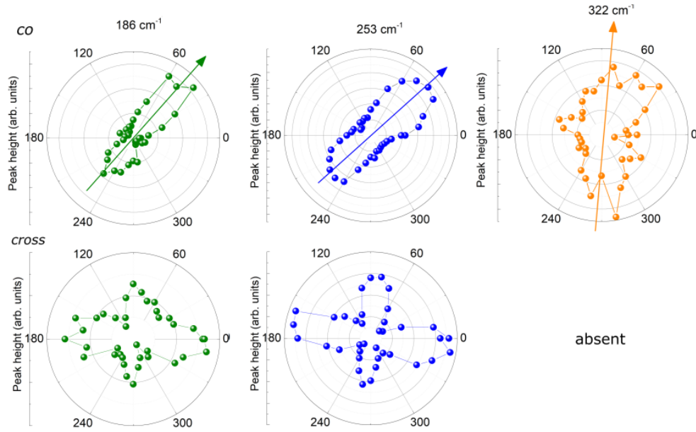
Figure B.24: Diagrammes polaires montrant l'intensité du mode 186 cm -1 (vert), 253 cm -1 (bleu foncé) et 322 cm -1 (orange) en fonction de l'angle d'excitation en polarisation parallèle (haut) et en polarisation croisée (bas). Le mode 322 cm -1 n'a pas été observé en polarisation croisée. Les flèches marquent les directions approximatives de l'intensité maximale.
