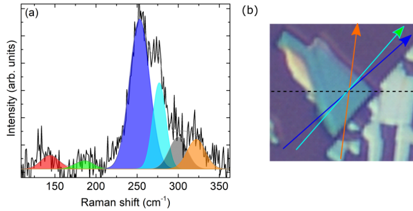
Figure B.25: (a) Exemple d'ajustement d'un spectre pour un angle d'excitation de 0° avec des pics lorentziens; (b) Micrographie optique du flocon. La direction 0° est marquée avec la ligne pointillée et les directions d'intensité maximale dérivées des diagrammes polaires pour les modes 186 cm -1 (vert), 253 cm -1 (bleu foncé) et 322 cm -1 (orange) sont indiquées par les flèches.
