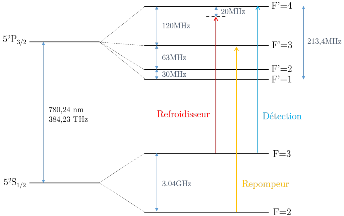
FIGURE 2.4 – Schéma des niveaux du \text{Rb}^{85} impliqués lors du refroidissement et de la détection des atomes.
