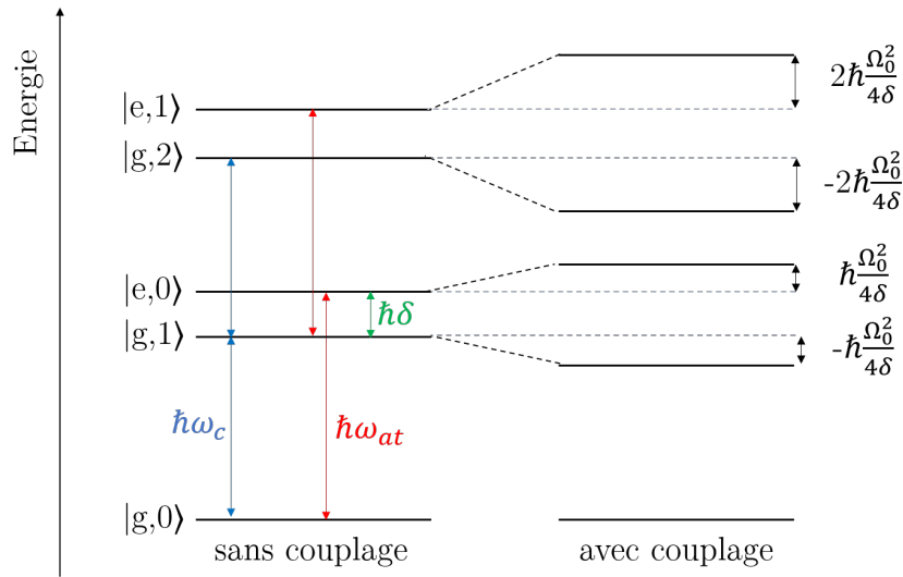
FIGURE 1.22 – Diagramme énergétique des deux premiers doublets et du niveau fondamental pour le système atome-champ dans le régime dispersif
