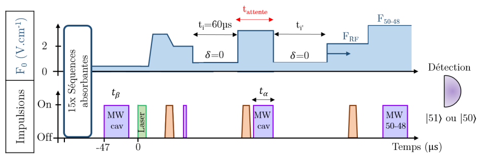
FIGURE 3.25 – Séquence expérimentale utilisée pour sonder la décohérence de l'état chat de Schrödinger déplacé, généré comme précédemment à partir de l'interaction d'un champ cohérent et d'un atome excité. Les deux injections micro-ondes correspondent à \beta = 3.63 et \alpha = -0.60 . Un temps d'attente variable à haut désaccord t_{attente} est choisi, puis les oscillations de Rabi entre le chat déplacé et l'atome réinitialisé dans l'état |e\rangle sont enregistrées autour de t'_i \approx t_R/2 .
