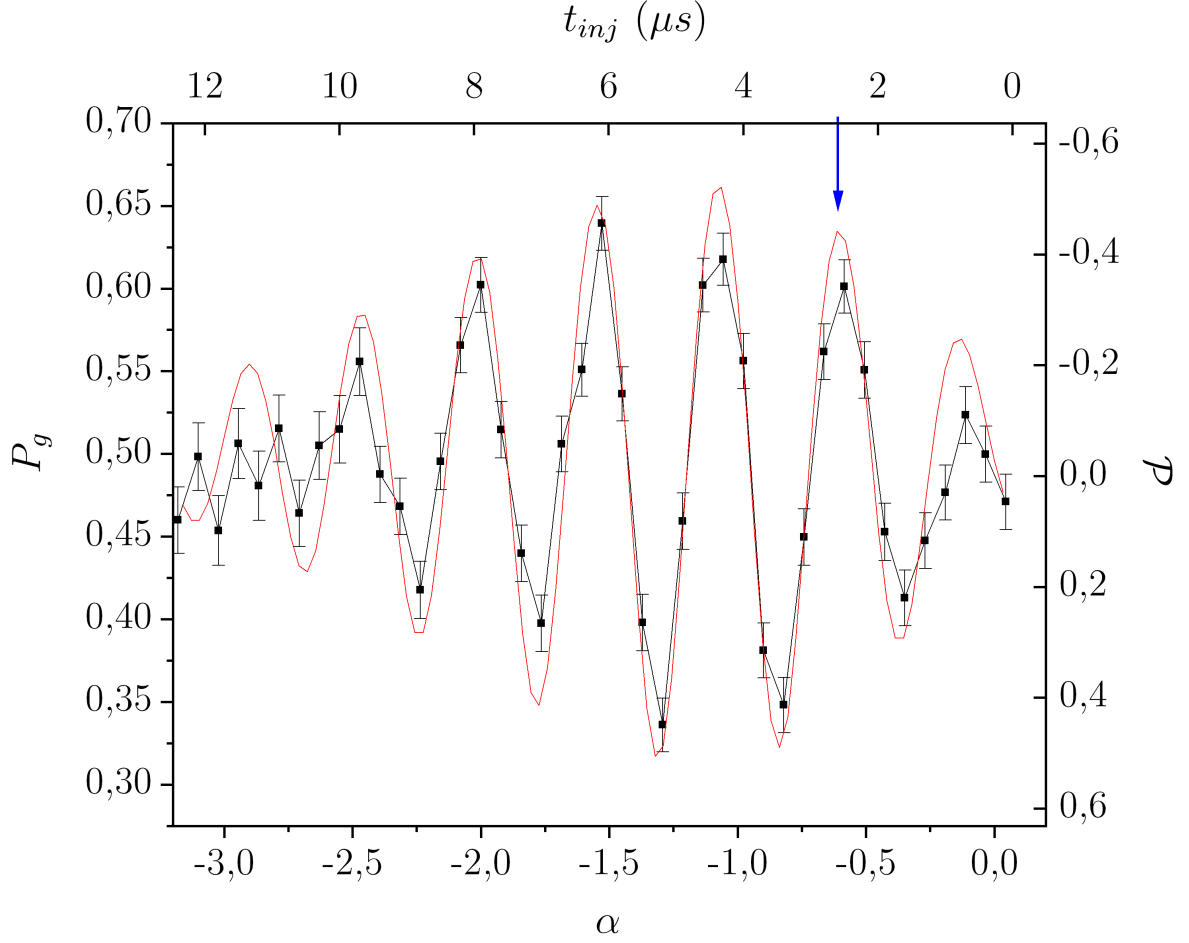
FIGURE 3.18 – Oscillations de parité dans un état chat de Schrödinger. Points noirs reliés par une ligne fine : P_g(t_1, \alpha) mesurée expérimentalement pour t'_i = t_1 = 68.5 \mu s en fonction du déplacement d'amplitude \alpha . La ligne rouge est le résultat d'une simulation numérique prenant en compte les paramètres expérimentaux. La flèche bleue marque \alpha = -0.596 , extremum local de la parité, que nous utiliserons pour mesurer les oscillations de Rabi temporelles dans un état chat.
