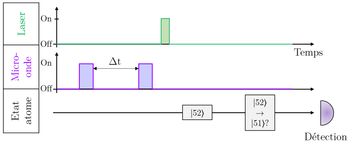
FIGURE 2.23 – Séquence expérimentale mise en oeuvre pour les courbes dites « de retour à 0 ». Deux injections micro-ondes d'espacement variable \Delta t sont faites à un faible désaccord. La probabilité de détecter l'atome dans l'état |51\rangle est ensuite mesurée et témoigne de la présence ou non d'un champ résiduel dans la cavité.
