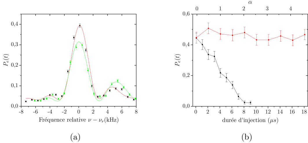
FIGURE 2.29 – (a) Spectroscopie du vide générée après le passage de 15 séquences absorbantes successives. L’atome sonde est préparé 2.7 ms après le passage des séquences absorbantes. La probabilité P_e(t) est tracée en fonction de la fréquence de l’injection relative par rapport à la fréquence \nu_r = \nu_{|h,0\rangle \rightarrow |e,0\rangle} = 48.179\,334\,7 GHz. La courbe rouge est un ajustement fait par une somme de sinus cardinaux. Les points verts et l’ajustement correspondant sont un rappel de la spectroscopie du champ thermique. (b) Amplitude du pic de la transition |h, 0\rangle \rightarrow |e, 0\rangle en fonction de la durée d’injection pour tester l’efficacité des séquences absorbantes. En noir : lorsque l’injection a lieu entre les séquences absorbantes et l’atome principal. En rouge : lorsque l’injection a lieu avant les séquences absorbantes.
