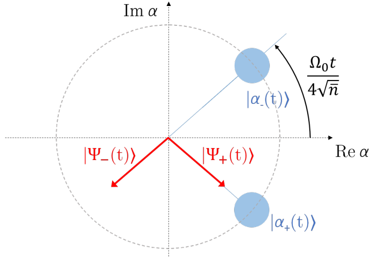
FIGURE 1.18 – Représentation dans le plan de Fresnel de l'état du système atome-champ à partir de |e\rangle \otimes |\alpha\rangle : création d'une superposition de champs cohérents. Le plan équatorial de la sphère de Bloch est superposé au plan de l'atome pour pouvoir représenter les états atomiques : l'état |+\rangle est orienté selon \text{Re}(\alpha) et l'état |-\rangle selon -\text{Re}(\alpha) .
