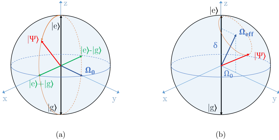
FIGURE 1.14 – Effet d’une impulsion micro-onde classique sur le vecteur de Bloch d’un atome initialement préparé dans l’état |e\rangle (a) Dans le cas résonnant c’est une rotation autour vecteur \Omega_0 aligné ici avec l’axe \mathbf{n}_y à une pulsation \Omega_0 (b) Dans le cas dispersif c’est une rotation autour vecteur \Omega_{\text{eff}} à une pulsation \sqrt{\Omega_0^2 + \delta^2} .
