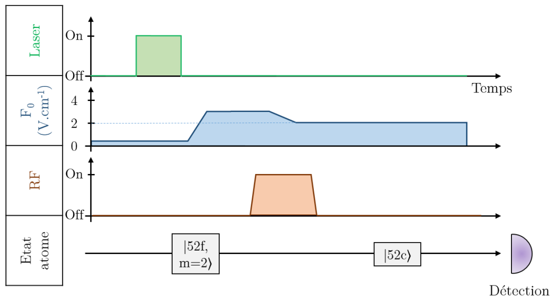
FIGURE 2.18 – Séquence expérimentale associée à la circularisation par passage adiabatique. L'allumage du laser, le profil du champ généré dans la cavité et l'allumage de la Radiofréquence sont représentés en fonction du temps.
