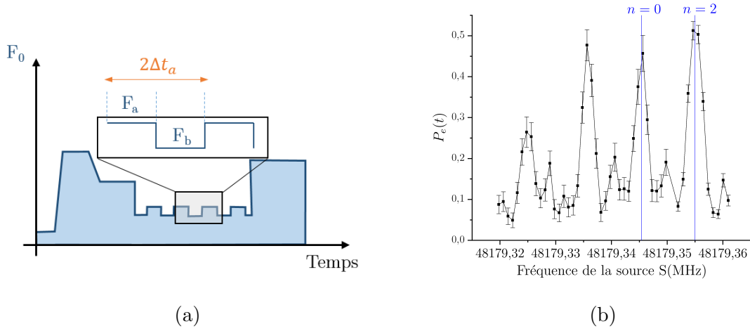
FIGURE 4.19 – (a) Profil en champ électrique utilisé pour générer des bandes latérales dans le spectre de la transition |h\rangle \rightarrow |e\rangle . La modulation est caractérisée par un motif en créneaux entre deux valeurs de champ F_a et F_b périodique de période 2\Delta t_a . (b) Spectroscopie de la transition |h\rangle \rightarrow |e\rangle lorsque la cavité est préparée dans l'état vide, en présence de la modulation précédente. On trace la probabilité P_e en fonction de la fréquence de la source. La modulation fait apparaître plusieurs bandes latérales, donc une coïncide exactement avec la position du pic associé à la transition \mathcal{T}_{-,2} (trait vertical bleu).
