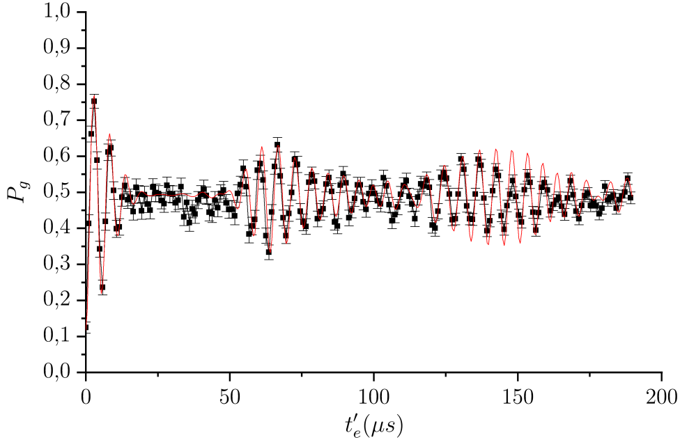
FIGURE 3.20 – Oscillations de Rabi dans un état chat de Schrödinger. Les points noirs reliés par un trait fin sont la probabilité P_g mesurée expérimentalement en fonction du temps effectif t'_e . La courbe rouge est le résultat d’une simulation numérique intégrant les caractéristiques de l’expérience et renormalisée par la loi homographique définie par les paramètres d’ajustement (3.12).
