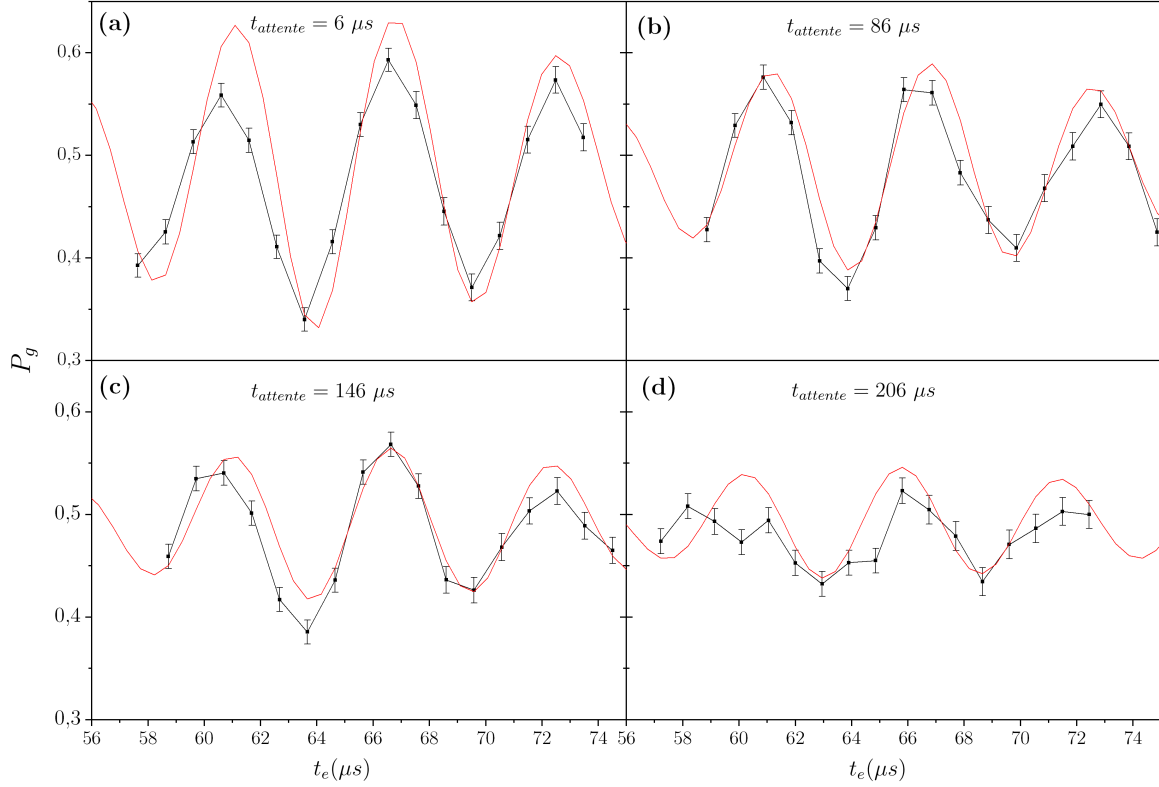
FIGURE 3.26 – Décohérence d'un état chat de Schrödinger : oscillations de Rabi P_g(t'_e) mesurées expérimentalement autour du temps de demi-résurgence t_R/2 dans un état chat de Schrödinger déplacé pour différents temps d'attente t_{attente} durant lequel la cohérence de la superposition décroît exponentiellement. Les courbes rouges sont le résultat de simulations numériques dans les conditions de l'expérience.
