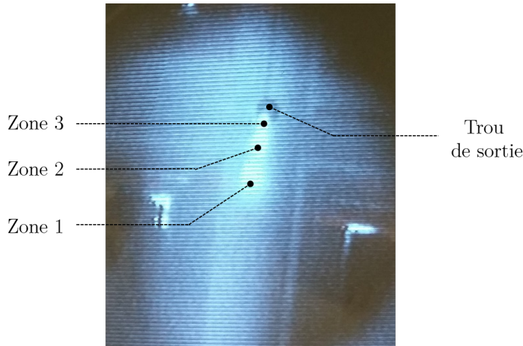
FIGURE 2.8 – Les 3 zones du 2D-MOT observées par en-dessous à l'aide d'une finger caméra une fois la procédure de réglages effectuée.
