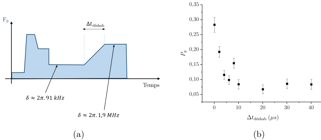
FIGURE 4.12 – (a) Profil du champ électrique de la séquence expérimentale utilisée pour déshabiller l'état du système {atome+champ} à la fin de la spectroscopie conditionnelle. Le désaccord passe continûment d'un régime de désaccord intermédiaire \delta/2\pi = 91 kHz dans lequel a lieu la spectroscopie longue durée à un régime fortement désaccordé \delta_d/2\pi = 1.9 MHz en un temps de déshabillage noté \Delta t_{\text{deshab}} . (b) Probabilité P_g de détecter l'atome dans l'état |g\rangle en fonction du temps de déshabillage \Delta t_{\text{deshab}} après préparation de l'état conditionnel associé à n = 5 photons.
