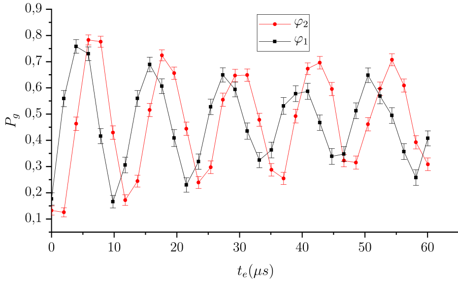
FIGURE 4.15 – Oscillations de Rabi P_g(t_e) dans l'état obtenu à l'issue d'une spectroscopie conditionnelle sur n = 2 puis d'une rotation du dipôle atomique d'une phase \varphi . La courbe noire correspond à un déphasage \varphi_1 = 2.38 et la courbe rouge à un déphasage \varphi_2 = 4.93 .
