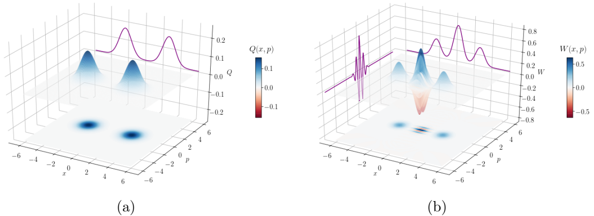
FIGURE 1.7 – (a) Représentation schématique d'un état chat de Schrödinger |\Psi_{pair}\rangle = (|2.5\rangle + |-2.5\rangle)/\mathcal{N}_{\pm} dans le plan complexe. (b) Fonction de Wigner du même état.
