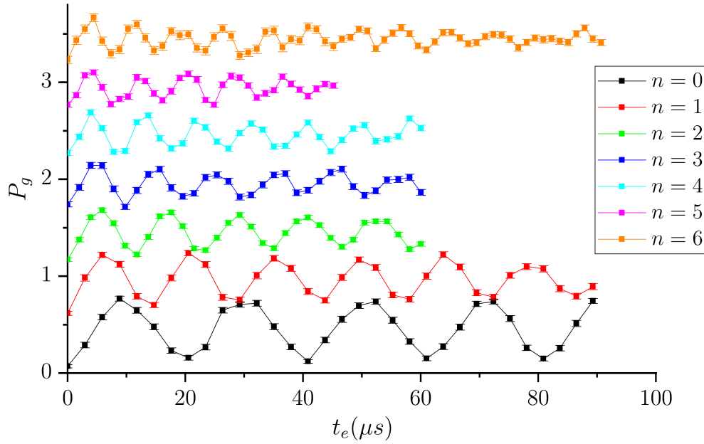
FIGURE 4.8 – Oscillations de Rabi P_g(t_e) dans les états de Fock |n\rangle obtenus par post-sélection à l'issue d'une spectroscopie conditionnelle sélective en n . Les 7 courbes sont décalées verticalement pour plus de lisibilité mais leur échelle est identique. L'axe des abscisses est le temps effectif calculé à partir du temps d'interaction t_i expérimental.
