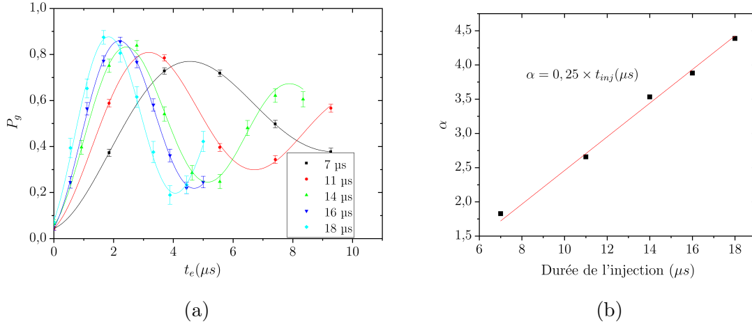
FIGURE 3.8 – Calibration de l’injection micro-onde dans le mode de la cavité : (a) Points discrets : oscillations de Rabi P_g en fonction du temps effectif t_e pour différentes durées d’injections dans la cavité t_{inj} et ajustement par une sinusoïde amortie (courbe continue) nous donnant pour chaque courbe un paramètre \alpha . (b) \alpha correspondant en fonction de t_{inj} . Un ajustement linéaire nous donne la loi de proportionnalité \alpha(t_{inj}) = k \cdot t_{inj} .
