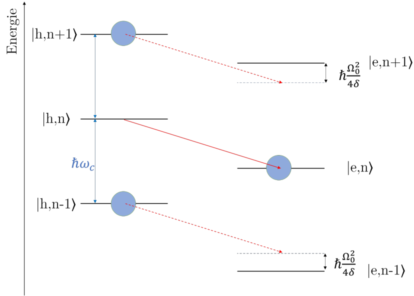
FIGURE 1.23 – Diagramme énergétique détaillant le principe de l'expérience menée en régime dispersif entre les niveaux non couplés |h, n\rangle et les niveaux couplés |e, n\rangle . L'état du système est représenté par un disque bleu. Les niveaux |h, n\rangle sont espacés régulièrement car ils sont non couplés. En revanche les niveaux |e, n\rangle sont modifiés et ce proportionnellement à n . En sondant la transition à une fréquence adaptée (en rouge) on peut adresser sélectivement la transition correspondant à un nombre donné de photons.
