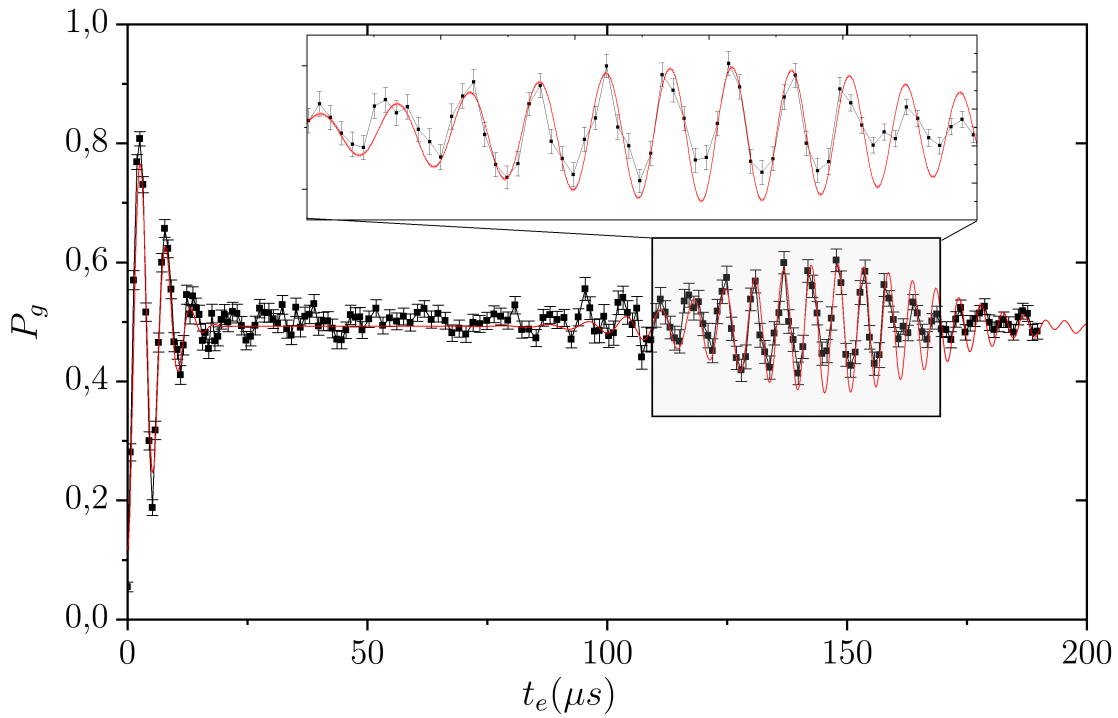
FIGURE 3.9 – Oscillations de Rabi dans un champ cohérent |\beta\rangle avec \beta^2 = 13.2 \pm 0.1 . Les points noirs reliés par un trait fin sont la probabilité P_g mesurée expérimentalement en fonction du temps effectif t_e . La courbe rouge est le résultat d’une simulation numérique intégrant les caractéristiques de l’expérience et renormalisée par une loi homographique. L’insert présente un zoom sur le résurgence des oscillations.
