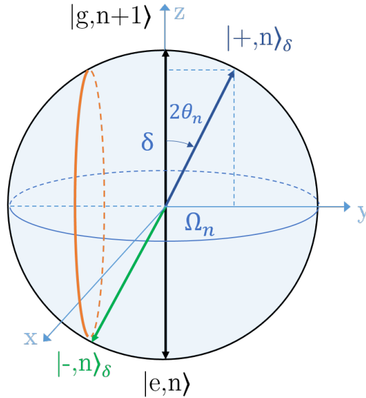
FIGURE 4.13 – Sphère de Bloch associée au sous-espace \{|e, n\rangle, |g, n+1\rangle\} . L'ellipse orange représente la trajectoire du vecteur décrivant l'état joint de l'atome et du champ durant les oscillations de Rabi P_g(t_e) faites à résonance. L'état initial est l'état obtenu à l'issue d'une spectroscopie conditionnelle sur n représenté ici par le vecteur vert |- , n\rangle_\delta .
