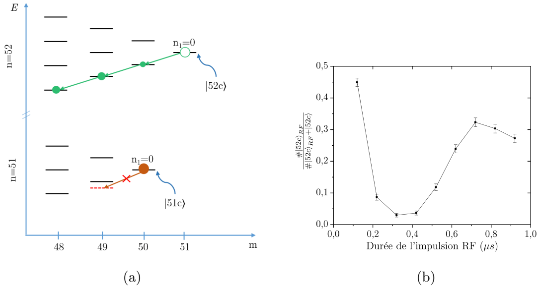
FIGURE 2.32 – (a) Transitions radiofréquence mises en jeu lors du transfert des atomes présents dans l'état |52c\rangle des états de plus faible nombre quantique m . Les atomes présents dans l'état |51c\rangle ne sont pas sensibles à cette radiofréquence car elle est hors résonance pour cette multiplicité. (b) Evolution du transfert entre l'état |52c\rangle en présence de l'impulsion radiofréquence par rapport à l'état |52c\rangle en son absence. Le nombre de |52c\rangle détectés est minimal pour une durée d'impulsion de 0.32 \mu\text{s} . La remontée du transfert après cette durée s'explique par le fait que nous induisons une oscillation de Rabi au sein des états |n = 52, m, n_1 = 0\rangle .
