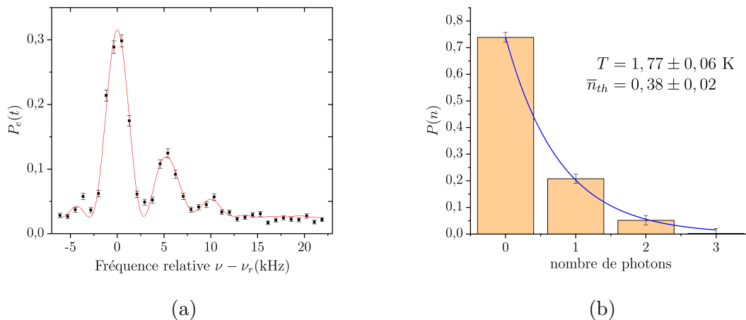
FIGURE 2.27 – (a) Spectroscopie du champ thermique réalisée en sondant les transitions |h, n\rangle \rightarrow |e, n\rangle dans un régime désaccordé. La probabilité P_e(t) est tracée en fonction de la fréquence de l'injection relative par rapport à la fréquence \nu_r = \nu_{|h,0\rangle \rightarrow |e,0\rangle} = 48.179\,334\,7 GHz. La courbe rouge est un ajustement fait par une somme de sinus cardinaux. (b) Amplitude relative des quatre pics de l'ajustement précédent nous donnant accès aux P(n) . Un ajustement (en bleu) est réalisé pour obtenir les paramètres de l'expérience que sont le nombre de photons thermiques et la température de la cavité.
