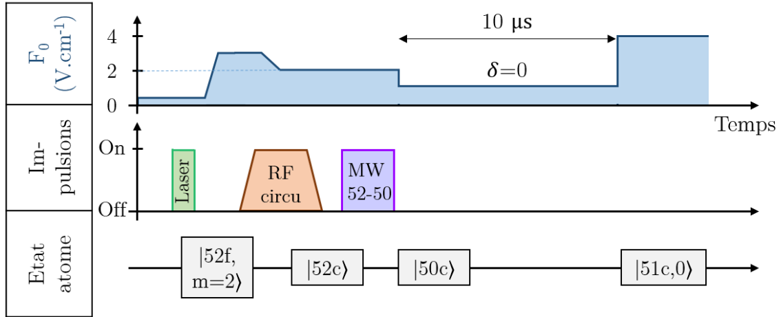
FIGURE 2.28 – Séquence expérimentale associée à une séquence absorbante utilisée pour réinitialiser le champ de la cavité.
