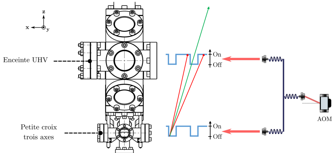
FIGURE 2.26 – Principe du système stroboscopique utilisé pour affiner la distribution en vitesses. Deux faisceaux laser espacés de 14 cm pulsés grâce à la commande d'un AOM dévient les atomes sauf la classe de vitesse souhaitée.
