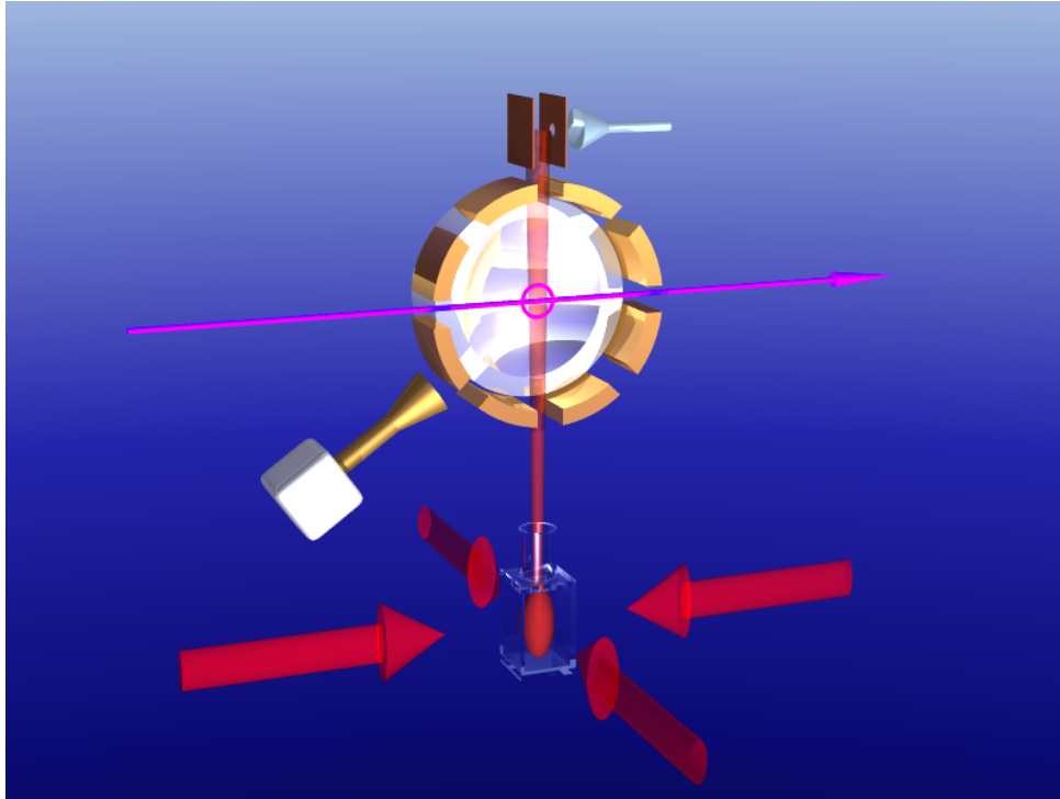
FIGURE 0.4 – Nouveau dispositif expérimental mis en place puis utilisé durant ma thèse. Une fontaine atomique reposant sur un piège magnéto-optique à deux dimension (en bas, en rouge) émet un jet d’atomes lents en direction de la cavité supraconductrice. Les atomes sont excités dans un niveau de Rydberg circulaire au sein de la cavité par des excitations laser (en violet) et un jeu d’électrodes (en doré) générant un champ radiofréquence. Les atomes sont ensuite détectés en sortie de la cavité.
