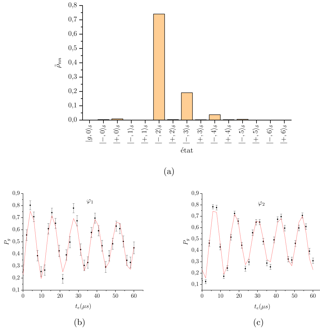
FIGURE 4.17 – (a) Éléments diagonaux de la matrice densité de l'état du système reconstruit par maximum de vraisemblance. (b) Comparaison des oscillations de Rabi expérimentales obtenues pour \varphi_1 (points noirs) et des oscillations de Rabi calculées pour l'état \rho_{exp} reconstruit (ligne rouge). (c) Comparaison des oscillations de Rabi expérimentales obtenues pour \varphi_2 (points noirs) et des oscillations de Rabi calculées pour l'état \rho_{exp} reconstruit (ligne rouge).
