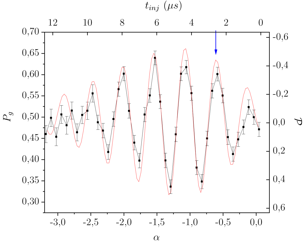
FIGURE 3.18 – Oscillations de parité dans un état chat de Schrödinger. Points noirs reliés par une ligne fine : P_g(t_1, \alpha) mesurée expérimentalement pour t'_i = t_1 = 68.5 \mu\text{s} en fonction du déplacement d'amplitude \alpha . La ligne rouge est le résultat d'une simulation numérique prenant en compte les paramètres expérimentaux. La flèche bleue marque \alpha = -0.596 , extremum local de la parité, que nous utiliserons pour mesurer les oscillations de Rabi temporelles dans un état chat.
