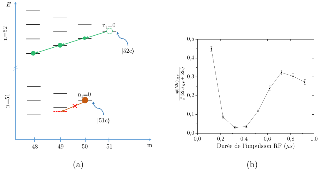
FIGURE 2.32 – (a) Transitions radiofréquence mises en jeu lors du transfert des atomes présents dans l'état |52c\rangle des états de plus faible nombre quantique m . Les atomes présents dans l'état |51c\rangle ne sont pas sensibles à cette radiofréquence car elle est hors résonance pour cette multiplicité. (b) Evolution du transfert entre l'état |52c\rangle en présence de l'impulsion radiofréquence par rapport à l'état |52c\rangle en son absence. Le nombre de |52c\rangle détectés est minimal pour une durée d'impulsion de 0.32\ \mu\text{s} . La remontée du transfert après cette durée s'explique par le fait que nous induisons une oscillation de Rabi au sein des états |n = 52, m, n_1 = 0\rangle .
