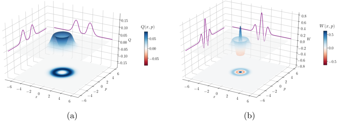
FIGURE 1.5 – (a) Fonction de Husimi-Q d'un état de Fock |n\rangle avec n = 2 . (b) Fonction de Wigner du même état.
