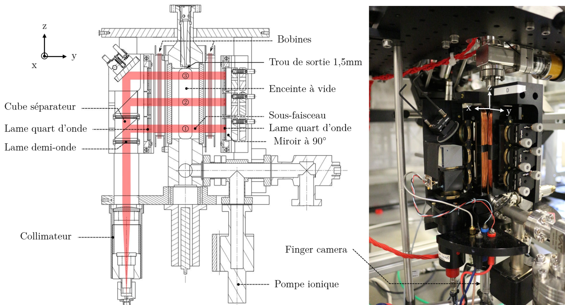
FIGURE 2.3 – (à gauche) Coupe selon le plan (yOz) du piège magnéto-optique à 2 dimensions utilisé dans l'expérience, formé de 3 zones successives. Les faisceaux laser sont représentés en rouge. (à droite) Photographie de la zone correspondante
