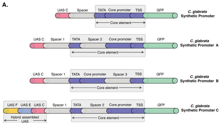
Figure 9. Amélioration du promoteur synthétique de C. glabrata . Le promoteur synthétique original de C. glabrata a été modifié pour permettre la synthèse d'une protéine fonctionnelle. Promoteur A : une séquence riche en A de 30 pb (Spacer 2) a été insérée en amont du promoteur du coeur promoteur pour l'éloigner de la boîte TATA. Promoteur B : une petite séquence de 6 pb (espaceur 3) a été insérée en amont du TSS. Promoteur C : sur la base du promoteur A, les éléments UAS F et UAS E ont été combinées avec l'élément UAS C.
