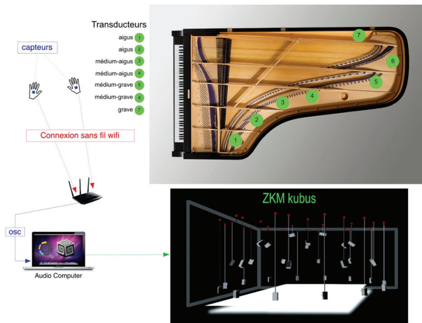
Fig. 65. Schéma technique et disposition des transducteurs dans la table d'harmonie du piano.
