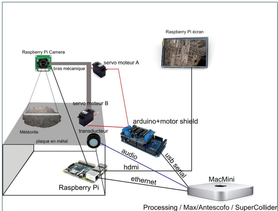
Fig. 46. Schéma de connexion entre les différents dispositifs de l'installation. L'ordinateur (Mac Mini) envoie les coordonnées au microcontrôleur Arduino pour déplacer le bras mécanique. L'image capturée est envoyée vers le Raspberry Pi qui la transfère à l'écran et au MacMini.
