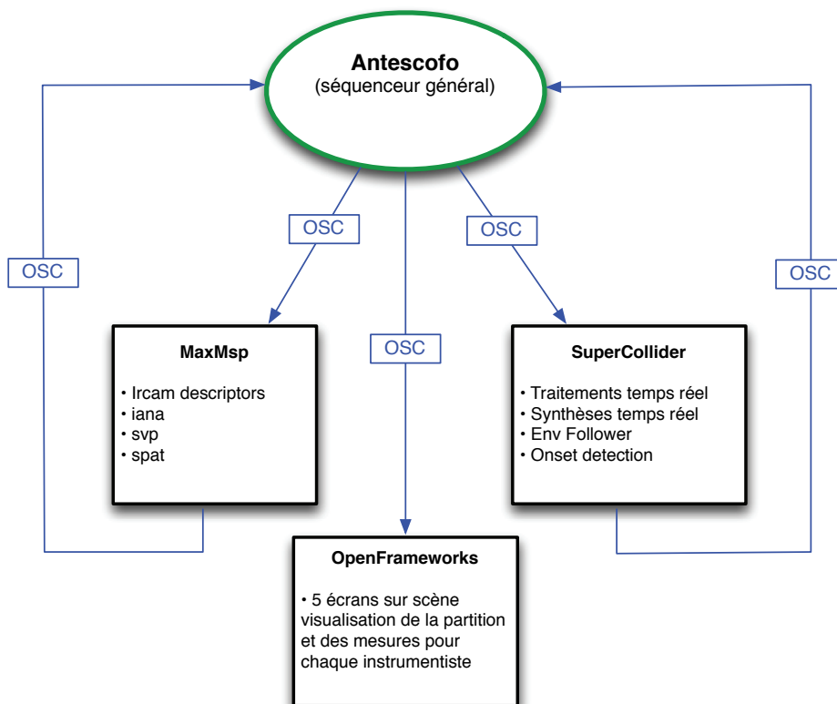
Fig. 36. Schéma de l'architecture de base du système utilisé : Antescofo employé comme « méta séquenceur » pour organiser tous les événements dans le temps en synchronisation avec la partition écrite par le protocole de communication OpenSoundControl.
