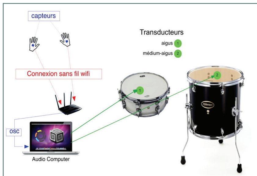
Fig. 67. Schéma technique et disposition des transducteurs sur les peaux des instruments.
