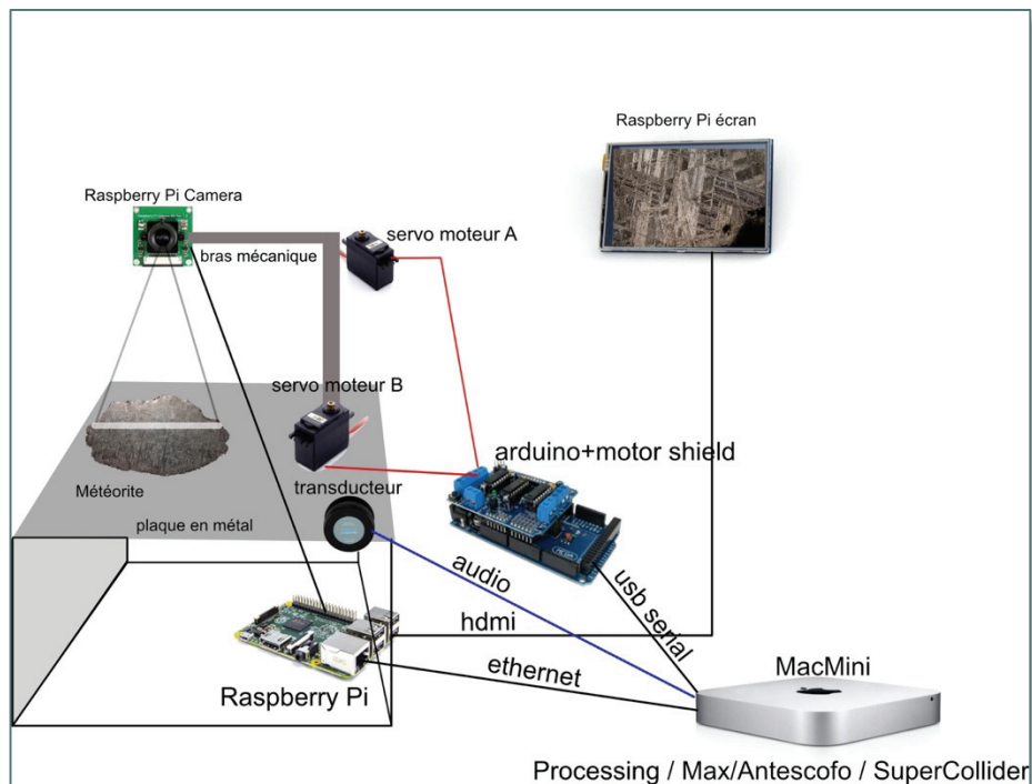
Fig. 46. Schéma de connexion entre les différents dispositifs de l'installation. L'ordinateur (Mac Mini) envoie les coordonnées au microcontrôleur Arduino pour déplacer le bras mécanique. L'image capturée est envoyée vers le Raspberry Pi qui la transfère à l'écran et au MacMini.
