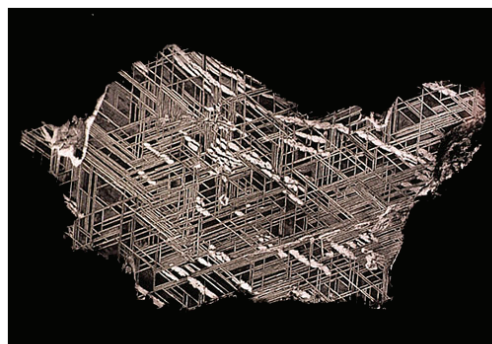
Widmanstätten Pattern
