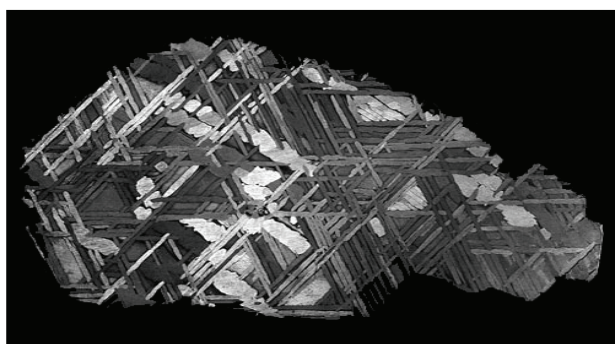
Widmanstätten Pattern
