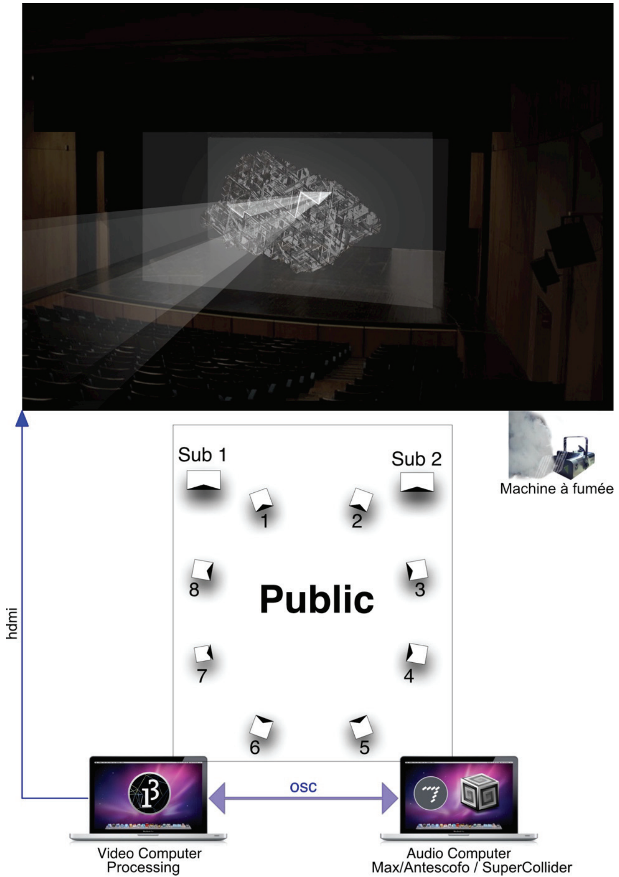
Fig. 50. Schéma de la version concert de l'œuvre audiovisuelle Octaédrite.
