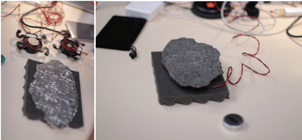
Fig. 48. Positionnement du transducteur au-dessous de la météorite : cette disposition n'a pas été retenue car la météorite étant trop petite et rigide, elle ne résonnait pas suffisamment. Le transducteur a finalement été posé sur une plaque en métal plus grande et résonante.
