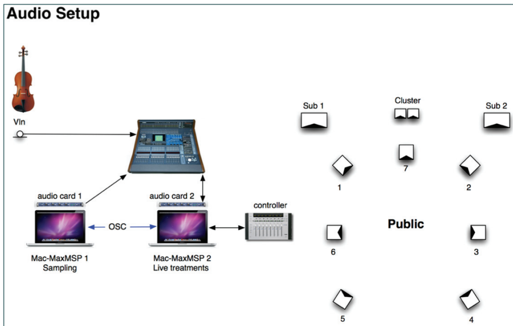
Fig. 28. L'ordinateur Mac-1 avec le suivi de partition Antescofo, déclenche des fichiers audio multicanaux et contrôle l'ordinateur Mac-2 avec les traitements en temps réel.
