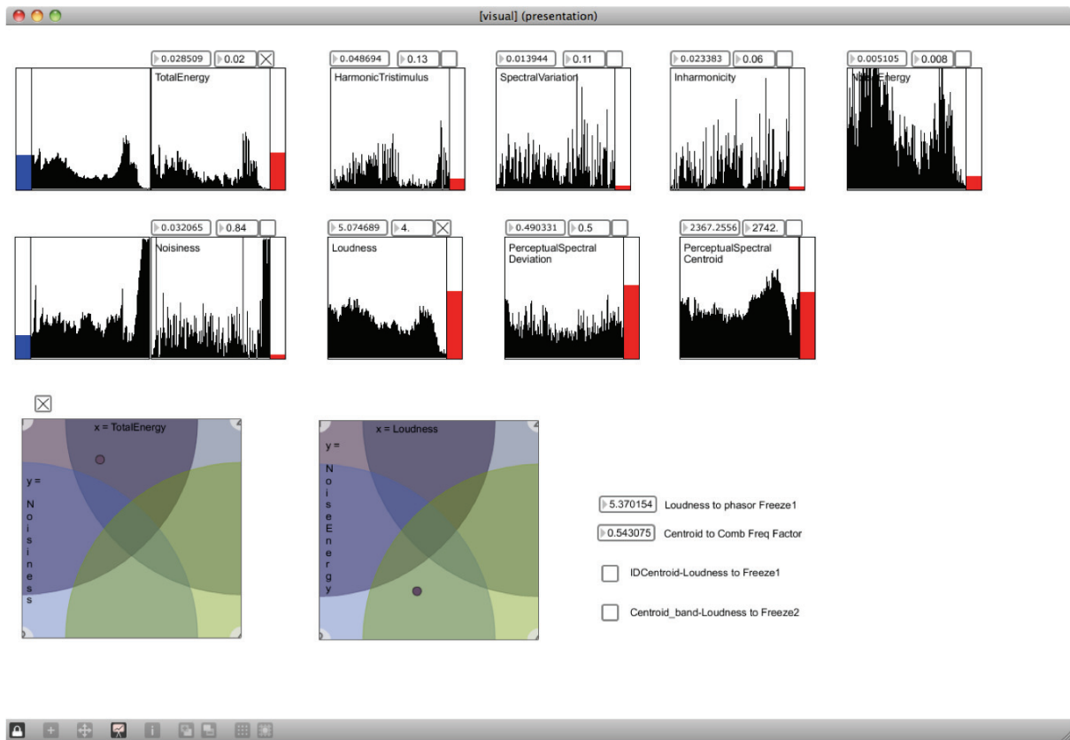
Fig. 34. Représentation graphique des différents descripteurs audio ; en bas, le couplage entre deux descripteurs pour le contrôle d'interpolation des paramètres.
