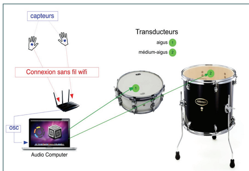
Fig. 67. Schéma technique et disposition des transducteurs sur les peaux des instruments.
