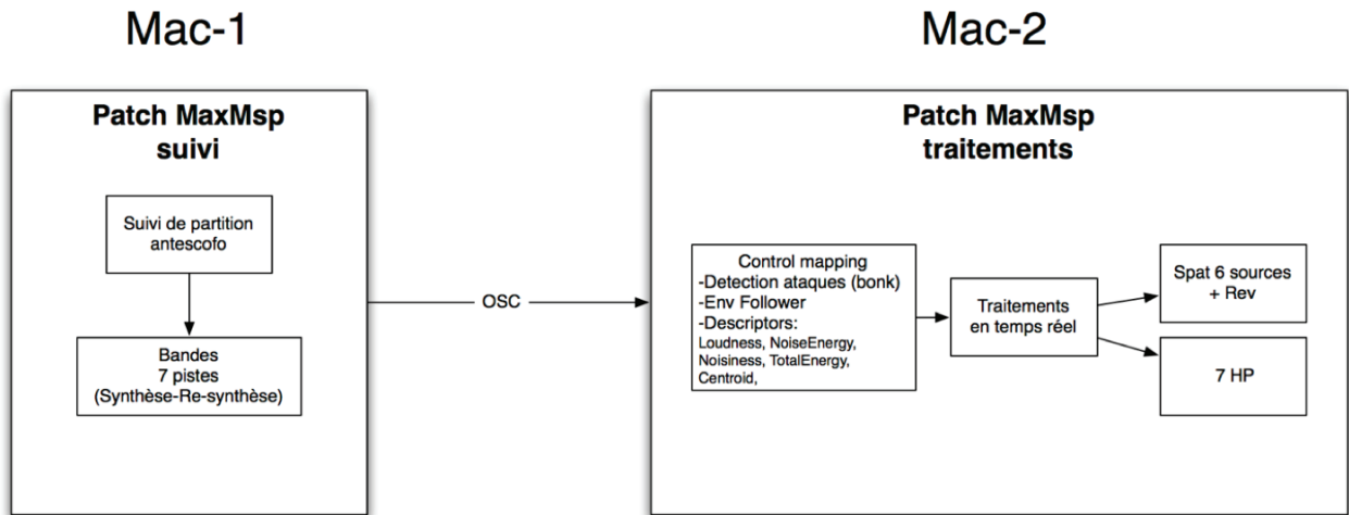
Fig. 28. L'ordinateur Mac-1 avec le suivi de partition Antescofo, déclenche des fichiers audio multicanaux et contrôle l'ordinateur Mac-2 avec les traitements en temps réel.
