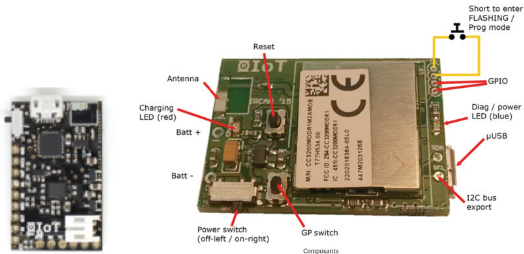
Fig. 22. Bitolino RiOT V3 et IRCAM RiOT V1.
