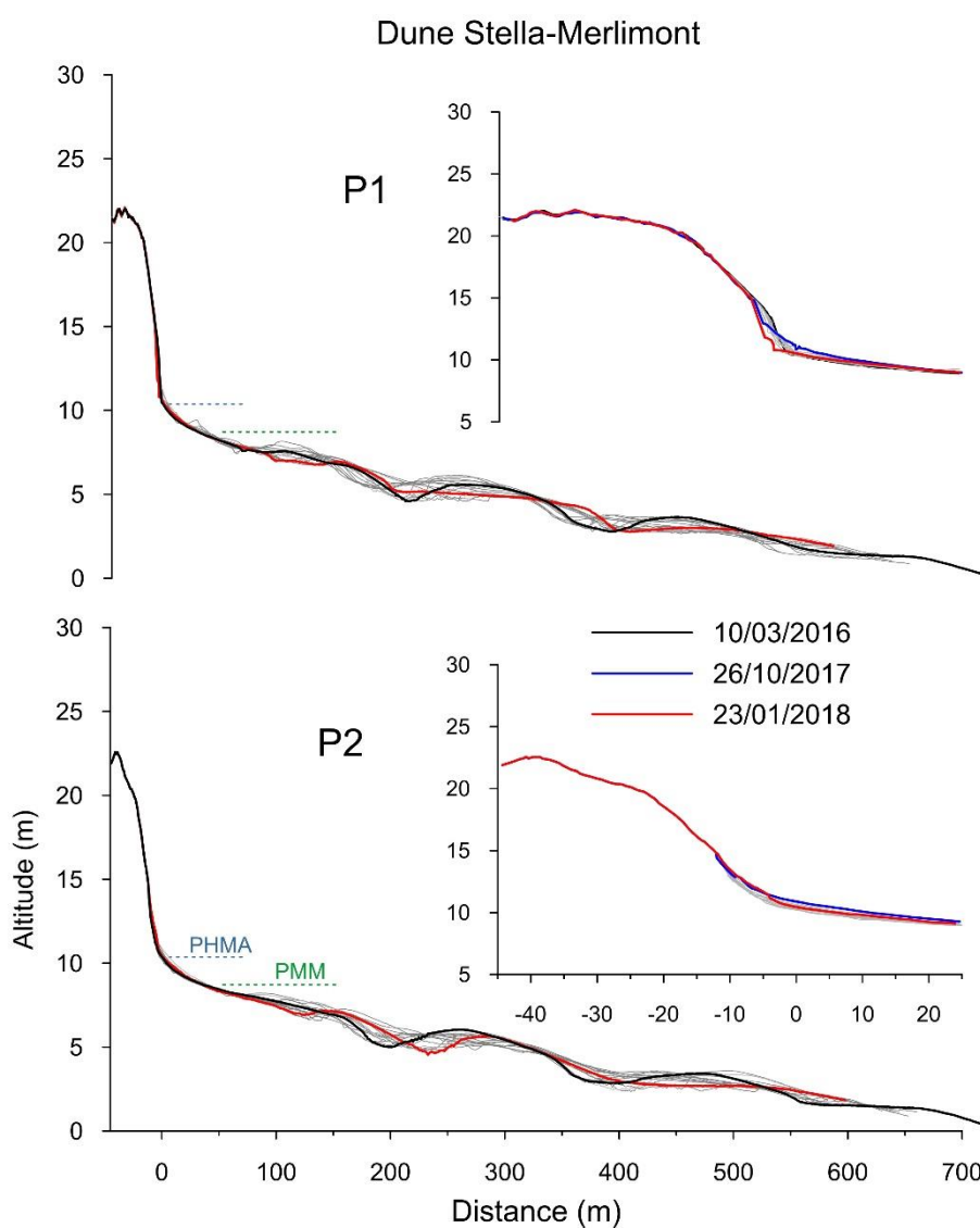
Figure VI-21 : profils topographiques réalisés de mars 2016 à janvier 2018 au niveau de la dune Stella-Merlimont (Annexe IV).
