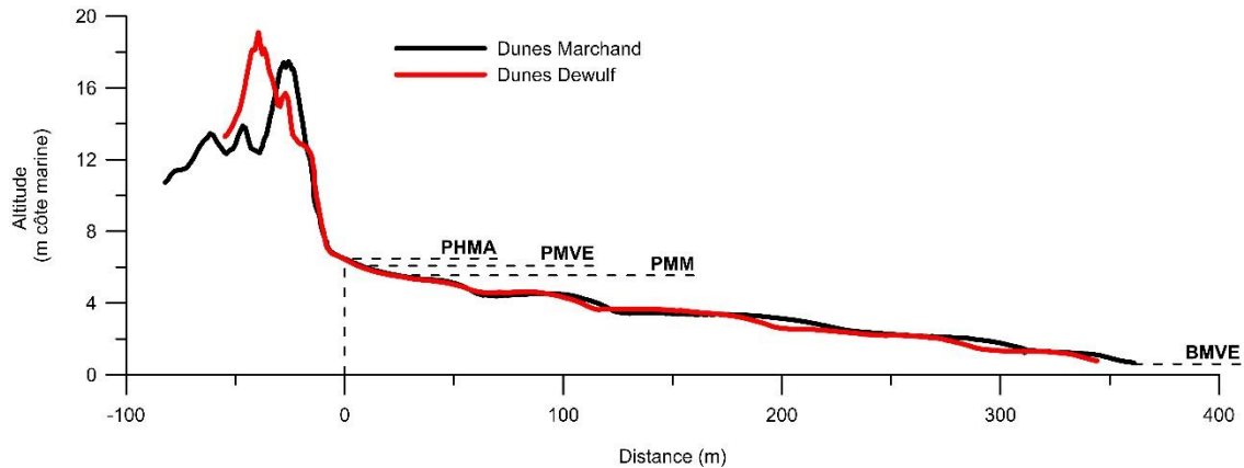
Figure IV-3 : profils topographiques réalisés le 25/02/2016 sur les deux secteurs dunaires du site de Dunkerque.
