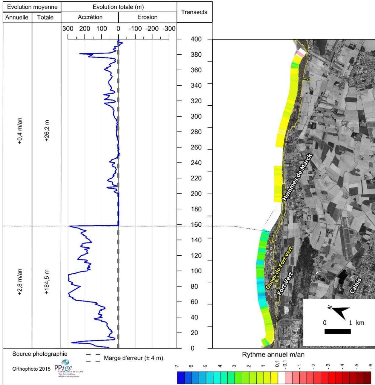
Figure III-9 : évolution du trait de côte à l'est de Calais entre 1949 et 2015 (Annexe I, carte 4).
