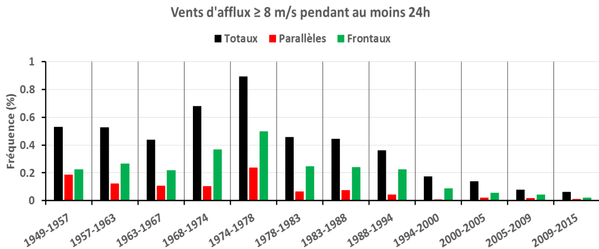
Figure IV-22 : fréquence des vents d'afflux supérieurs ou égaux à 8 m/s pendant au moins 24 heures à Dunkerque.
