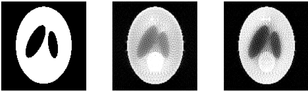
(a) fonction f (b) f_{appr} , méthode de Chang (c) f_1 méthode de Kunyansky
