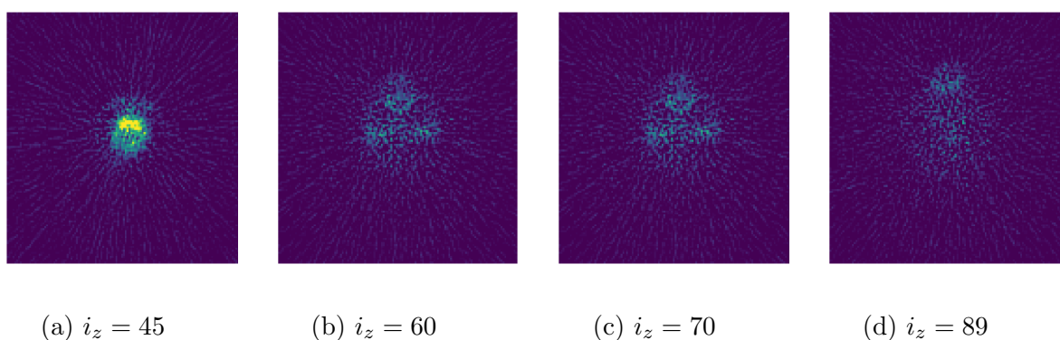
Figure 1.33 : Reconstruction de la distribution des nucléotides dans différents plans z = \text{const} . Notons que le plan i_z = 45 (a) correspond à la région du cerveau du singe.
