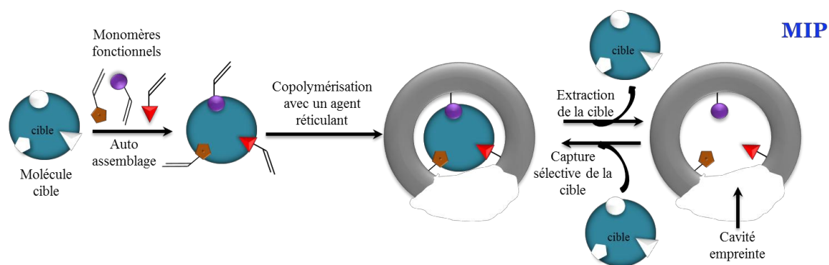
Figure 1-1. Principe des polymères à empreintes moléculaires.
