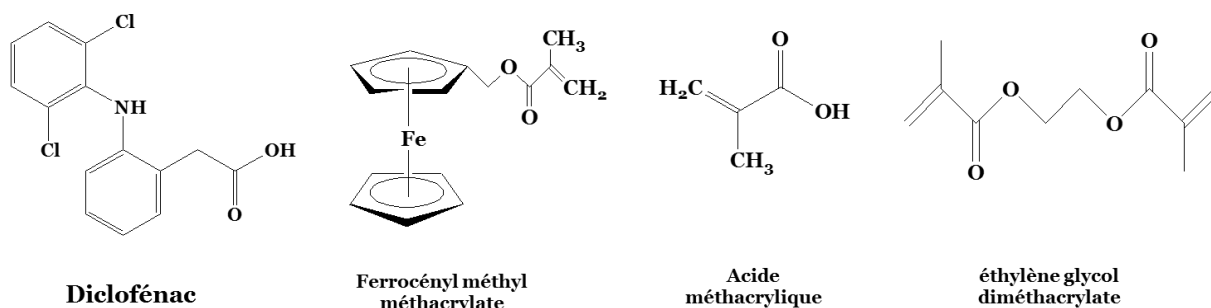
Figure 4-19. Structures des monomères ayant servi à synthétiser e-(MIP/NIP)-Fc18 et e-(MIP/NIP)-Fc26.
