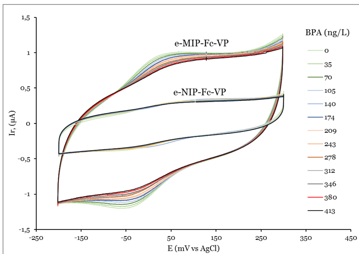
Figure 4-14. Evolution de l'intensité de courant en fonction de la quantité de BPA ajoutée. V=25\text{ mV/s} .
