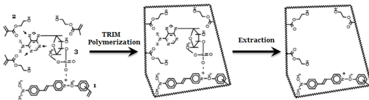
Figure 1-10. Formation de l'empreinte à partir du monomère fonctionnel fluorescent (1) et du monomère fonctionnel 2-hydroxyéthyl méthacrylate (HEMA) (2) disposés autour de la molécule cible, cAMP (3) 33 .
