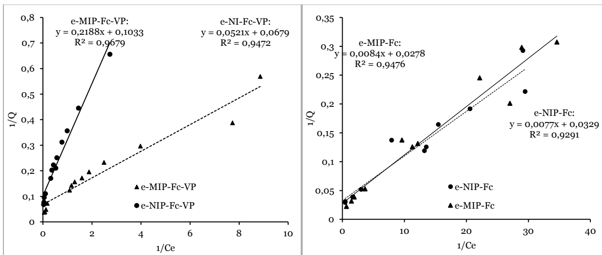
Figure 2-10. Isothermes selon le modèle de Langmuir des e-(MIP/NIP)-Fc et e-(MIP/NIP)-Fc-VP.
