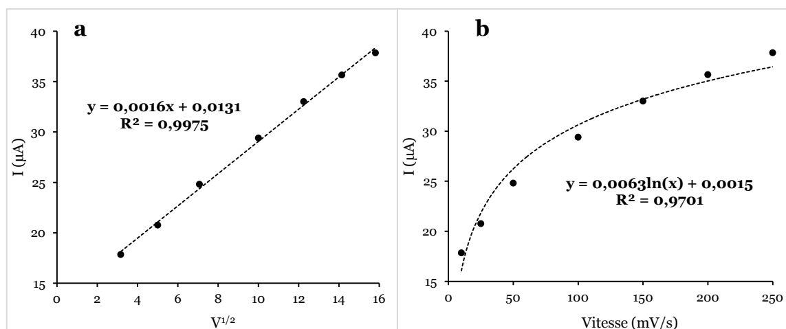
Figure 3-5. (a) Courbe intensité- racine carrée de la vitesse des e-MIP-Fc ; (b) Courbe intensité-vitesse des e-MIP-Fc.
