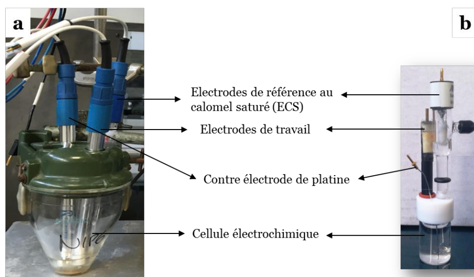
Figure 3-1. Cellules électrochimiques pour les analyses (a) en milieu organique et (b) en milieu aqueux.
