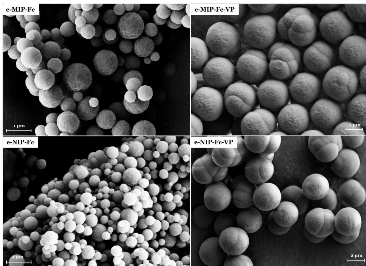
Figure 2-5. Images MEB des e-MIP-Fc et e-MIP-Fc-VP et les poly e-NIP-Fc et e-NIP-Fc-VP non imprimés.
