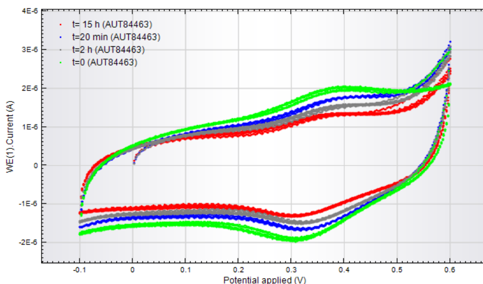
Figure 3-29. Voltampérogrammes cycliques de l'électrode de carbone/e-MIP-Fc, avant (vert) et après ajout de BPA à 20 minutes (bleu), 2h (gris) et 15h (rouge), v=100 \text{ mV/s} .
