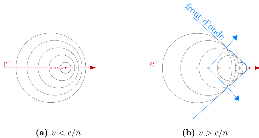
Figure 1.2 – Schéma illustrant l'apparition du rayonnement Cherenkov lorsque la vitesse v de la particule chargée (ici un électron) dépasse c/n . Les cercles représentent les positions spatiales des fronts d'onde successifs rayonnés par les dipôles générés par le passage de la particule chargée.
