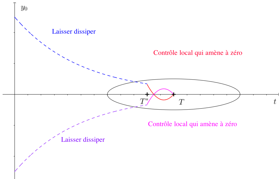
FIGURE 9.1 – Illustration de la preuve du Théorème 9.4.1
