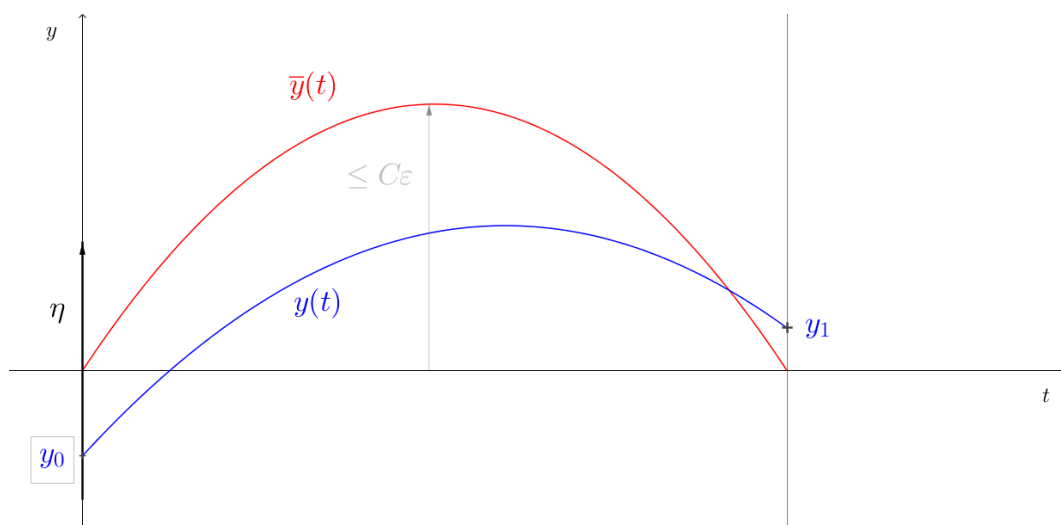
FIGURE 2.1 – Illustration de la méthode du retour
