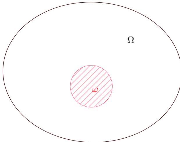
FIGURE 2.2 – L'ouvert \Omega et le sous-ouvert \omega
