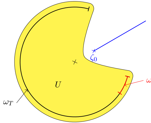
FIGURE 10.1 – Illustration d'un domaine U qui contient \omega_T , contenu strictement dans D(0, 1) .
