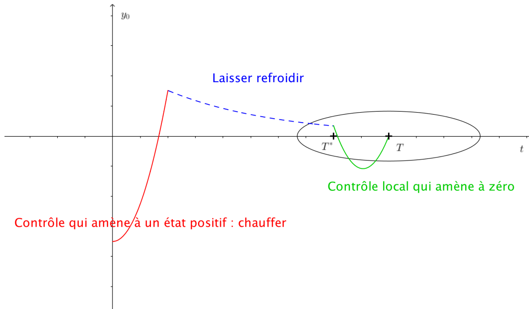
FIGURE 9.2 – Illustration de la preuve du Théorème 9.7.1
