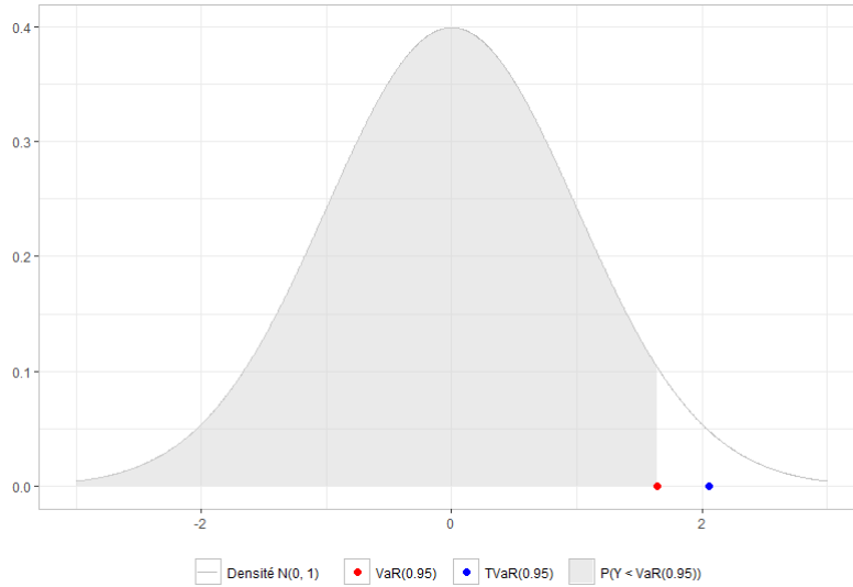
FIGURE A.1 – Valeurs de \text{VaR}_{0.95}[X] (point rouge) et \text{TVaR}_{0.95}[X] (point bleu) pour X distribuée suivant une loi normale centrée et réduite.
