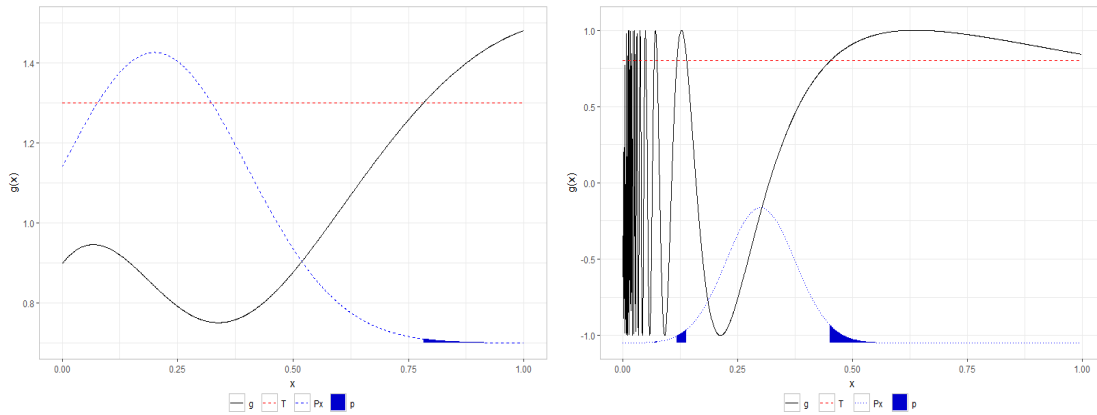
FIGURE 4.1 – À gauche : la fonction vérifie (\mathcal{H}_1) . À droite : la fonction ne vérifie pas (\mathcal{H}_1) .
