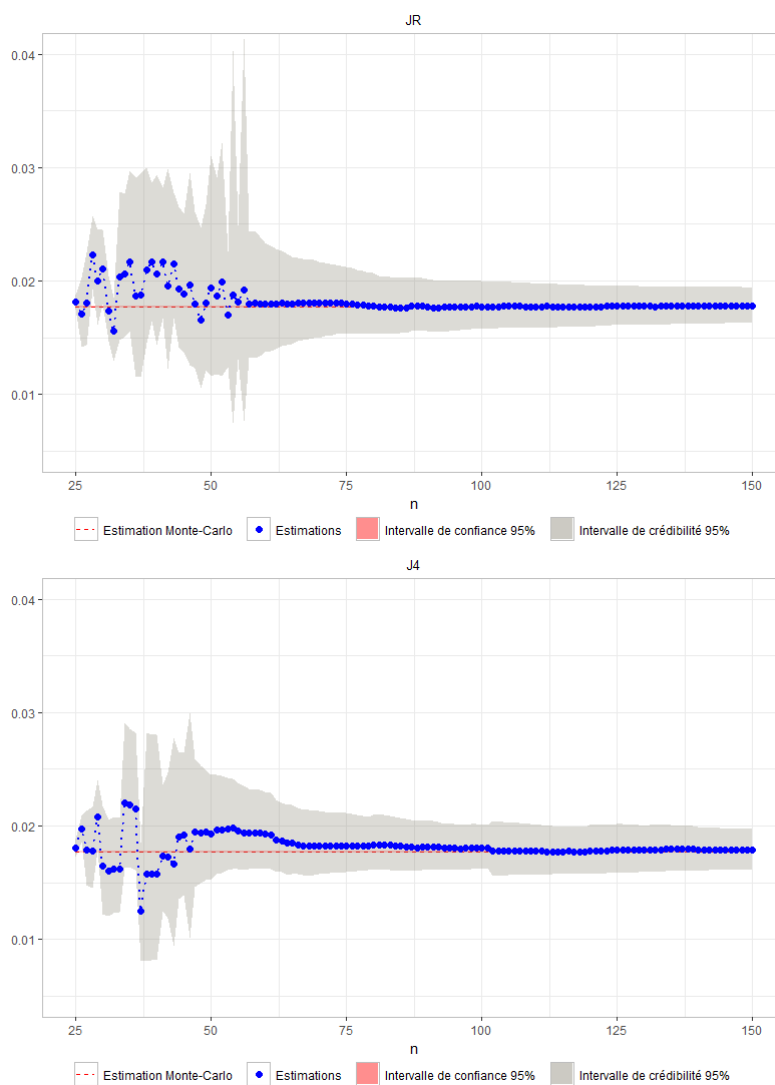
FIGURE 3.8 – Estimations successives de la probabilité de défaillance avec les critères J_{R_n} (en haut) et J_{4,n} (en bas). Ligne en pointillés rouges : l'estimation de la probabilité de défaillance obtenue par application de la méthode Monte-Carlo naïve avec N = 10^7 . Aire rouge : intervalle de confiance à 95% pour p obtenu également par la méthode Monte-Carlo naïve. Puisqu'il est égal à [1.76 \times 10^{-2}, 1.78 \times 10^{-2}] , cet intervalle est à peine visible. Points bleus : estimations successives de p obtenues grâce à l'estimateur (3.5). Aire grise : estimations par la méthode Monte-Carlo naïve de l'intervalle de crédibilité à 95% donné en (3.21).
