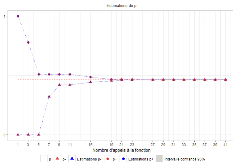
FIGURE 4.13 – Ligne pointillés rouge : la vraie valeur de p . Triangles rouges : les approximations successives p^-(\mathbf{t}) . Points rouges : les approximations successives p^+(\mathbf{t}) . Triangles bleus : les estimations successives \hat{p}^-(\mathbf{t}) de p^-(\mathbf{t}) . Points bleus : les estimations successives \hat{p}^+(\mathbf{t}) de p^+(\mathbf{t}) . Aires grises : les intervalles de confiance à 95% pour les approximations p^-(\mathbf{t}) et p^+(\mathbf{t}) . Ces intervalles étant à peine visibles, on donne en figure 4.14 une version agrandie de ce graphique.
