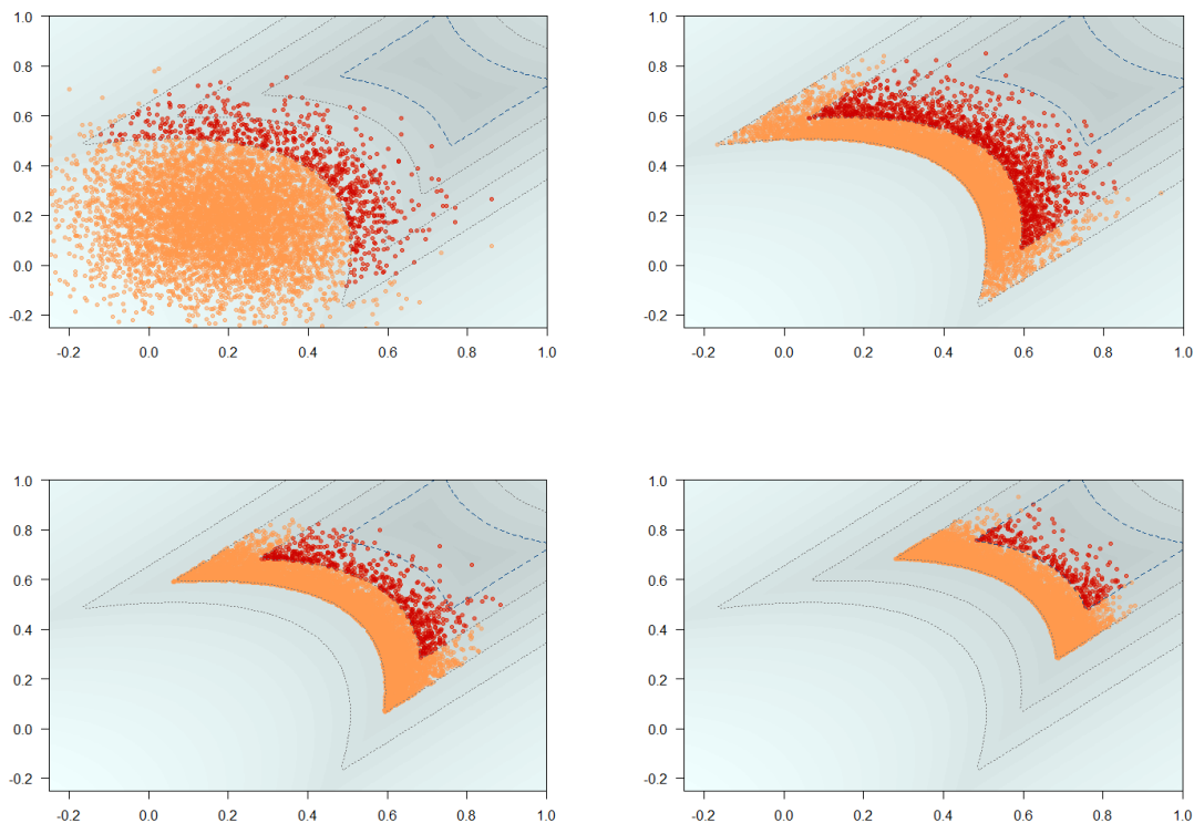
FIGURE 2.2 – Illustration du principe de la méthode de splitting. La frontière du domaine de défaillance \mathbb{F} est la ligne de niveau en tirets bleus. Les frontières des domaines de défaillance intermédiaires sont les lignes de niveaux en pointillés gris. L'estimateur de p est égal au produit des proportions de points rouges. L'estimation de p qui en retourne est donc non-nulle, alors qu'une estimation directe par la méthode Monte-Carlo naïve est égale à 0 (voir figure en haut à gauche, où l'échantillon est simulé suivant la loi initiale et où aucun point ne tombe dans le domaine de défaillance).
