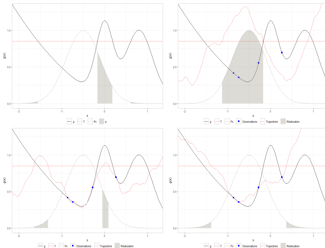
FIGURE 3.1 – En haut à gauche : la probabilité cible p (aire grise). En haut à droite : exemple d’une réalisation de la variable aléatoire S définie en (3.2) (aire grise). La courbe rouge est la trajectoire d’un processus gaussien dont la loi n’est pas conditionnée aux observations (points bleus). En bas : exemple de réalisations de la variable aléatoire S_n définie en (3.3) (aires grises). L’approximation de p est meilleure à gauche qu’à droite. Les courbes rouges sont les trajectoires d’un processus gaussien dont la loi est conditionnée aux observations (points bleus).
