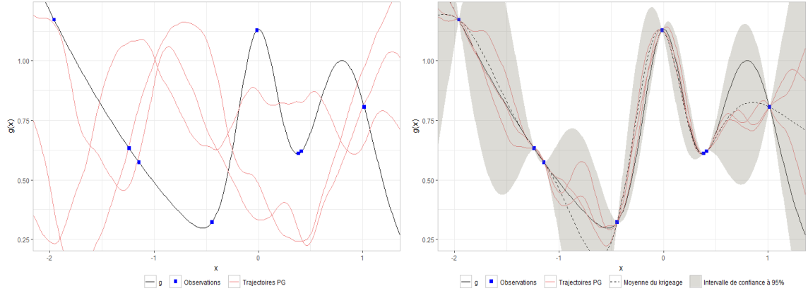
FIGURE 2.4 – Exemple de modélisation par processus gaussien. Courbe noire : fonction g que l'on cherche à modéliser. Points bleus : valeurs observées de g . À gauche : trajectoires du processus gaussien distribué suivant la loi du modèle (2.13). À droite : trajectoires du processus gaussien distribué suivant la loi conditionnée aux observations, donnée en proposition 2.3.1. La courbe noire en pointillés est la moyenne (2.16) et les surfaces grises sont des intervalles de confiance à 95%.
