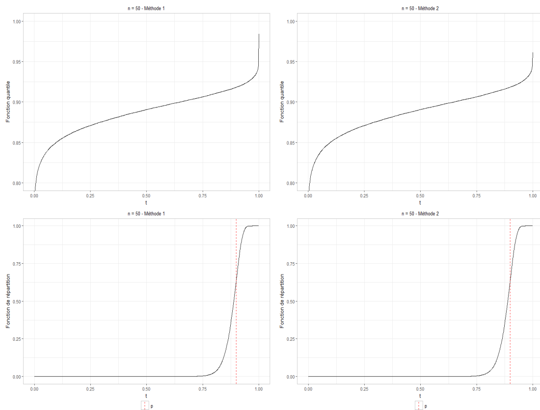
FIGURE B.2 – Droite en pointillés rouge : la vraie probabilité de défaillance p . À gauche : la fonction quantile (en haut) et la fonction de répartition (en bas) de R_n , par application de la méthode 1. À droite : la fonction quantile (en haut) et la fonction de répartition (en bas) R_n par application de la méthode 2.
