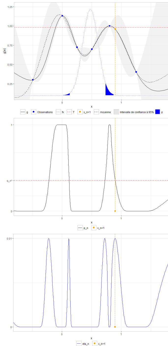
FIGURE 3.5 – Exemple simple pour aider à l’interprétation du critère J_{R_n} . En haut : la fonction g (courbe noire) est observée en n = 6 points et l’aire bleue sous la densité f_{\mathbf{X}} est la probabilité p . Au milieu : représentation de la fonction \mathbf{x} \in \mathbb{X} \mapsto p_n(\mathbf{x}) et de la valeur de q_n^* donnée en proposition 3.6.3. En bas : représentation de la fonction \mathbf{x} \in \mathbb{X} \mapsto \eta_n(\mathbf{x}) définie dans la proposition 3.6.2. Les points dans \mathbb{X} où \eta_n est maximale (par exemple, le point orange) conduisent à p_n = q_n^* . Il s’agit de points où le modèle de processus gaussien a ses trajectoires relativement proches du seuil T et doit être renseigné pour améliorer l’estimation de p .
