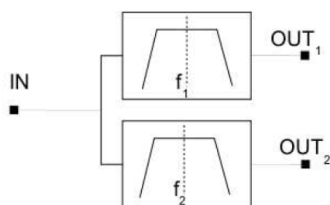
FIGURE 3.9 – Schéma d'un duplexeur. IN : entrée du signal, OUT : sorties pour chacun des signaux séparés.
