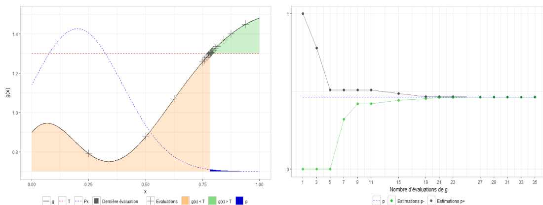
FIGURE 4.12 – À gauche : résultat de l’algorithme une fois le budget de n = 35 évaluations atteint. À droite : approximations successives en fonction du nombre d’appels à la fonction g . En bleu : la vraie probabilité de défaillance p . En gris : l’approximation par excès p^+(\mathbf{t}) . En vert : l’approximation par défaut p^-(\mathbf{t}) .
