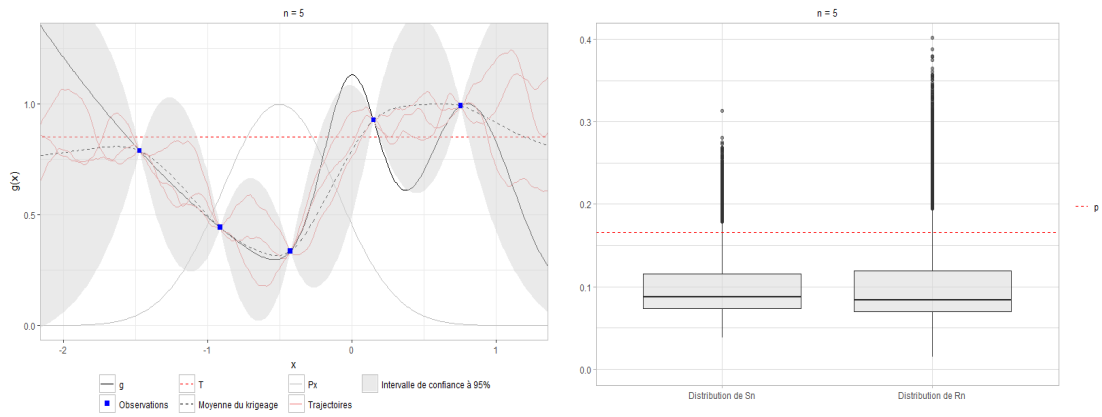
FIGURE 3.2 – À gauche : modèle de processus gaussien pour n = 5 évaluations de la fonction g (représentée par la courbe noire). À droite : distributions empiriques de S_n et R_n .
