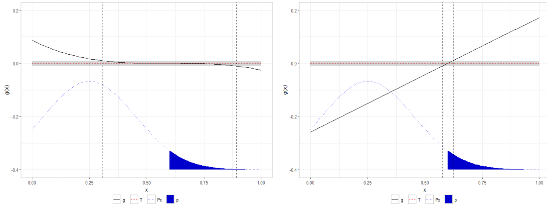
FIGURE 4.3 – Exemples de fonctions qui vérifient (\mathcal{H}_1) avec la même constante L \approx 0.4 . À gauche : la fonction vérifie (\mathcal{H}_2) avec C \gg 1 . À droite : la fonction vérifie (\mathcal{H}_2) avec C = 1 .
