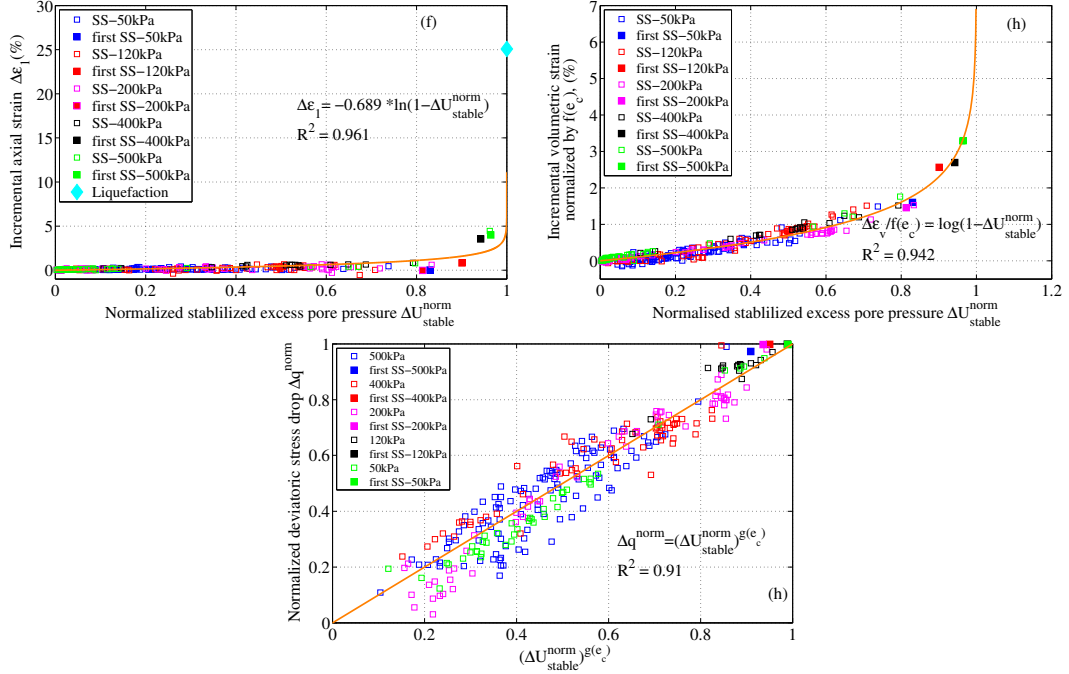
Figure E.2: Effets de surpression interstitielle stable et normalisée \Delta U_{stable}^{norm} sur l'incrément des déformations axiales \Delta \varepsilon_1 , l'incrément des déformations volumiques \Delta \varepsilon_{vol} et la chute du déviateur normalisé \Delta q_{norm} en frottements saccadés.
