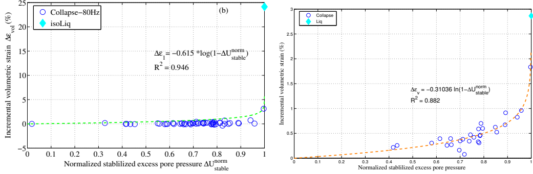
Figure E.3: Effets de surpression interstitielle stable et normalisée \Delta U_{stable}^{norm} sur l'incrément des déformations axiales \Delta \varepsilon_1 , l'incrément des déformations volumiques \Delta \varepsilon_{vol} en consolidation isotrope.
