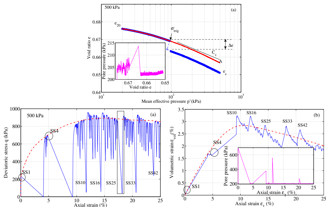
Figure E.1: Frictions saccadées en consolidation isotrope et en compression triaxiale drainée à 500 kPa.
