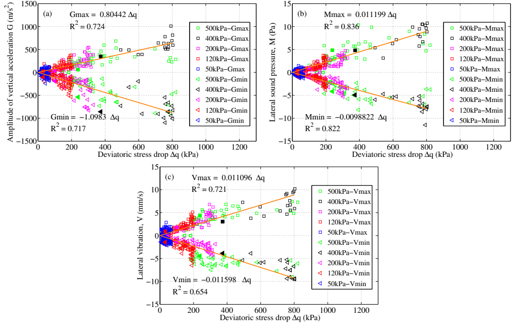
Figure E.4: Effets de l'accélération verticale G , pression acoustique horizontale M , vibration horizontale V sur la chute du déviateur \Delta q en frottements saccadés.
