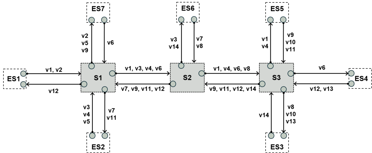
Figure 5 – Exemple de configuration réseau AFDX comprenant de multiples VL unicasts.
