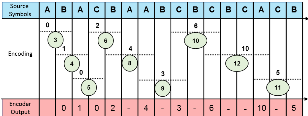
Figure 67 – Exemple simplifié de l'algorithme LZW : réception initiale de symboles sources et séquence encodée de mots de code.
