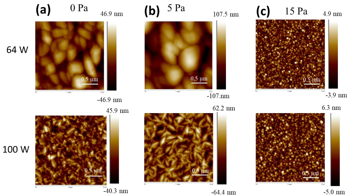
Figure IV. 10 : Topographies C-AFM des couches de TiO 2 préparées à 64 W et à 100 W (a) non dopées, (b) dopées à 5 Pa et (c) dopées à 15 Pa.
