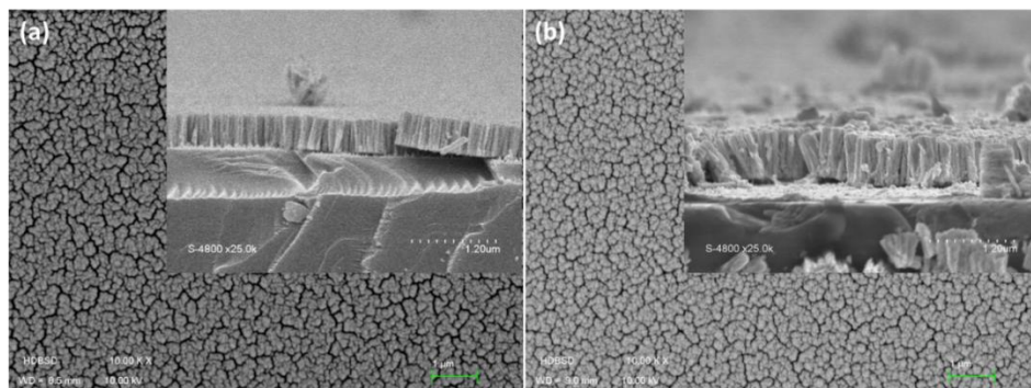
Figure A1. 5 : Morphologies surfaciques de couches de Pt sur Si pour un même temps de dépôt de 45 min à (a) 20 Pa et (b) 30 Pa.
