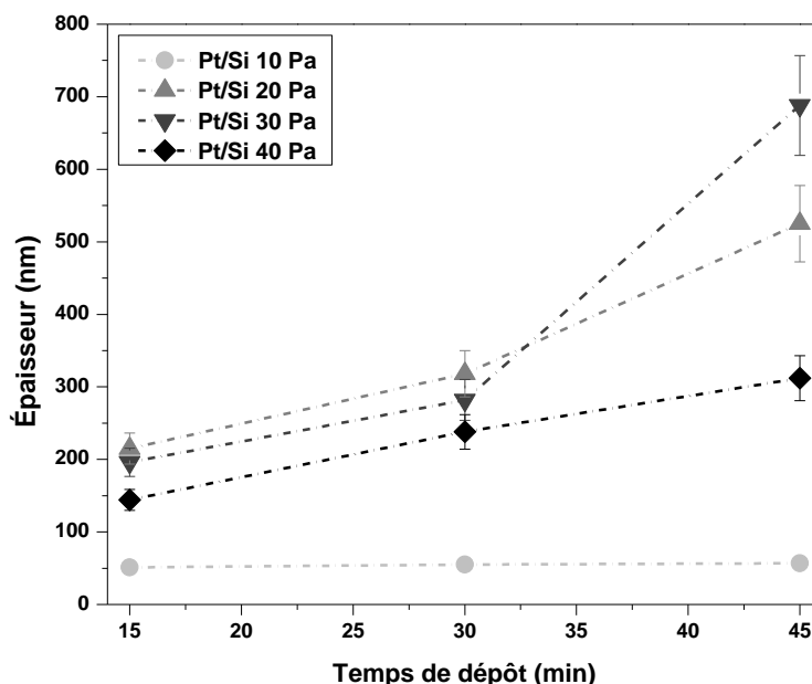
Figure A1. 6 : Variation de l'épaisseur des couches de Pt sur Si à 10 Pa, 20 Pa, 30 Pa et à 40 Pa en fonction du temps de dépôt.
