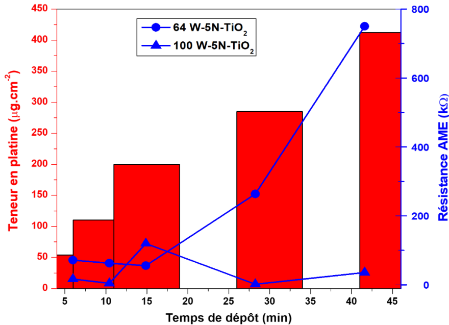
Figure A2. 7 : Variation de la résistance globale des AME en fonction de la teneur en platine dans les contre-électrodes et pour les anodes de TiO 2 dopées à l'azote à 5 Pa.
