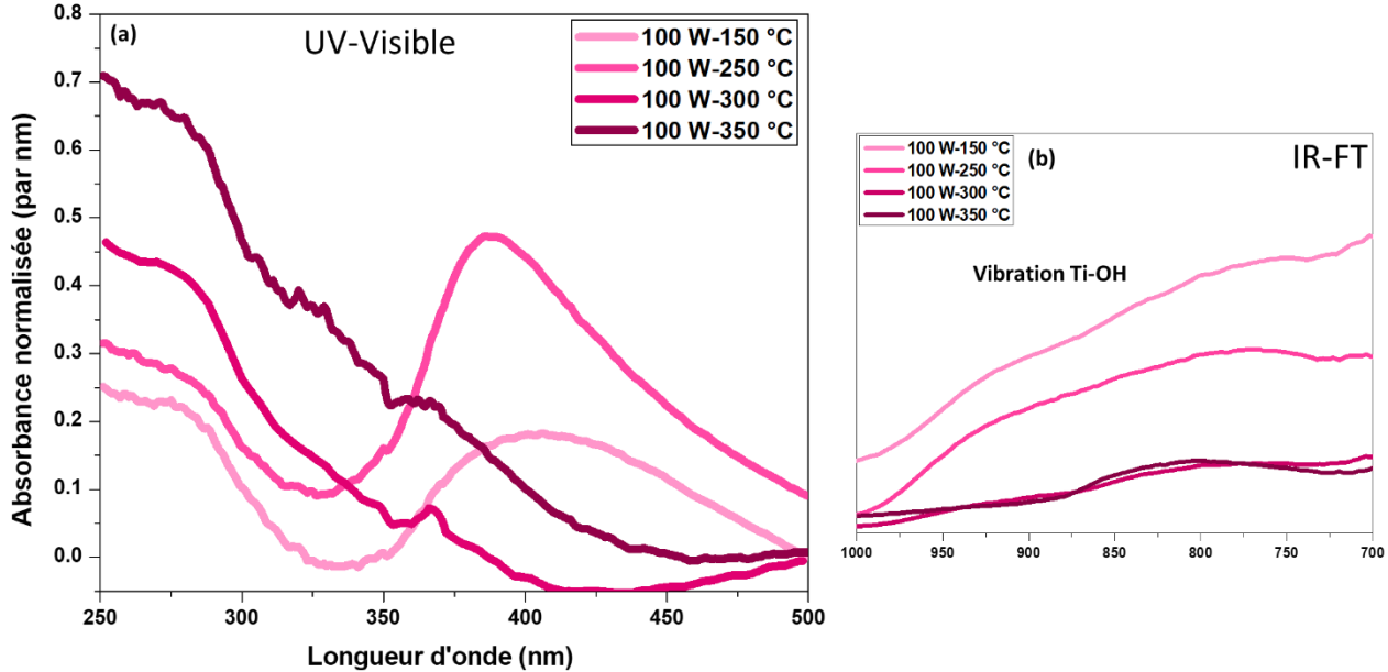
Figure III. 14 : Représentation des (a) spectres UV-Visible des couches de TiO 2 déposées sur Si à 100 W et 150 °C, 250 °C, 300 °C, 350 °C accompagnées (b) des spectres IRTF de la zone concernée.
