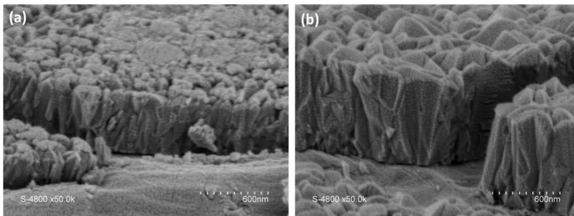
Figure A2. 8 : Clichés MEB des sections de couches de \text{TiO}_2 dopées à 5 Pa à l'azote et déposées à (a) 64 W et (b) 100 W.
