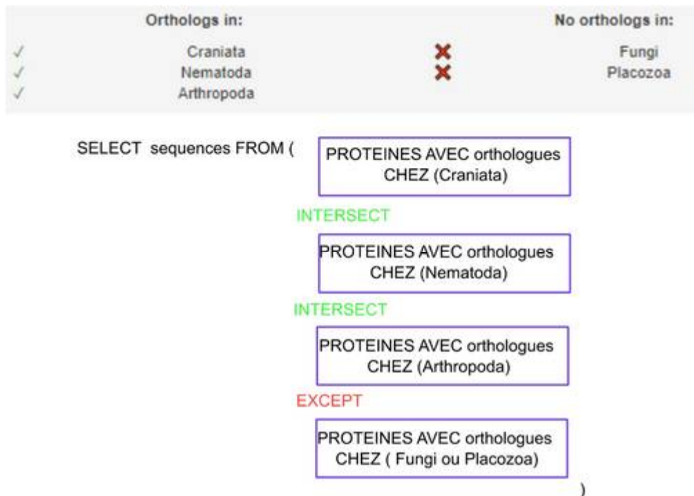
Figure 7-2 Structure modulaire des recherches par profil. Le bloc de base, en violet, permet de retrouver toutes les protéines ayant un orthologue dans au moins une espèce d'une liste donnée. On enchaîne autant de ces blocs que de contraintes de présence avec le mot clé INTERSECT, et on y rajoute un bloc commun pour toutes les contraintes d'absence avec le mot clé EXCEPT.
