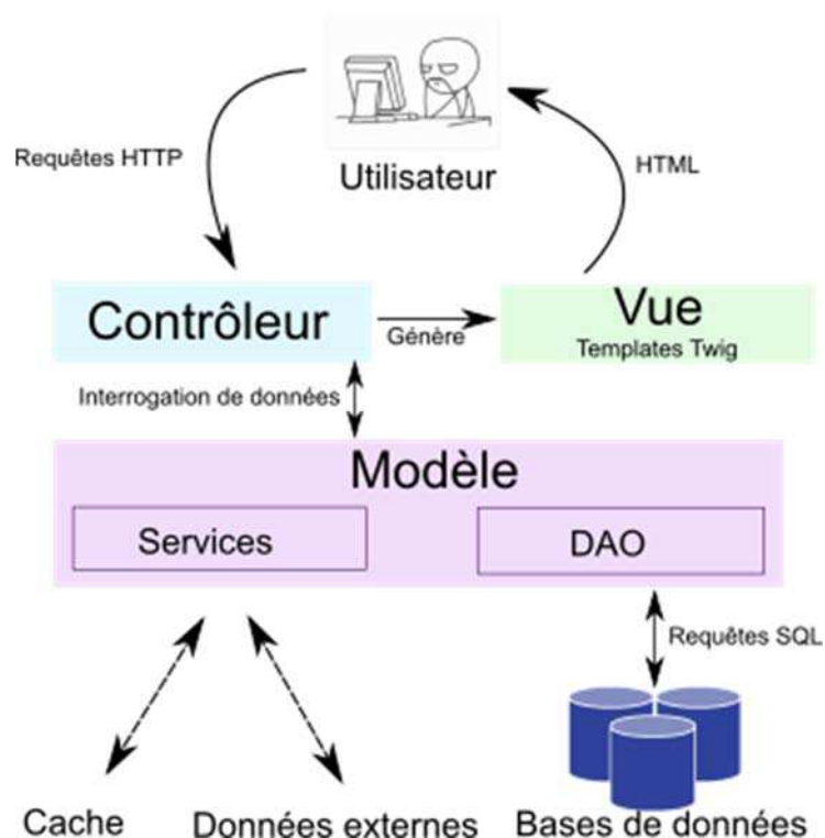
Figure 7-1 Organisation technique du portail OrthoInspector. Le code est séparé en trois modules. Le Contrôleur gère les requêtes de l'utilisateur, interroge les données via les sections de la partie Modèle, et utilise les données traitées à la partie Vue pour générer le code HTML visualisé par l'utilisateur.
