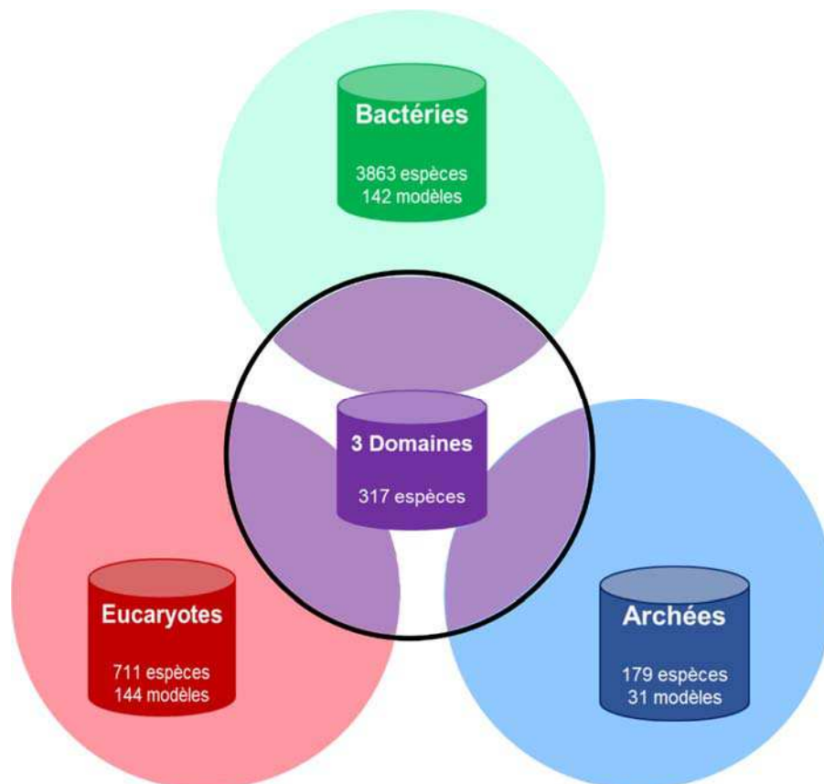
Figure 4-6 Architecture de données d'OrthoInspector 3.0. La ressource repose sur quatre bases complémentaires, trois bases de données 'exhaustives' et spécifiques à chaque domaine, et une base de données inter-domaines avec seulement des espèces modèles de chacun des trois domaines.
