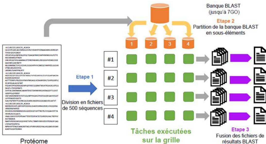
Figure 4-8 Protocole des comparaisons tous-contre-tous . Les protéomes sont divisés en fichiers de 500 séquences et les requêtes sont effectuées sur la grille sur des partitions de la base BLAST conçue à partir de l'ensemble des protéomes. Les fichiers issus de ces comparaisons multiples sont ensuite fusionnés.
