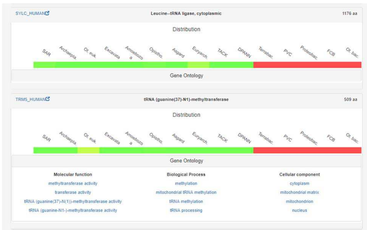
Figure 5-3 Visualisation synthétique des protéines dans la recherche par profil. Deux encarts de protéines sont représentés, chacun est décrit par l'identifiant, la description et la longueur de la protéine. On y retrouve la distribution synthétique de la protéine et un volet détaillant les annotations Gene Ontology associées.
