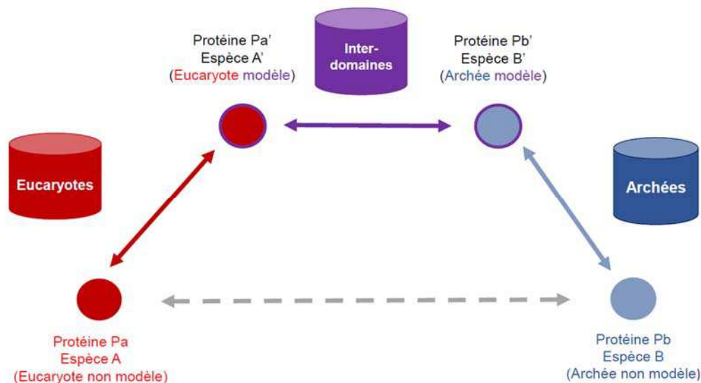
Figure 4-7 Prédiction par transitivité entre espèces non-modèles. La relation d'orthologie entre Pa et Pb (en pointillé), deux protéines d'espèces non modèles Eucaryotes et Archées, n'est pas directement disponible dans OrthoInspector 3.0. On peut les retrouver par transitivité en passant par des orthologues dans les espèces modèles proches.
