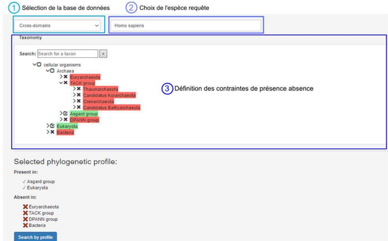
Figure 5-2 Interface de recherche par profil phylogénétique. Les paramètres se définissent en 3 étapes indiquées sur la figure. La sélection des contraintes de présence-absence se fait au niveau des clades dans un arbre taxonomique interactif.
