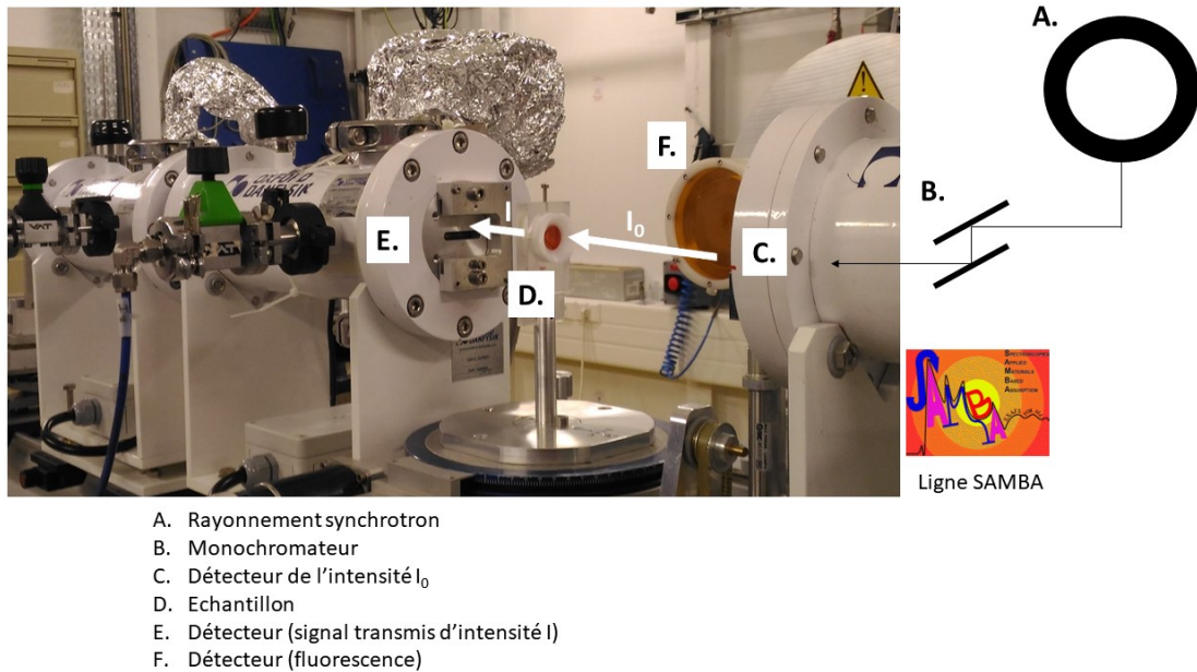
FIGURE E.2 – Schéma de fonctionnement de la ligne SAMBA du Synchrotron SOLEIL
