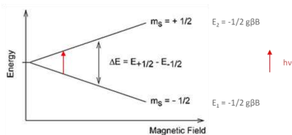
Figure II-7 : Schéma de la levée de dégénérescence des états de spin en présence d'un champ magnétique
