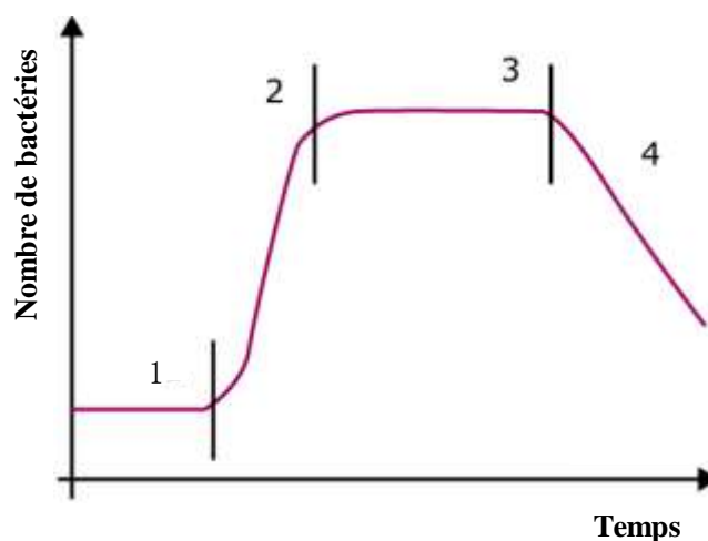
Figure VI-5 : Courbe de croissance théorique de micro-organismes, constituée de quatre phases : 1) Phase de latence, 2) Phase exponentielle, 3) Phase stationnaire, 4) Phase de déclin
