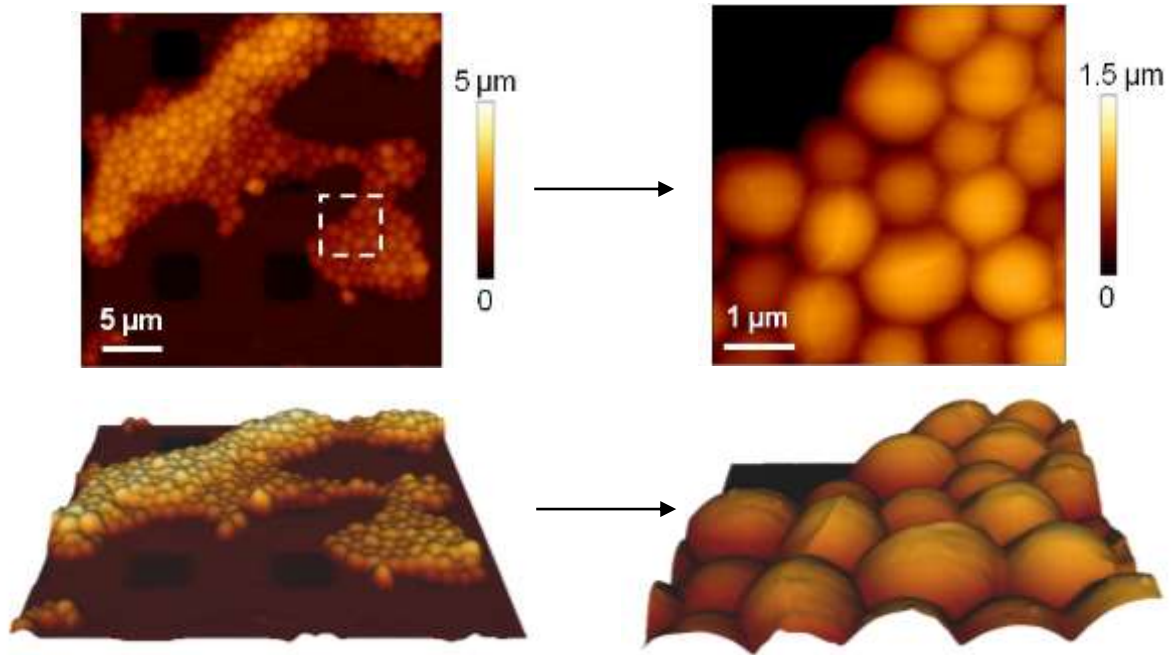
Figure VI-4 : Observation en AFM liquide d'agrégats de la souche ATCC 35984. Les images de droite sont extraites de la zone représentée par un carré blanc sur l'image de gauche. Sous chaque image AFM en 2D, une image en 3D de la même zone est présentée.
