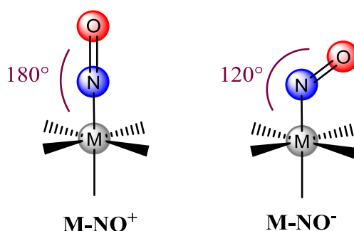
Figure I-23 : Les deux géométries possibles de la liaison M-N-O
