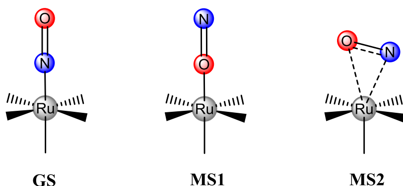
Figure II-1 : Les configurations des différents états GS, MS1 et MS2 (d'après Rose et al. , Coord. Chem. Rev. , 2008)
