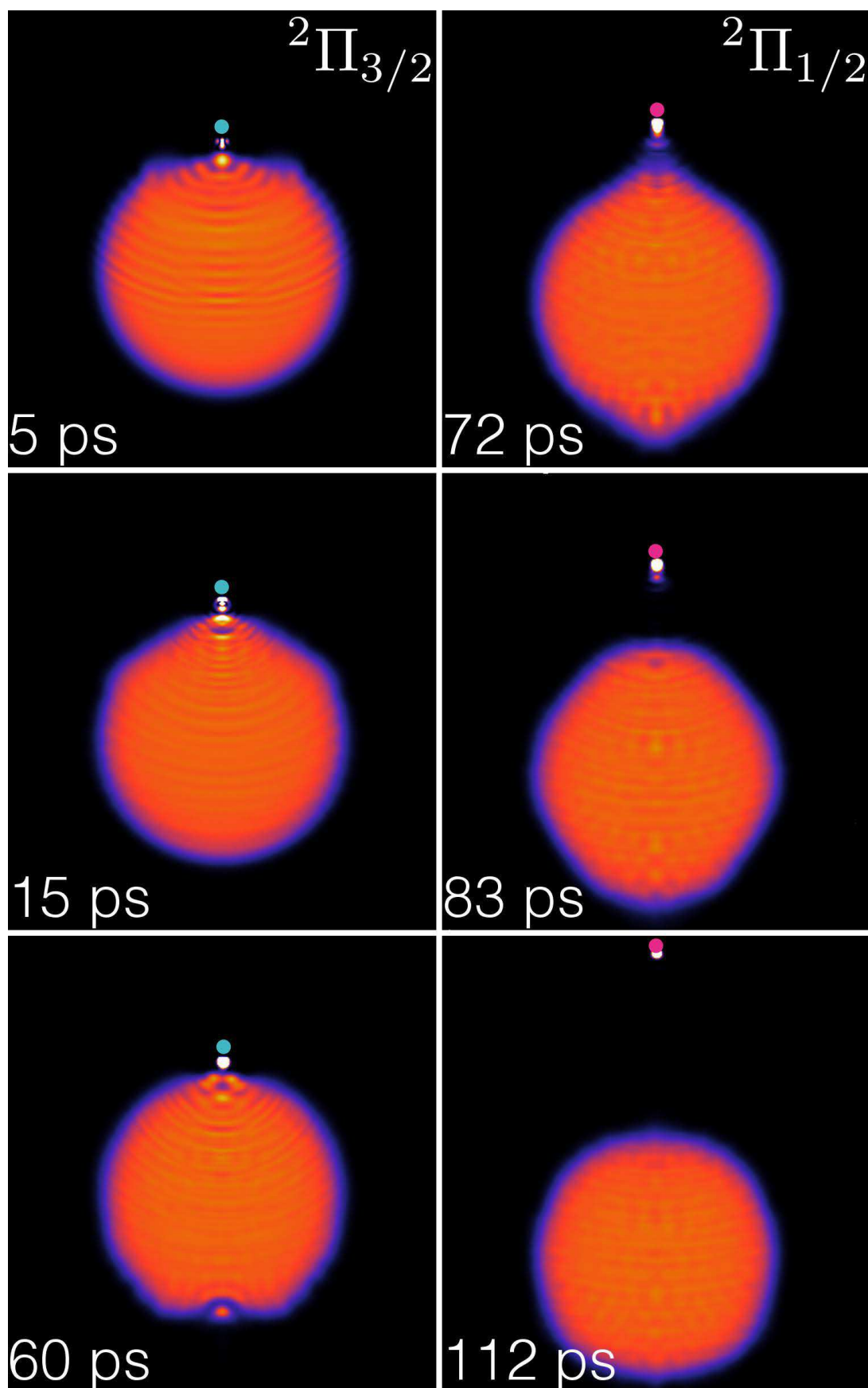
Figure 2: Instantanés de la densité de l'hélium au cours de l'évolution du complexe RbHe 1000 excité pour \eta=15\% , \Delta t=60 ps. Le point vert représente l'atome Rb, excité à l'état 5p\Pi_{3/2} ; le point magenta est l'atome Rb après une relaxation soudaine à l'état 5p\Pi_{1/2} . (Voir Chapitre 5 de la thèse.)
