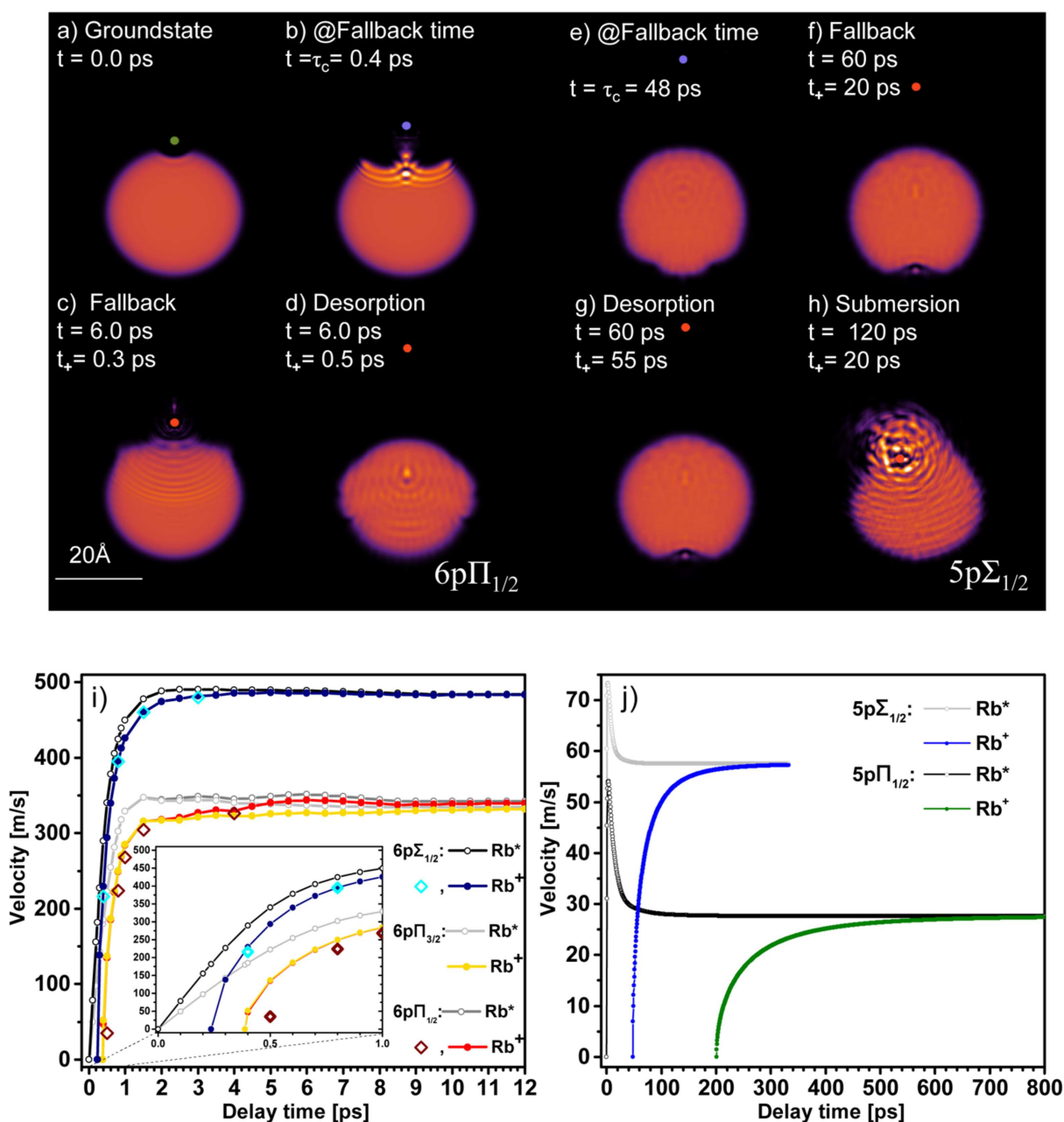
Figure 1: Densités 2D (a–d,e–h) et vitesses basées sur TDDFT (i,j) pour un atome de Rb attaché à une goutelle He 1000 et excité depuis l'équilibre (a) vers des états 6p (colonne de gauche) et 5p (colonne de droite). Les densités sont représentées pour différents temps total de propagation t et différents instants d'ionisation t_+ : (b,e) Rb neutre à t = \tau_c (« fall-back time », temps critique de retour); (c,f) ionisation à t_+ < \tau_c , l'ion Rb + retombe sur la nanogoutelle; (d,g) t_+ > \tau_c , désorption de Rb + ; (h) solvation de Rb + ; (i,j) évolution des vitesses Rb* avec le temps t (symboles gris vides), et vitesses finales de Rb + (symboles pleins) en fonction de t_+ . (Voir Chapitre 4 de la thèse.)
