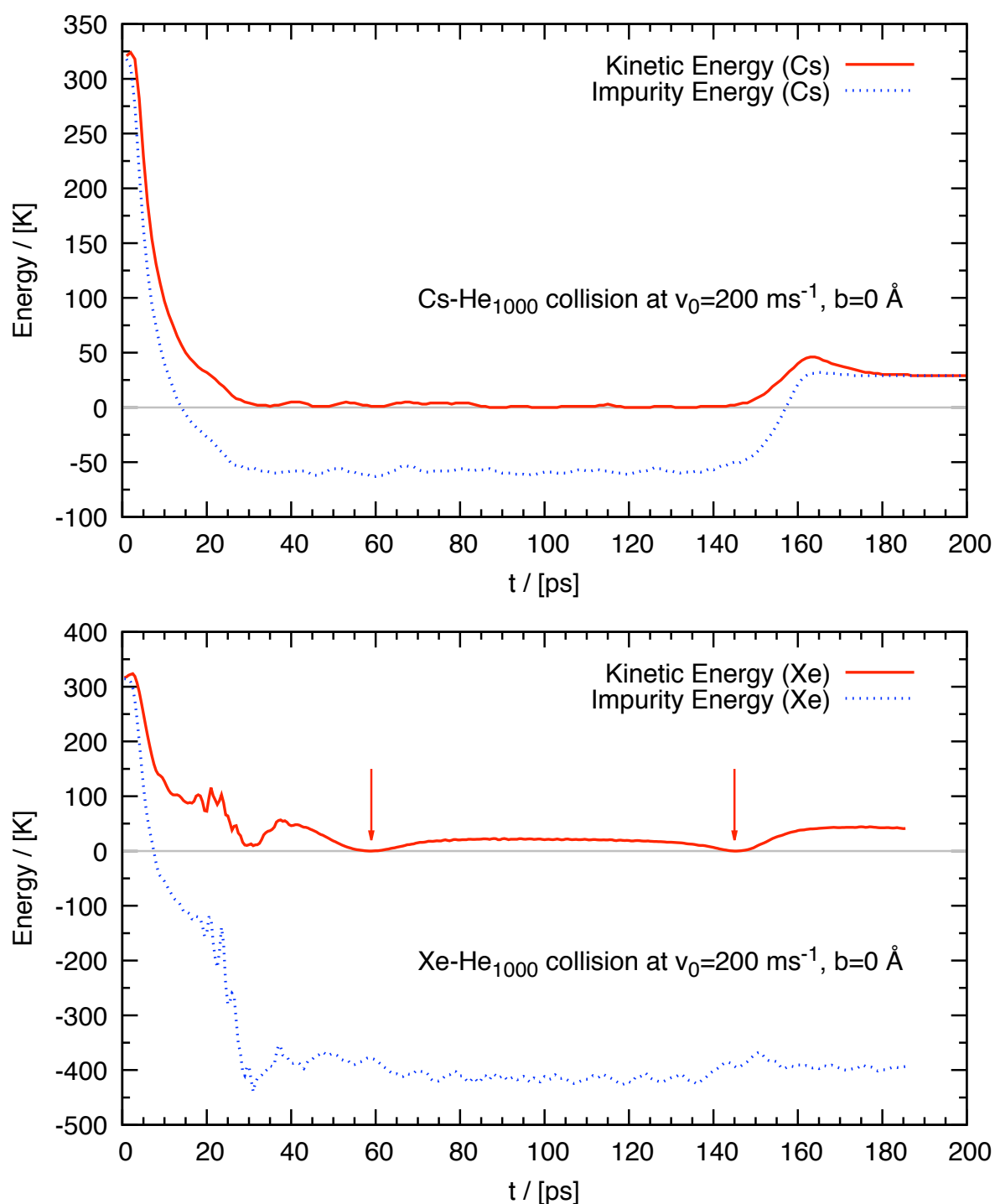
Figure 3: Figure supérieure : Énergie cinétique et totale (cinétique et potentielle) en fonction du temps d'un atome de Cs, collision frontale contre une gouttelette de {}^4\text{He}_{1000} à v_0=200 m/s. Figure inférieure : même que le figure supérieur pour un atome de Xe. Les flèches verticales indiquent les deux premiers points de virage à 59 et 145 ps, dont les densités d'hélium correspondantes sont indiquées dans la colonne de droite de la Figure 8.2. (Voir Chapitre 8 de la thèse.)
