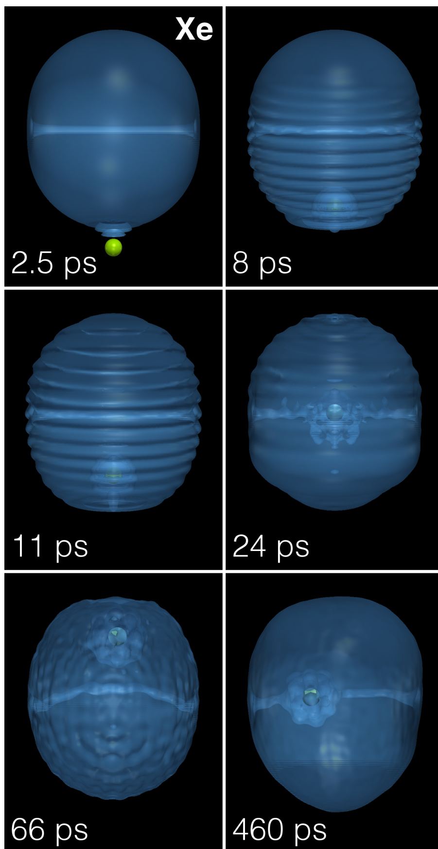
Figure 4: Evolution dynamique d'un atome de Xe (point vert) en collision avec une gouttelette de ^4\text{He}_{1000} hébergeant une ligne de vortex à v_0=200 m/s. Le temps correspondant est indiqué dans chaque image. (Voir Chapitre 9 de la thèse.)
