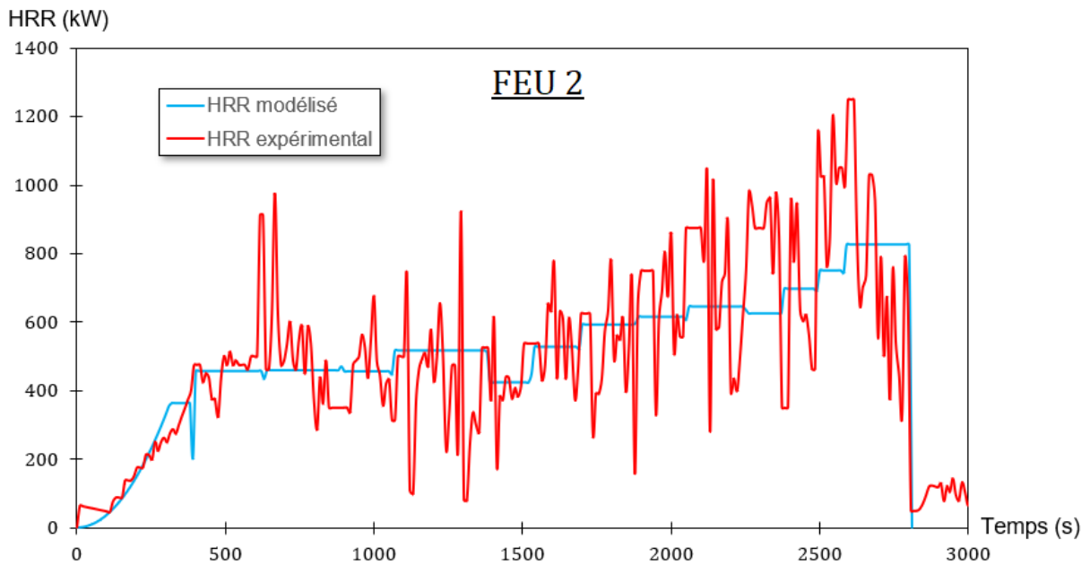
Figure 4.13 – Comparaison des HRR modélisés et expérimentaux pour le deuxième feu de la carrière de Lugasson.
