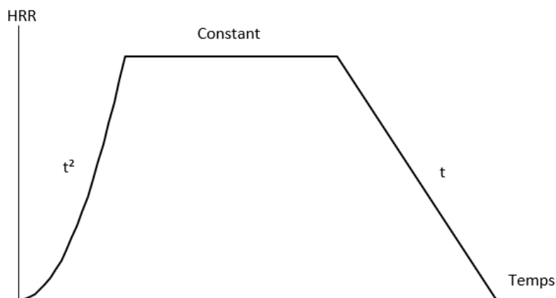
Figure 4.9 – Courbe conventionnelle du HRR selon le modèle des wood cribs .
