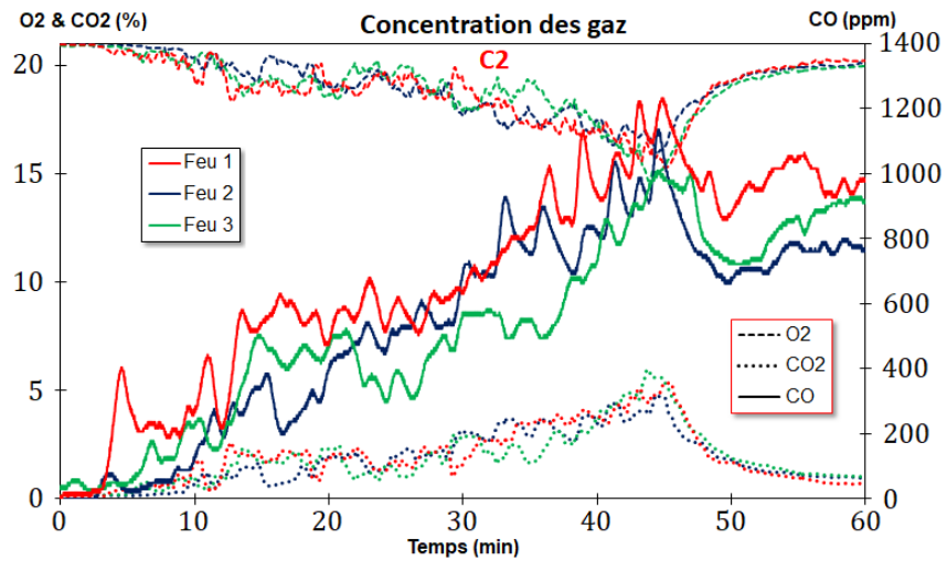
Figure F.2.9 – Mesures des concentrations de gaz effectuées en C2.
