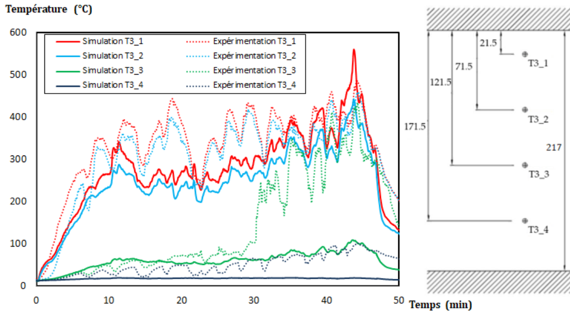
Figure 3.22 – Températures simulées et mesurées par les thermocouples de l'arbre T3. La localisation des thermocouples est indiquée à droite.
