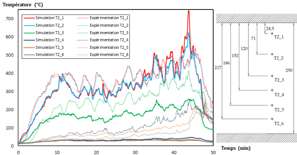
Figure 3.21 – Températures simulées et mesurées par les thermocouples de l'arbre T2. La localisation des thermocouples est indiquée à droite.
