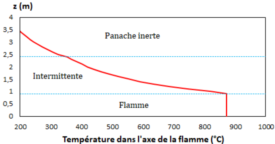
Figure 1.10 – Profil de température dans le panache thermique issu d'un foyer de 600 \text{ kW} et de 80 \text{ cm} de diamètre.
