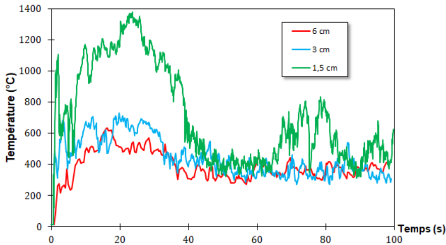
Figure 3.11 – Comparaison des températures dans la flamme pour 3 maillages (1,5 cm, 3 cm et 6 cm).
