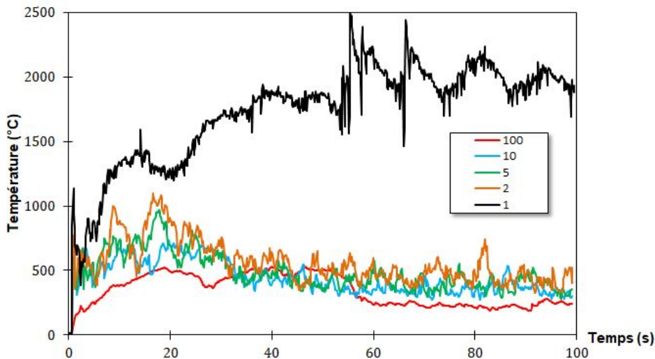
Figure 3.16 – Comparaison des températures dans la flamme pour 5 fréquences (1, 2, 5, 10 et 100).
