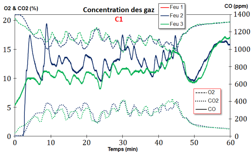
Figure F.2.8 – Mesures des concentrations de gaz effectuées en C1.
