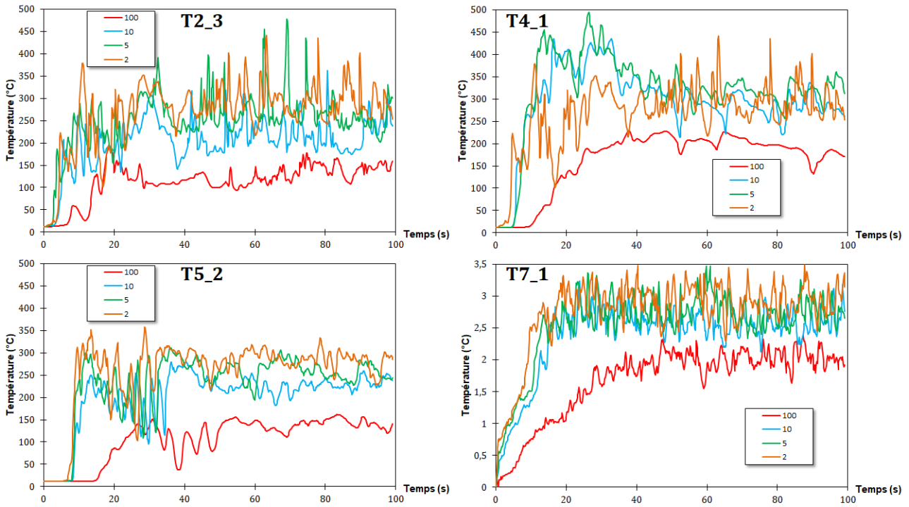
Figure 3.17 – Comparaison des champs de température aux points T2_3, T4_1 et T5_2 ainsi que de la vitesse en T7_1 pour 4 fréquences de résolution (2, 5, 10 et 100).
