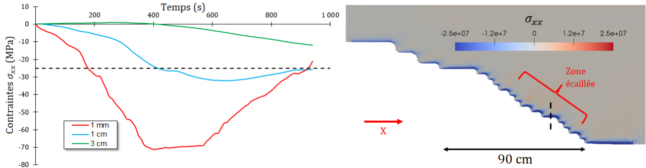
Figure 4.44 – Contraintes mécaniques issues de la simulation de la combustion d'un foyer de 20 kg de bois. a - Courbes temporelles des contraintes mécaniques \sigma_{xx} à plusieurs profondeurs dans la roche (la droite en pointillé correspond à la résistance en compression à 20°C). La localisation verticale des points où les contraintes sont calculées est indiquée par la ligne en pointillé sur la figure b. b - Champ de contrainte \sigma_{xx} 460 secondes après l'allumage dans le plan de coupe orthogonal à l'axe de la galerie et passant par le centre du foyer.
