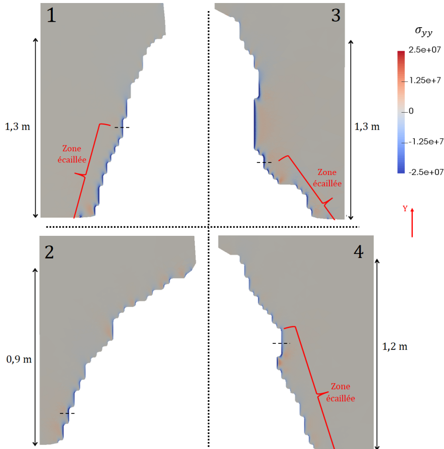
Figure 4.62 – Champ de contrainte \sigma_{yy} 470 secondes après l’allumage d’un feu de 25 kg de bois. Le numéro des coupes correspond à celles présentées sur la figure 4.61.
