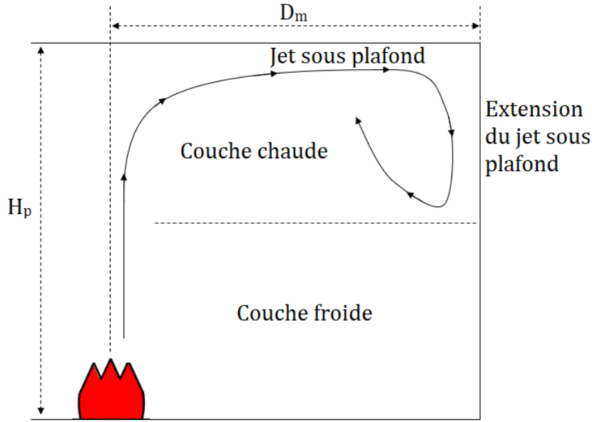
Figure 1.13 – Schématisation de l'extension du jet sous plafond aux parois verticales.
