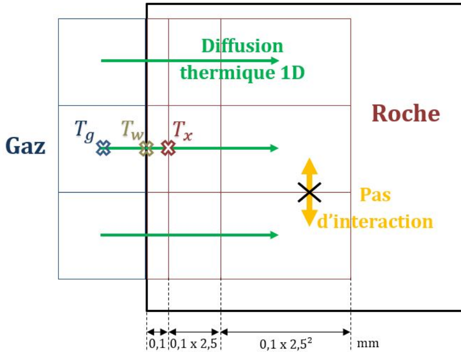
Figure 2.1 – Description schématique de la condition limite. La taille des cellules n'est pas à l'échelle.
