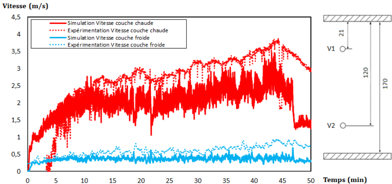
Figure 3.30 – Vitesses des gaz simulées et mesurées par les deux capteurs positionnés sur l'arbre T7.
