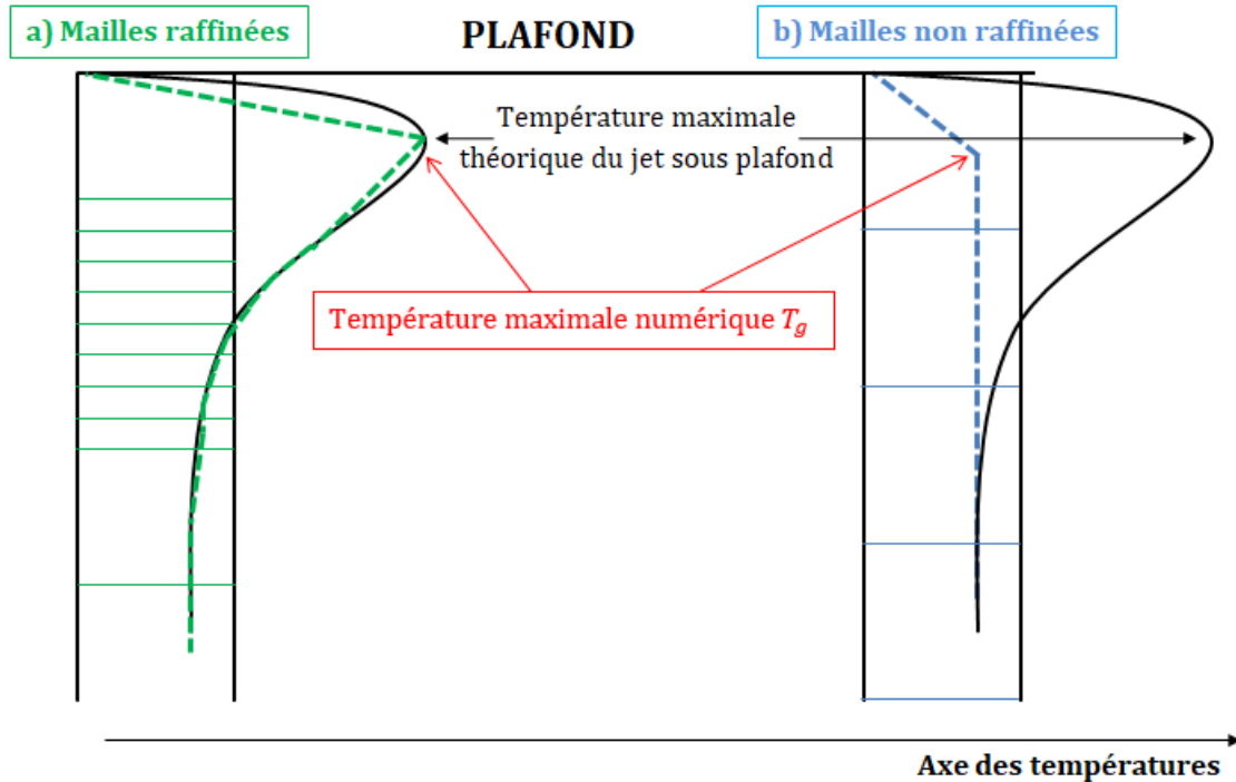
Figure 2.15 – Le profil de température réel est schématisé par les courbes noires. a) Profil numérique de la température du jet sous plafond pour un maillage raffiné sous la première cellule (en vert). b) Profil numérique de la température du jet sous plafond pour un maillage non raffiné (en bleu).
