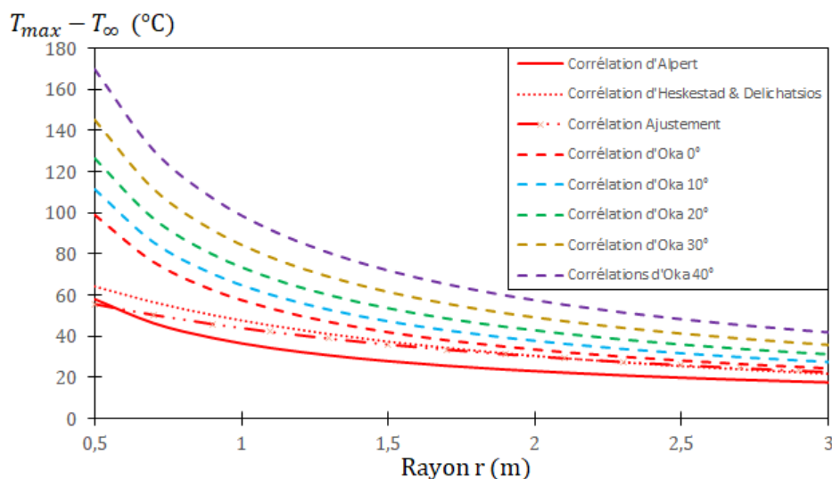
Figure 1.12 – Comparaison entre les différentes corrélations des températures maximum du jet sous plafond pour H_p = 2,5 \text{ m} et \dot{Q}_c = 70 \text{ kW} . La corrélation d’Oka (1.3.17) est tracée pour différents angles.
