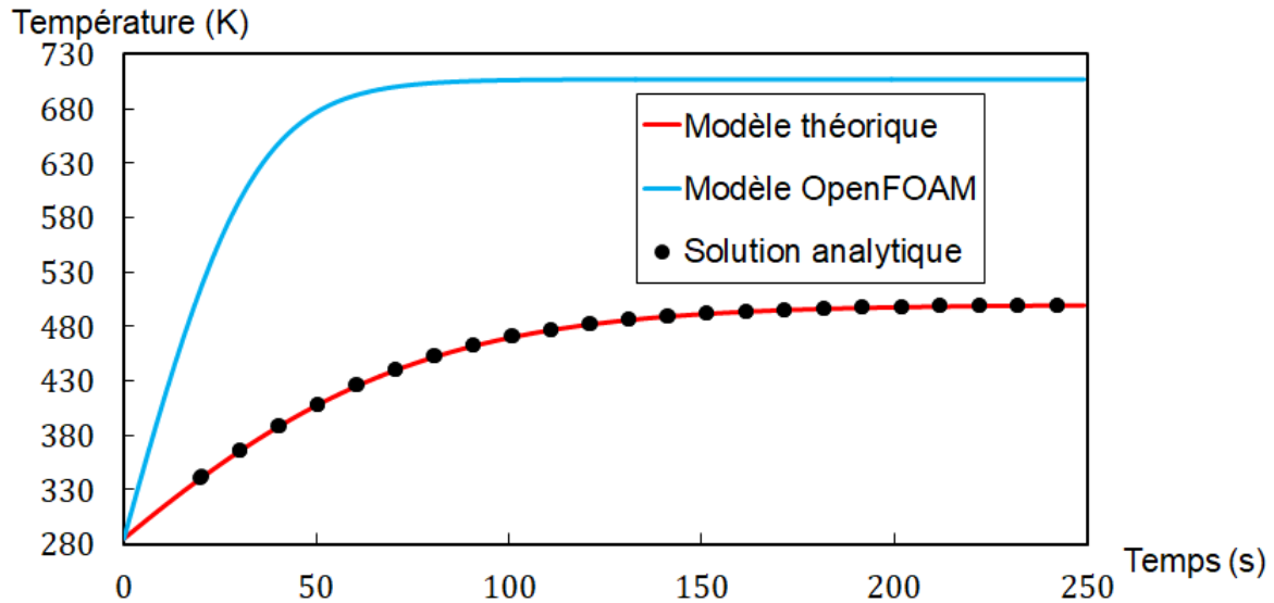
Figure 2.4 – Évolution de la température d’un thermocouple calculée par le modèle théorique (2.1.16), le modèle implémenté dans OpenFOAM [7] (2.1.17) et la solution analytique du cas test.
