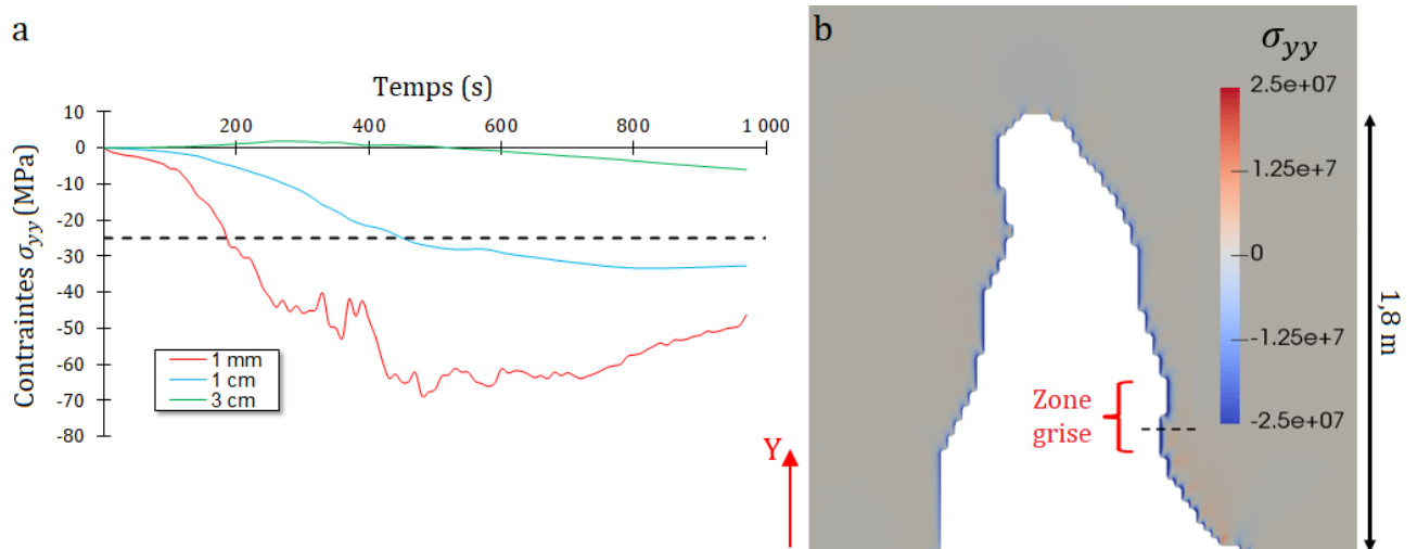
Figure 4.35 – Contraintes mécaniques issues de la simulation de la combustion d’un foyer de 25 kg de bois. a - Courbes temporelles des contraintes mécaniques \sigma_{yy} à plusieurs profondeurs dans la roche (la droite en pointillé correspond à la résistance en compression à 20^{\circ}C ). La localisation verticale des points où les contraintes sont calculées est indiquée par la ligne en pointillé sur la figure b. b - Champ de contrainte \sigma_{yy} 470 secondes après l’allumage dans le plan de coupe orthogonal à l’axe de la galerie et passant par le centre du foyer.
