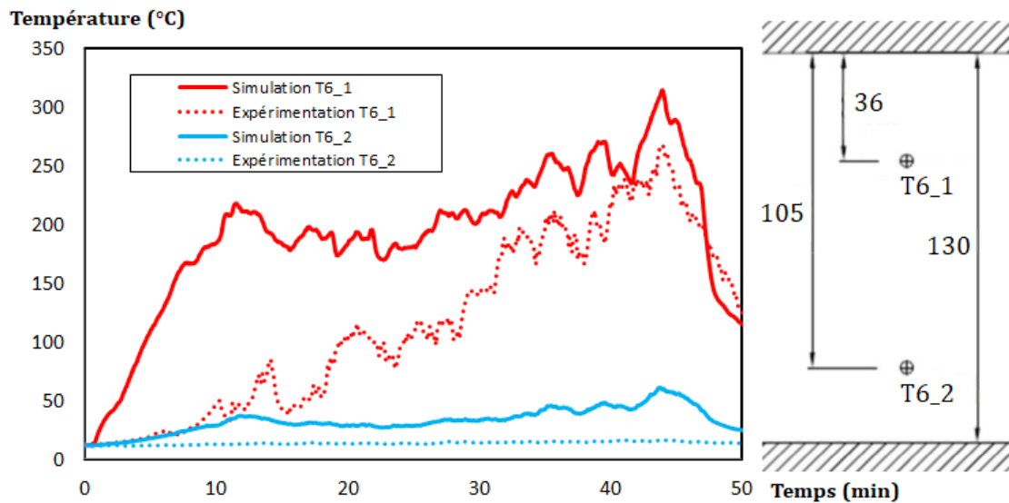
Figure 3.25 – Températures simulées et mesurées par les thermocouples de l'arbre T6. La localisation des thermocouples est indiquée à droite.
