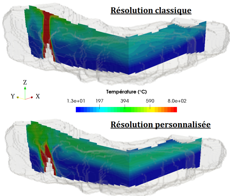
Figure 2.23 – Comparaison des champs de température dans les sections médianes des deux galeries de la carrière à la fin de la simulation (100 s).
