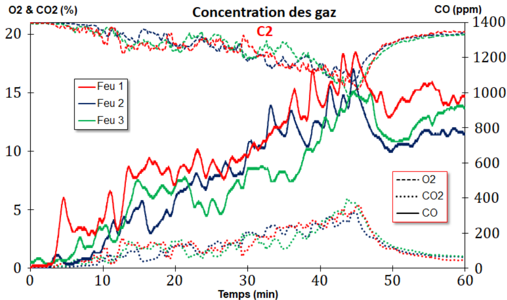
Figure 3.7 – Comparaison des mesures des concentrations de gaz effectuées en C2 pour les trois feux.
