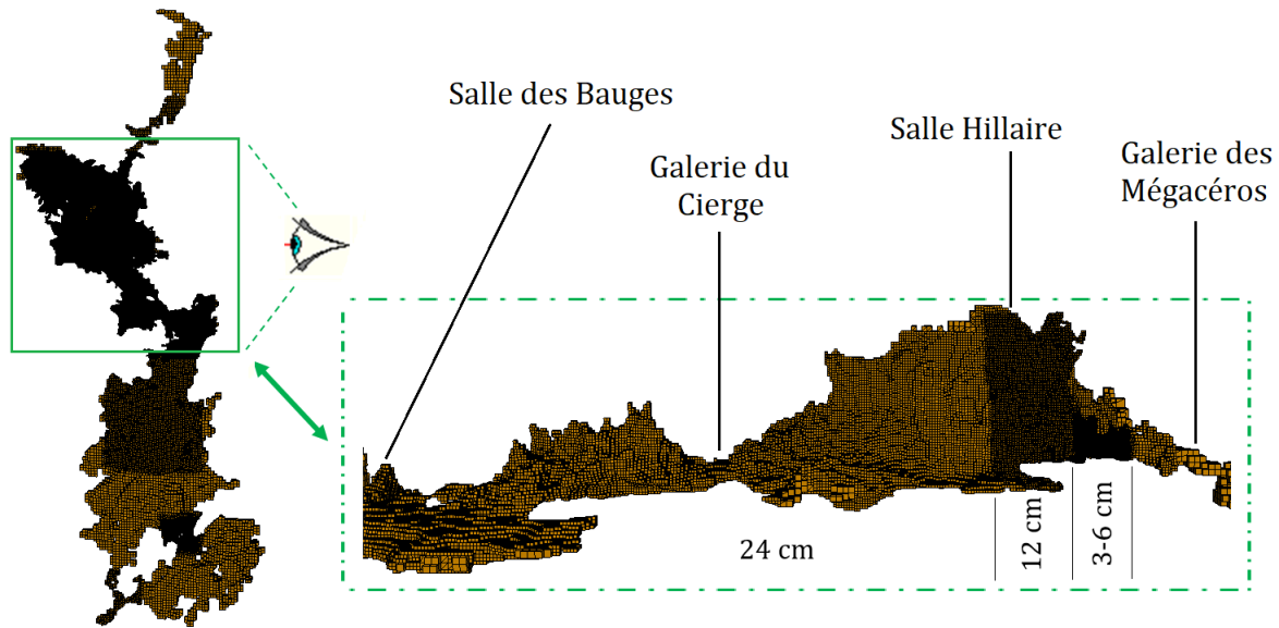
Figure 4.84 – Maillage raffiné de la grotte Chauvet-Pont d'Arc constitué d'environ 1 million de mailles. La géométrie dans le carré vert correspond au maillage vu de côté.
