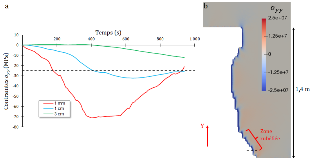
Figure 4.51 – Contraintes mécaniques issues de la simulation de la combustion d’un foyer de 10 kg de bois. a - Courbes temporelles des contraintes mécaniques \sigma_{yy} à plusieurs profondeurs dans la roche (la droite en pointillé correspond à la résistance en compression à 20^{\circ}C ). La localisation verticale des points où les contraintes sont calculées est indiquée par la ligne en pointillé sur la figure b. b - Champ de contrainte \sigma_{yy} 460 secondes après l’allumage dans le plan de coupe orthogonal à l’axe de la galerie et passant par le centre du foyer.
