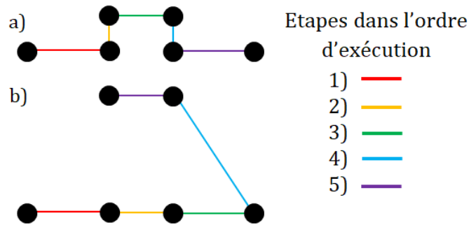
Figure E.3 – La géométrie réelle correspond à un créneau. a) Cas présentant un succès de la méthode. b) Cas présentant un échec de la méthode.
