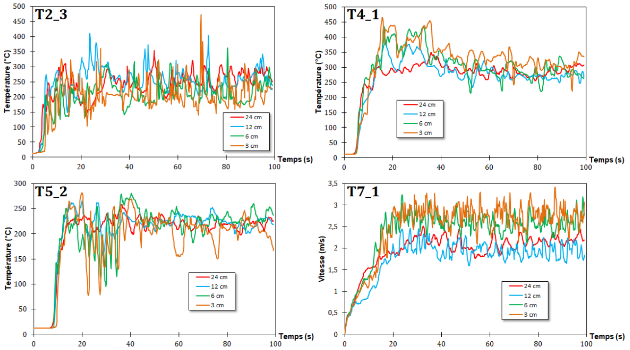
Figure 3.10 – Comparaison des champs de température aux points T2_3, T4_1 et T5_2 ainsi que de la vitesse en T7_1 pour 4 maillages (3 cm, 6 cm, 12 cm et 24 cm).
