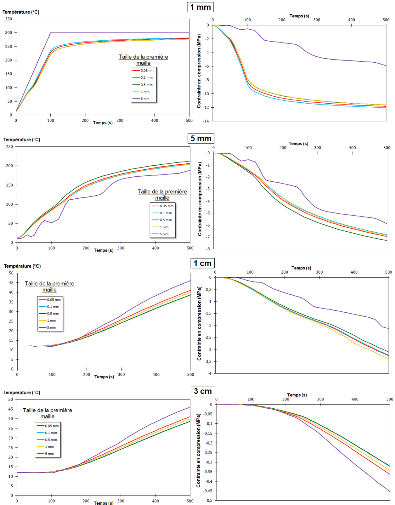
Figure 3.13 – Comparaison des températures et des contraintes en compression à différentes profondeurs pour plusieurs discrétisations. La première colonne correspond aux températures et la seconde aux contraintes. Chaque ligne est associée à une profondeur : 1 mm pour la première, 5 mm pour la deuxième, 1 cm pour la troisième et 3 cm pour la dernière.
