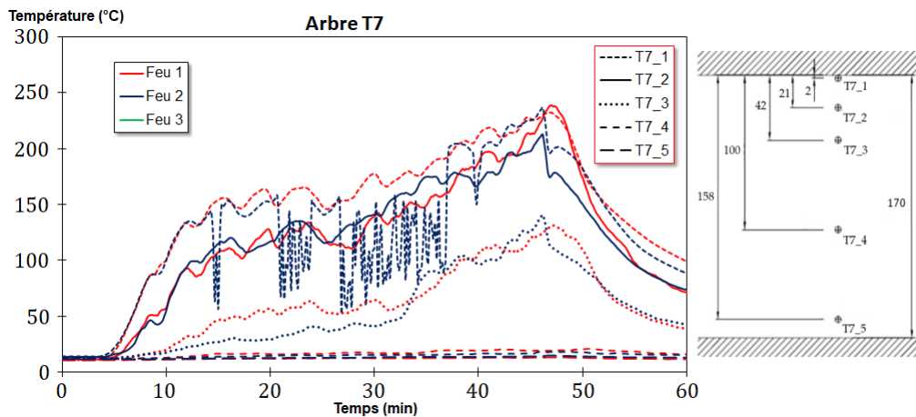
Figure F.2.7 – Mesures de température effectuées par les thermocouples de l’arbre T7. La localisation verticale des thermocouples est indiquée en cm.
