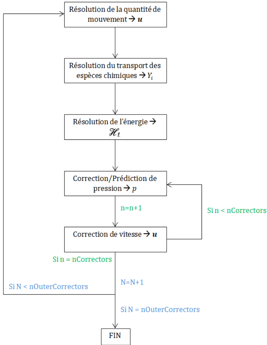
Figure 1.29 – Schéma de l’algorithme PIMPLE.
