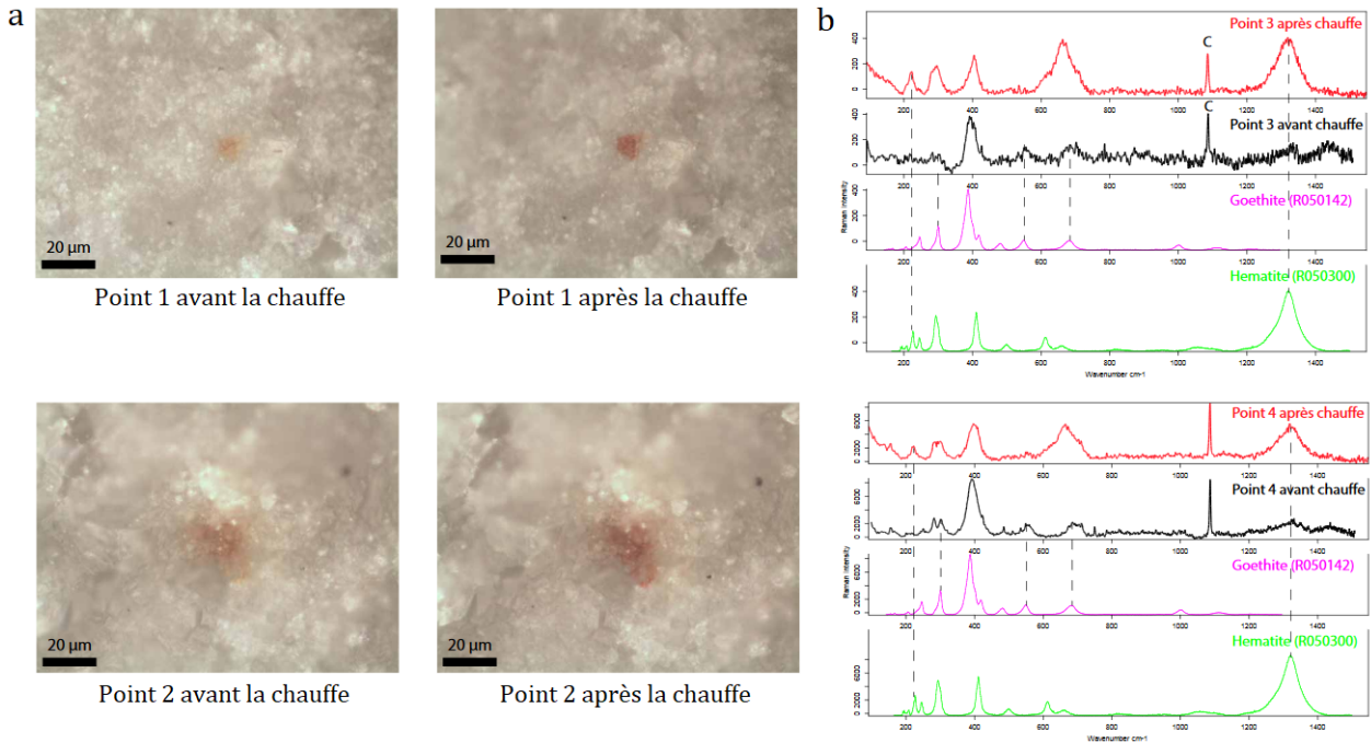
Figure 1.20 – a - Observation des points étudiés avant et après une chauffe de 250^\circ C pendant 45 minutes dans un four électrique à rayonnement. La consigne est basée sur la température de surface des échantillons. b - Intensité des spectres Raman avant et après la chauffe pour les deux points étudiés. Ces spectres sont comparés avec ceux de la goethite et de l'hématite. Essai effectué par C. Ferrier, A. Queffelec et J.-C. Mindeguia.
