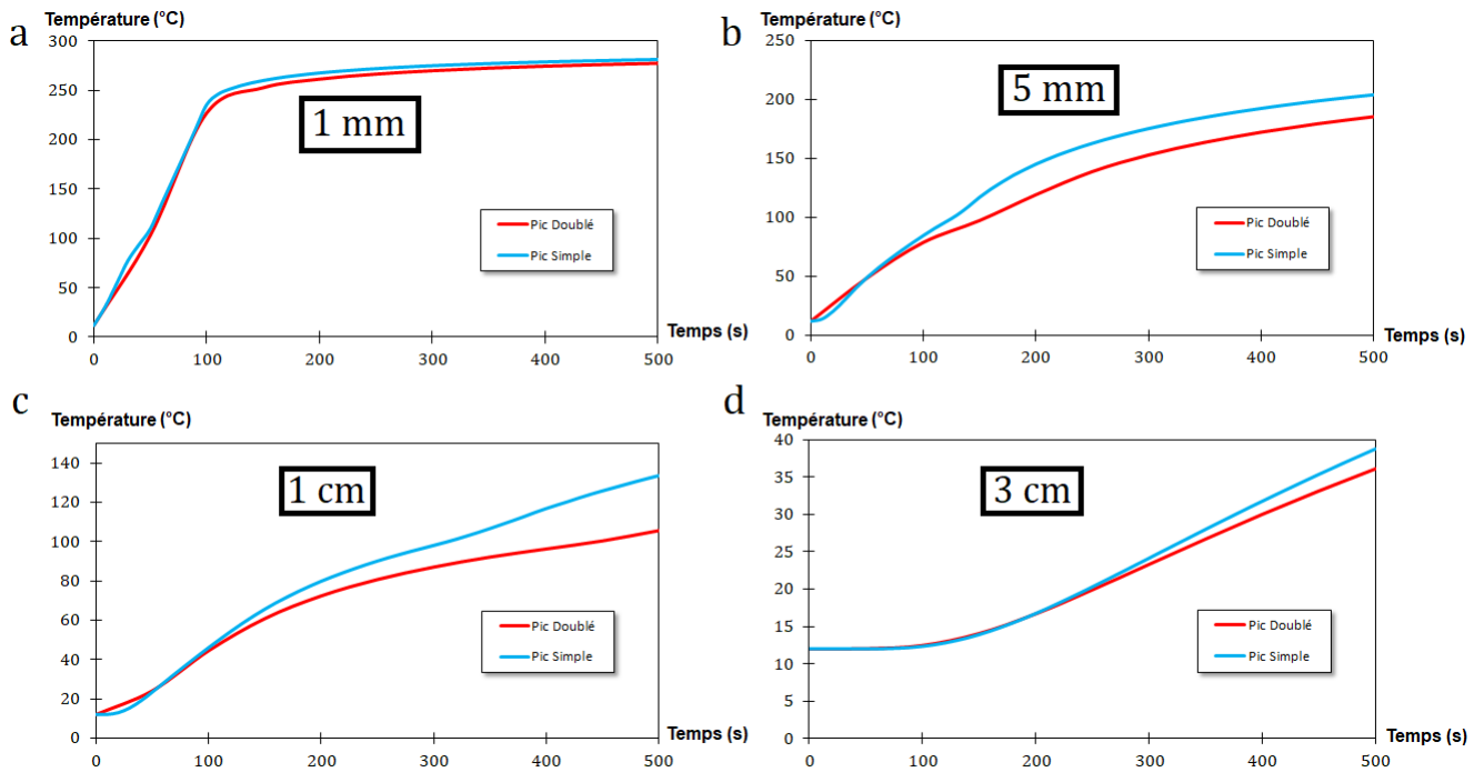
Figure 4.6 – Comparaison des températures simulées avec une capacité thermique prenant en compte le pic théorique et le pic doublé par rapport à la théorie. a - Comparaison à 1 mm de profondeur. b - Comparaison à 5 mm de profondeur. c - Comparaison à 1 cm de profondeur. d - Comparaison à 3 cm de profondeur.
