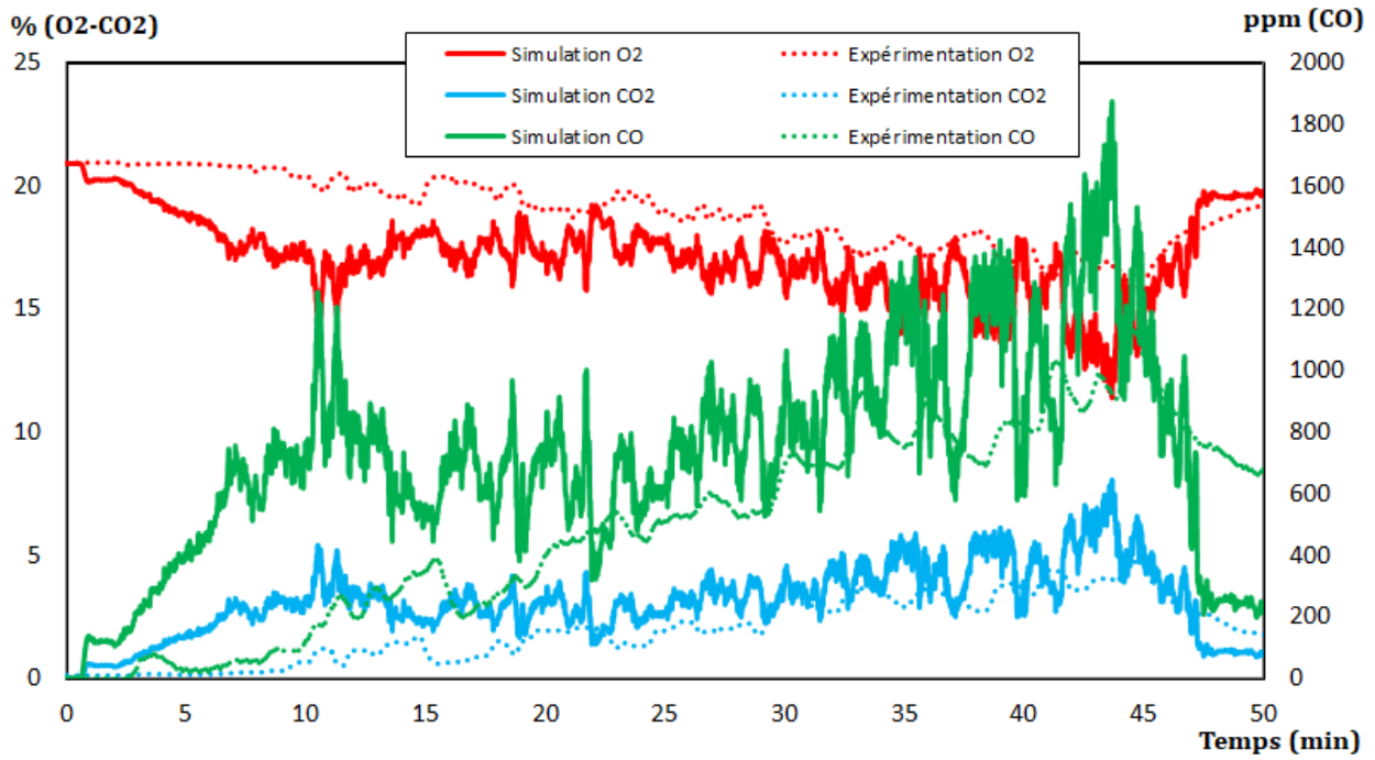
Figure 3.28 – Concentrations simulées et mesurées par les capteurs en C2.
