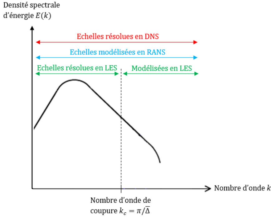
Figure 1.16 – Comparaison des approches de résolution de la turbulence.
