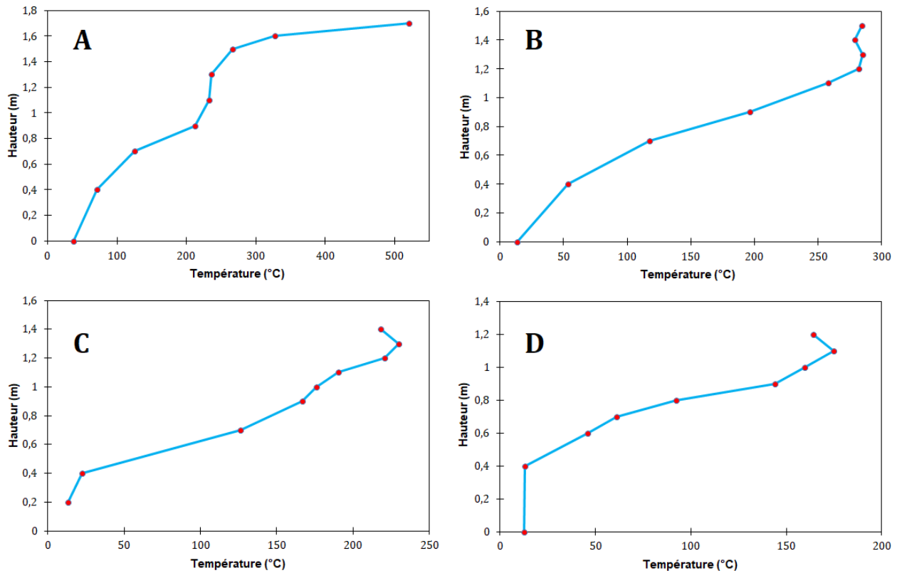
Figure 2.19 – A - Profil de température simulée le long de l’arbre A. B - Profil de température simulée le long de l’arbre B. C - Profil de température simulée le long de l’arbre C. D - Profil de température simulée le long de l’arbre D.
