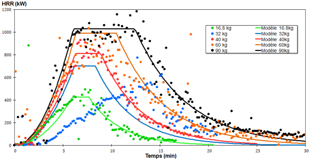
Figure 4.11 – Comparaison expérimentale des HRR pour différentes masses initiales. Les points correspondent aux mesures tandis que les courbes pleines correspondent aux résultats du modèle des wood cribs adapté à ce type de foyer.
