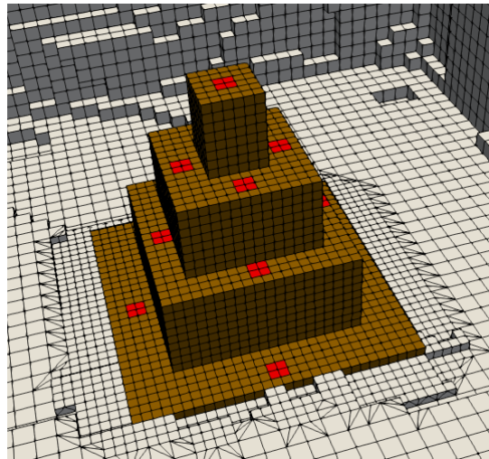
Figure 3.18 – Maillage du foyer au fond de la seconde galerie. Les brûleurs (en rouge) sont parsemés sur toute la surface du foyer (en marron).
