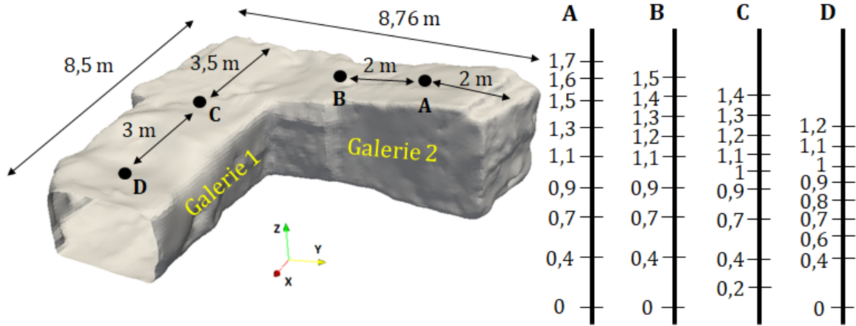
Figure 2.18 – Position des points de comparaison pour le cas test. La figure de gauche indique la localisation spatiale des arbres de points verticaux et la figure de droite détaille la disposition verticale des points de chaque arbre. Les arbres sont systématiquement placés au centre des galeries.
