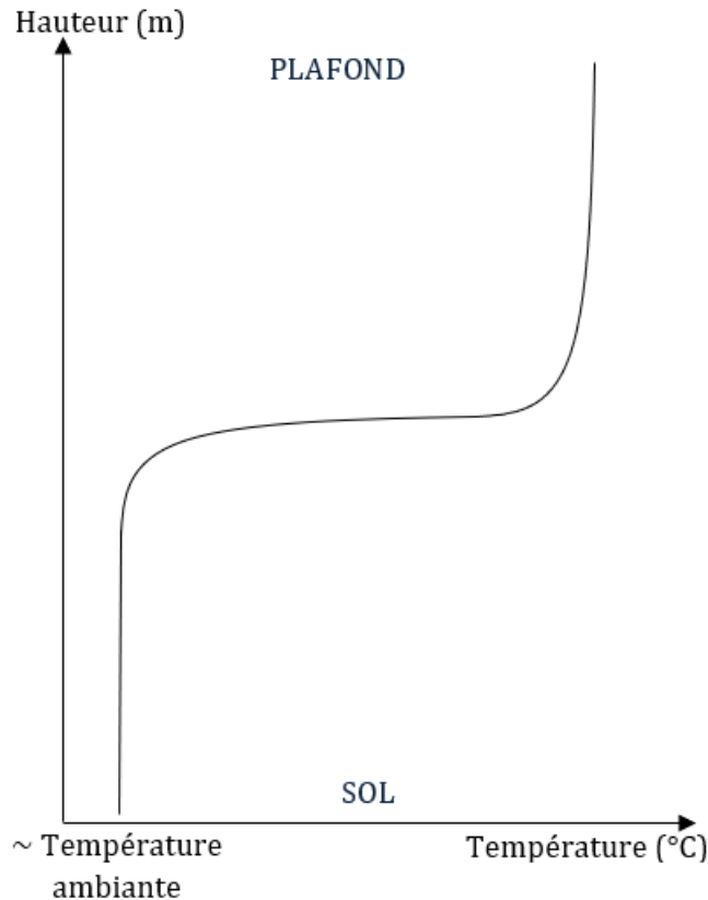
Figure 2.17 – Profil de température typique lors de l'établissement de deux couches de températures distinctes : une couche chaude de température homogène et une couche froide de température presque identique à l'air ambiant.
