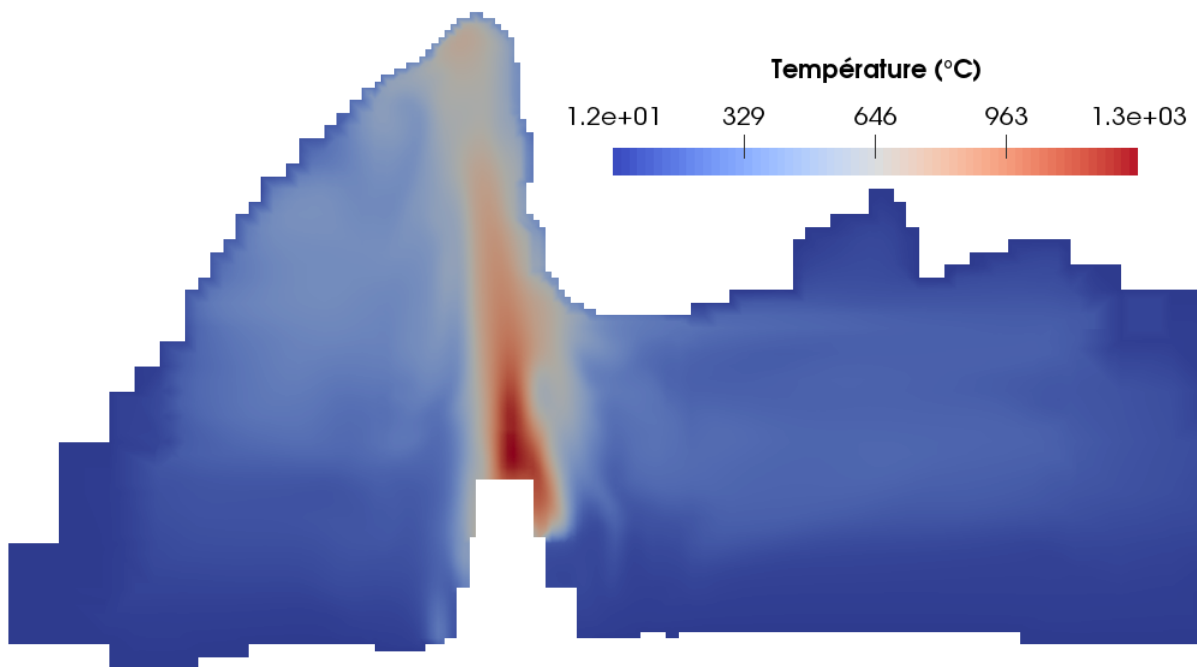
Figure 4.67 – Champ de température dans le plan orthogonal à l'axe de la galerie et passant par le centre du foyer 460 s après l'allumage d'un foyer de 15 kg de bois.
