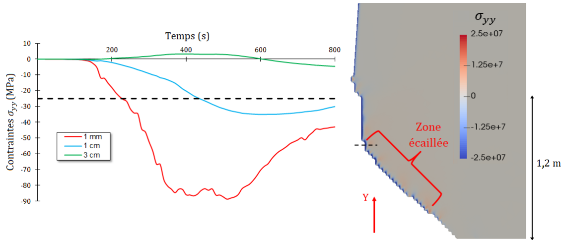
Figure 4.82 – Contraintes mécaniques issues de la simulation de la combustion d’un foyer de 10 kg de bois. a - Courbes temporelles des contraintes mécaniques \sigma_{yy} à plusieurs profondeurs dans la roche (la droite en pointillé correspond à la résistance en compression à 20^{\circ}\text{C} ). La localisation verticale des points où les contraintes sont calculées est indiquée par la ligne en pointillé sur la figure b. b - Champ de contrainte \sigma_{yy} 460 secondes après l’allumage dans le plan de coupe orthogonal à la galerie et passant par le centre du foyer.
