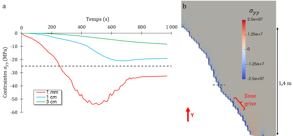
Figure 4.24 – Contraintes mécaniques issues de la simulation de la combustion d’un foyer de 20 kg de bois. a - Courbes temporelles des contraintes \sigma_{yy} à plusieurs profondeurs dans la roche (la droite en pointillé correspond à la résistance en compression du calcaire urgonien à 20°C). La localisation verticale des points où les contraintes sont calculées est indiquée par la ligne en pointillé sur la figure b. b - Champ de contrainte \sigma_{yy} 460 secondes après l’allumage dans le plan de coupe orthogonal à l’axe de la galerie et passant par le centre du foyer.
