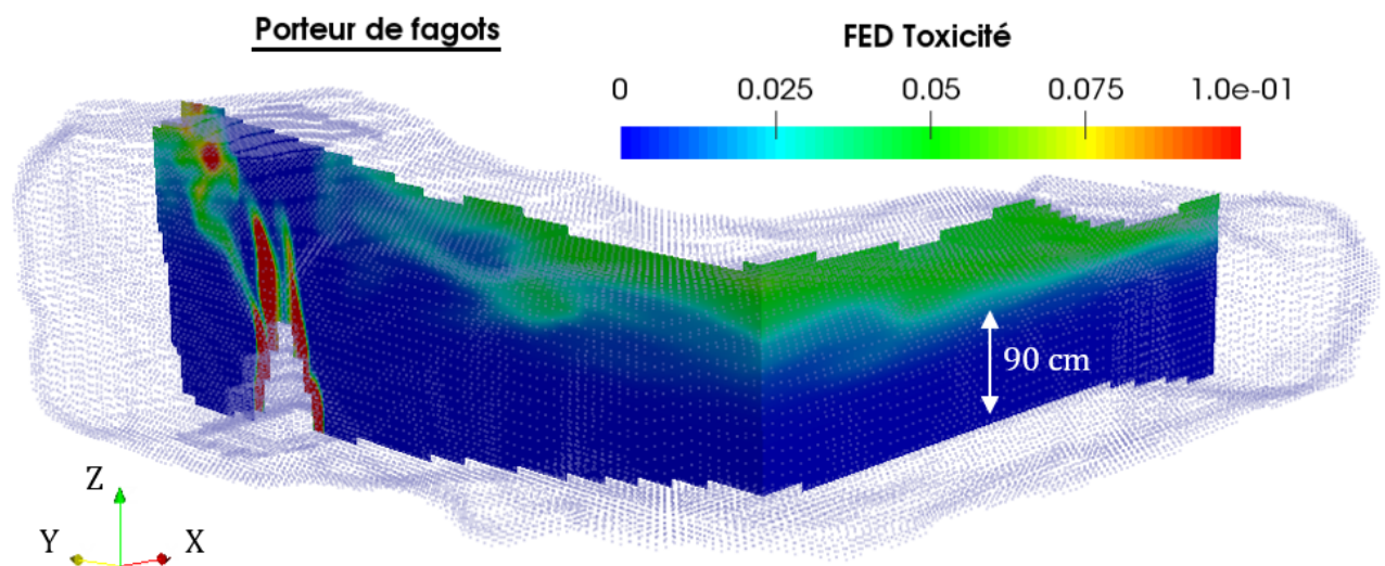
Figure 3.41 – FED relative à la toxicité pour un porteur alimentant le foyer 43 minutes après l'allumage.
