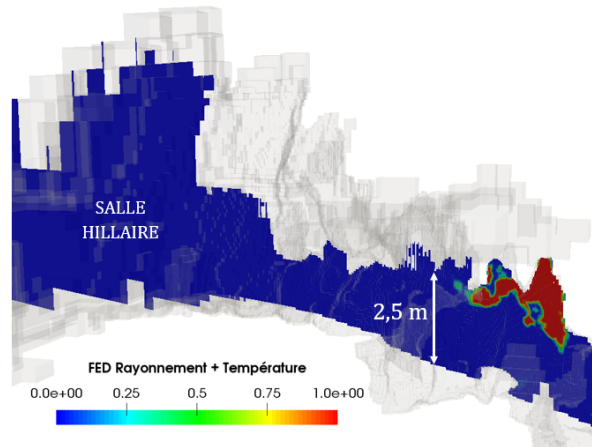
Figure 4.60 – Coupe transversale de la Galerie des Mégacéros correspondant à la FED relative au rayonnement et à la température pour une personne alimentant le foyer 19 minutes après l’allumage dans le cadre du protocole C.
