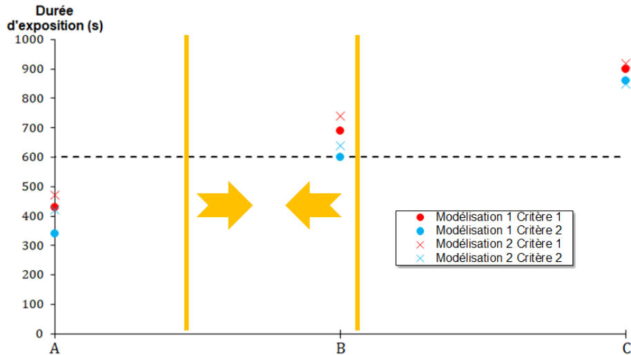
Figure 4.32 – Durée d'exposition de la surface altérée aux températures correspondant aux critères de rubéfaction dans la zone 2 en fonction du protocole considéré. La ligne en pointillé correspond à la durée pour laquelle il y a reproduction des thermo-altérations observables in situ .
