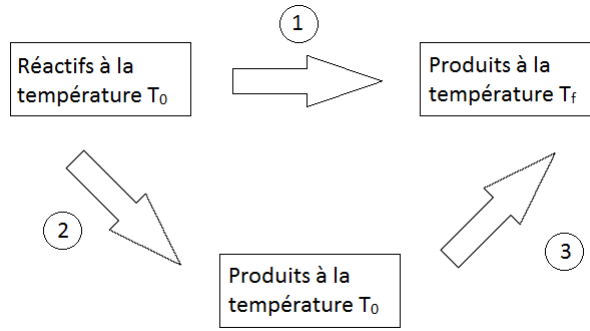
Figure 1.8 – Chemins thermodynamiques réel ① et fictif ② + ③.
