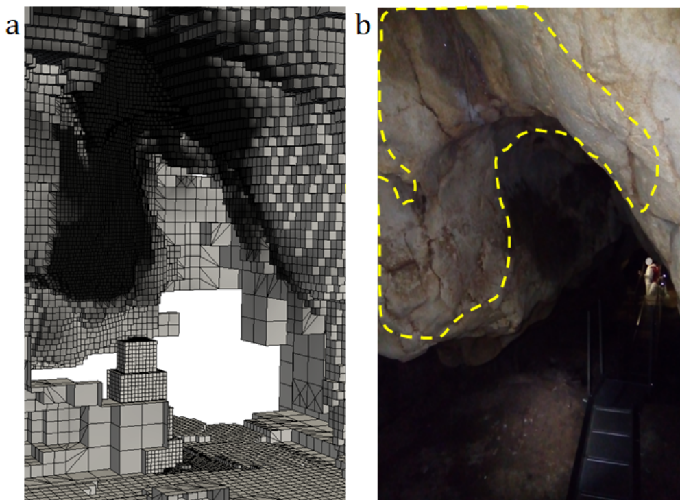
Figure 4.74 – a - Dépôt de suie simulé dans la géométrie numérique de la grotte Chauvet-Pont d'Arc pour un feu de 15 kg de bois dans la zone 6. b - Dépôt de suie numérique issu de la simulation (délimité en jaune) transposé dans la Galerie des Mégacéros (extrait de la photogrammétrie réalisée par T. Sagory / Équipe grotte Chauvet - MC).
