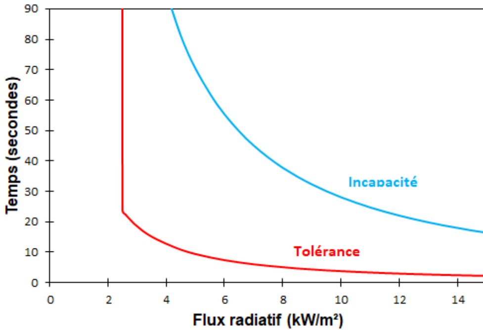
Figure 2.6 – Temps de tolérance et d'incapacité (2.1.30) sous un rayonnement q_r .
