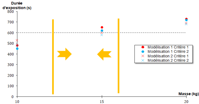
Figure 4.78 – Durée d'exposition de la surface altérée aux températures correspondant aux critères de rubéfaction dans la zone 7 en fonction de la masse du foyer considéré. La ligne en pointillé correspond à la durée pour laquelle il y a reproduction des thermo-altérations observables in situ .
