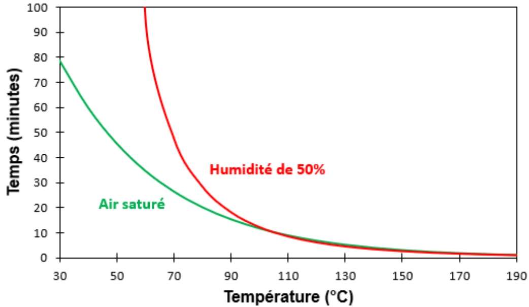
Figure 2.8 – Temps de tolérance en air saturé (2.1.33) et non saturé (2.1.32) sous une température T .
