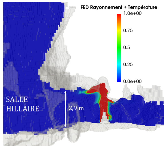
Figure 4.34 – FED relative au rayonnement et à la température pour une personne alimentant le foyer 10 minutes après l’allumage, dans le cadre du protocole C.
