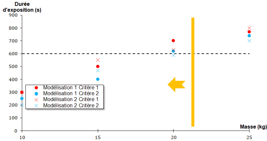
Figure 4.19 – Durée d'exposition de la surface altérée aux températures correspondant aux critères de rubéfaction dans la zone 1 en fonction de la masse du foyer considéré. La ligne en pointillé correspond à la durée pour laquelle il y a reproduction des thermo-altérations observables in situ .
