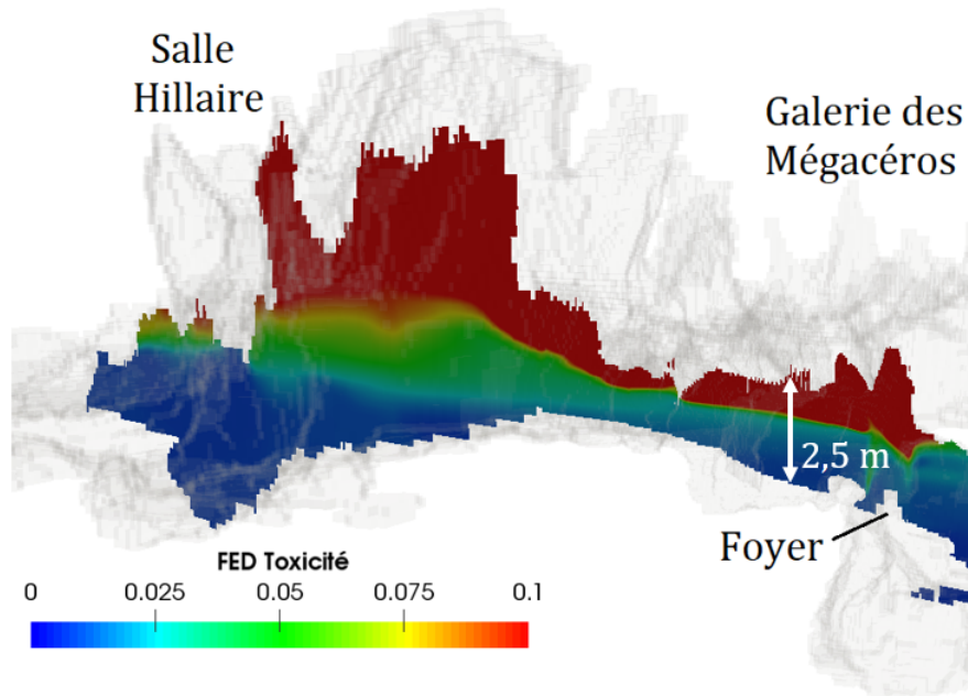
Figure 4.87 – FED relative à la toxicité pour un observateur ayant demeuré dans la Salle Hillaire pendant toute la combustion d’un foyer de 30 kg situé à l’emplacement du feu de la zone 5.
