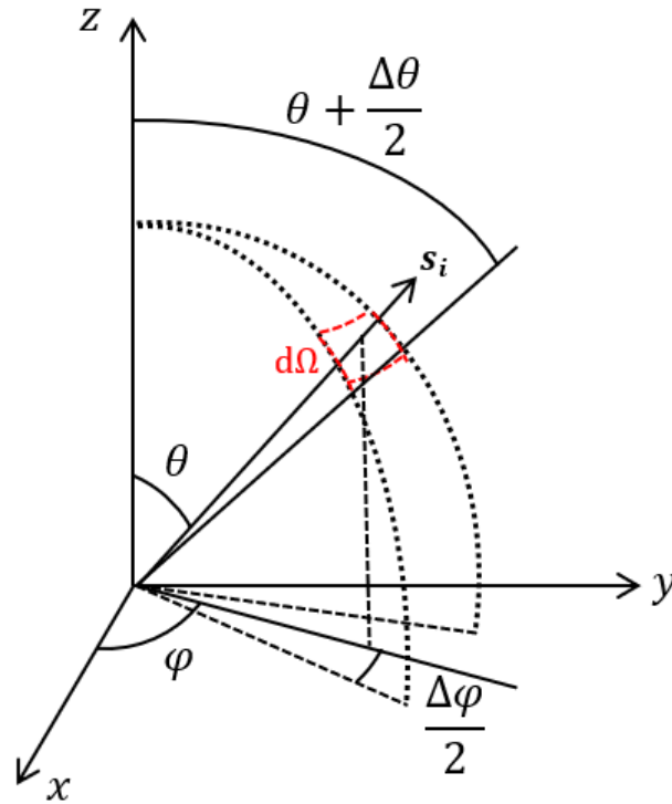
Figure 1.28 – Schématisation de l'angle solide et notations utilisées.
