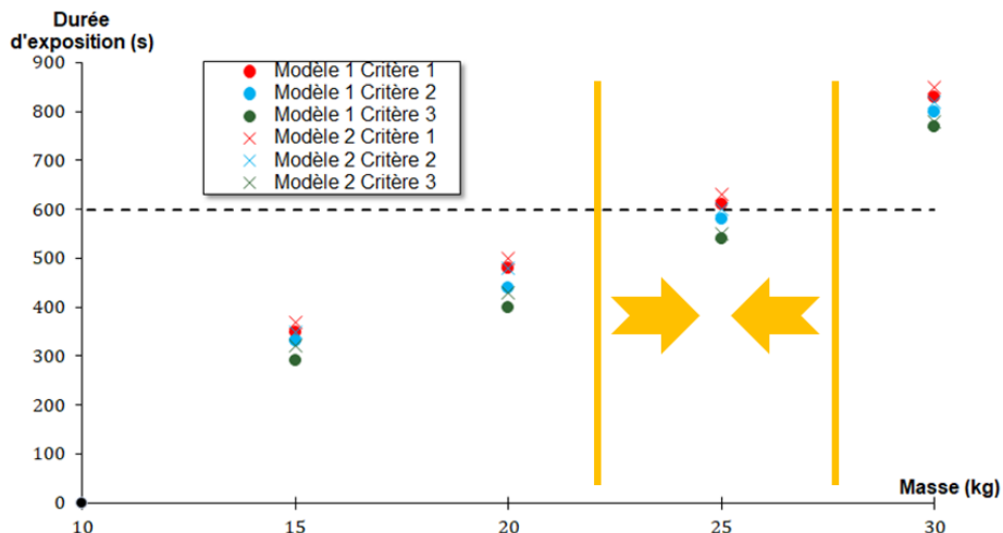
Figure 4.57 – Durée d'exposition de la surface altérée aux températures correspondant aux critères de couleur grise dans la zone 5 en fonction de la masse du foyer considéré. La ligne en pointillé correspond à la durée pour laquelle il y a reproduction des thermo-altérations observables in situ .
