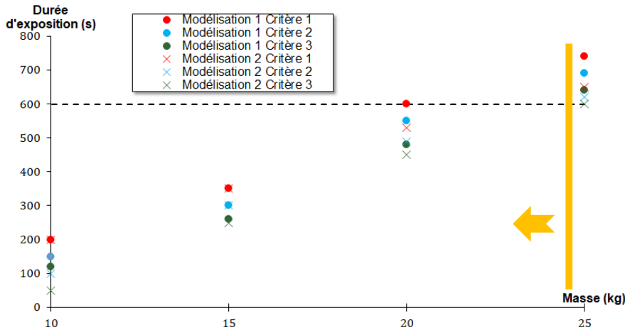
Figure 4.20 – Durée d'exposition de la surface altérée aux températures correspondant aux critères de couleur grise dans la zone 1 en fonction de la masse du foyer considéré. La ligne en pointillé correspond à la durée pour laquelle il y a reproduction des thermo-altérations observables in situ .
