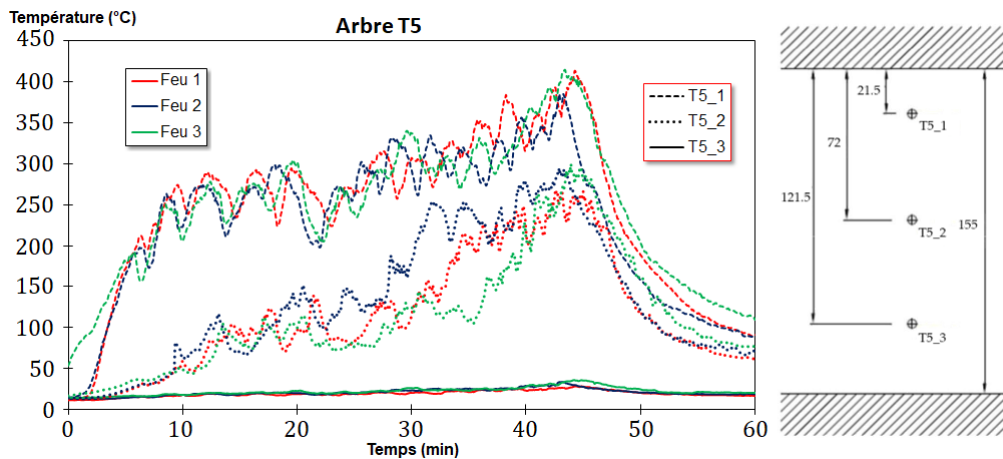
Figure F.2.5 – Mesures de température effectuées par les thermocouples de l’arbre T5. La localisation verticale des thermocouples est indiquée en cm.
