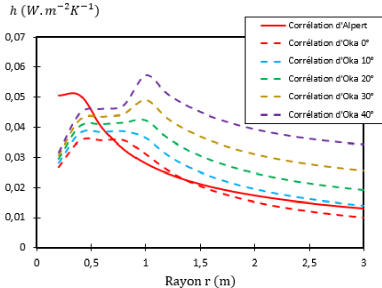
Figure 2.14 – Comparaison entre les deux corrélations du coefficient de transfert thermique pour H_p = 2,5 \text{ m} et \dot{Q}_c = 70 \text{ kW} . La corrélation d'Oka (2.3.8) est tracée pour différents angles.
