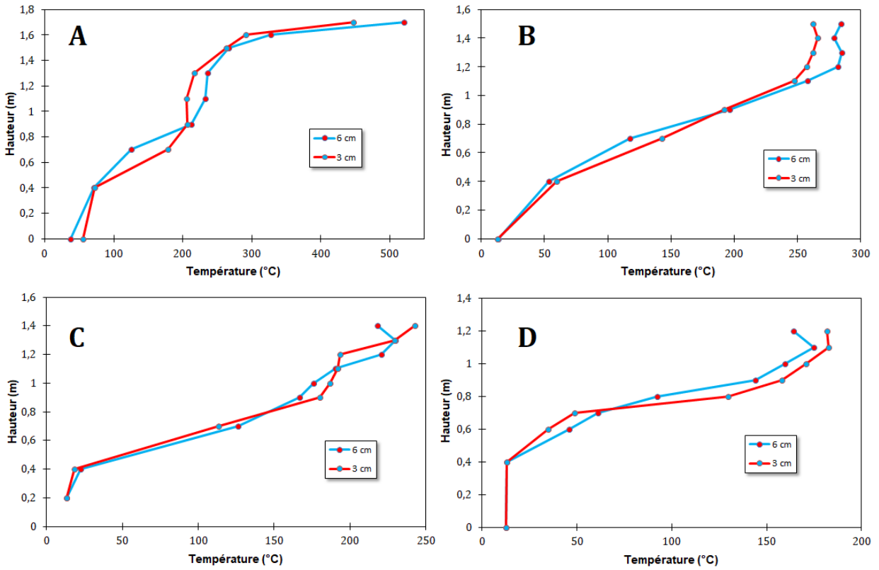
Figure 2.20 – Comparaison des profils de températures des arbres A, B, C et D pour des mailles de 3 cm et 6 cm.
