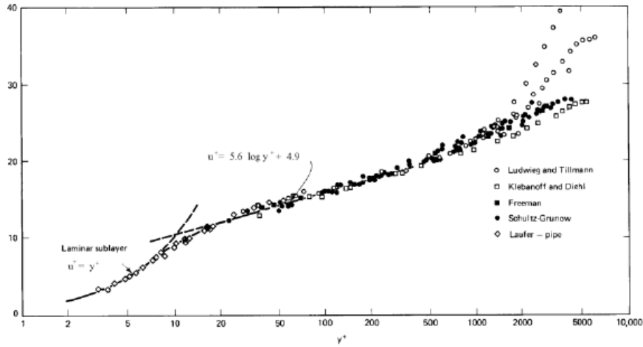
Figure 1.18 – Comparaison des lois de paroi avec des données expérimentales [5] (Clauser, 1956).
