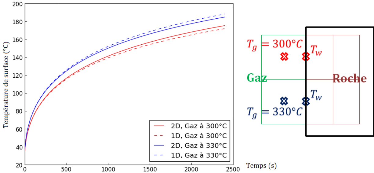
Figure 2.3 – Comparaison de la température de surface entre les résolutions 1D et 2D de la diffusion thermique lorsque les températures de deux cellules adjacentes sont 300°C et 330°C.
