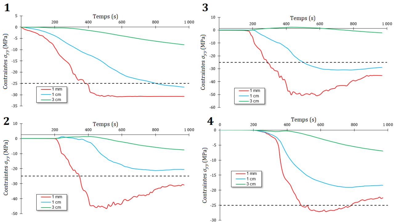
Figure 4.63 – Courbes temporelles des contraintes mécaniques \sigma_{yy} à plusieurs profondeurs dans la roche (la droite en pointillé correspond à la résistance en compression à 20^{\circ}C ). Les graphes sont associés aux numéros des plans de coupes définis sur la figure 4.61. La localisation verticale des points où les contraintes sont calculées est indiquée par les lignes en pointillé sur la figure 4.62.
