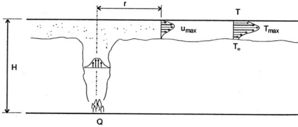
Figure 1.11 – Profils de température et de vitesse dans un jet sous plafond [4].
