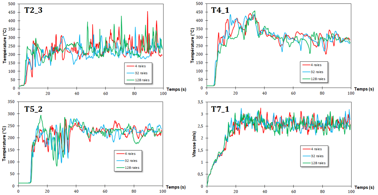
Figure 3.15 – Comparaison des champs de température aux points T2_3, T4_1 et T5_2 ainsi que de la vitesse en T7_1 pour 3 discrétisations angulaires différentes (4, 32 et 128).
