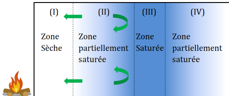
Figure 1.23 – Formation d’une couche saturée putative empêchant l’écoulement des vapeurs d’eau vers l’intérieur du massif. Le schéma représente une zone de l’ordre de quelques centimètres et les flèches vertes matérialisent la circulation des vapeurs d’eau.
