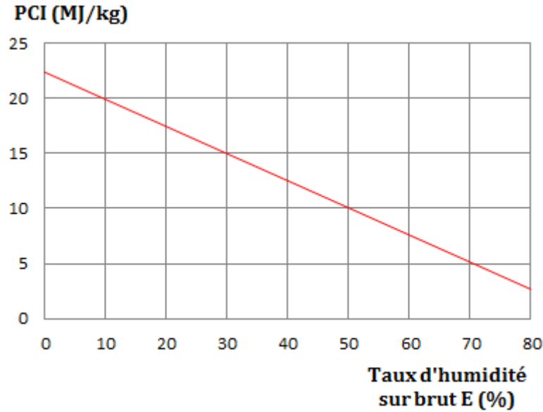
Figure 1.7 – Évolution du PCI du pin sylvestre en fonction de l'humidité.
