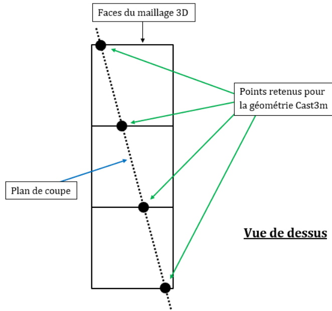
Figure 2.25 – Construction des points qui formeront le contour de la géométrie 2D utilisée par Cast3m.
