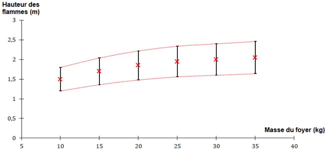
Figure 4.15 – Hauteur calculée des flammes des foyers en tipi de pin sylvestre en fonction de leur masse.
