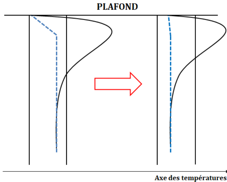
Figure 2.16 – Le profil de température réel est schématisé par les courbes noires. Les profils numériques de la température du jet sous plafond schématisé (à gauche) et plus réaliste (à droite) sont schématisés par les courbes bleues.
