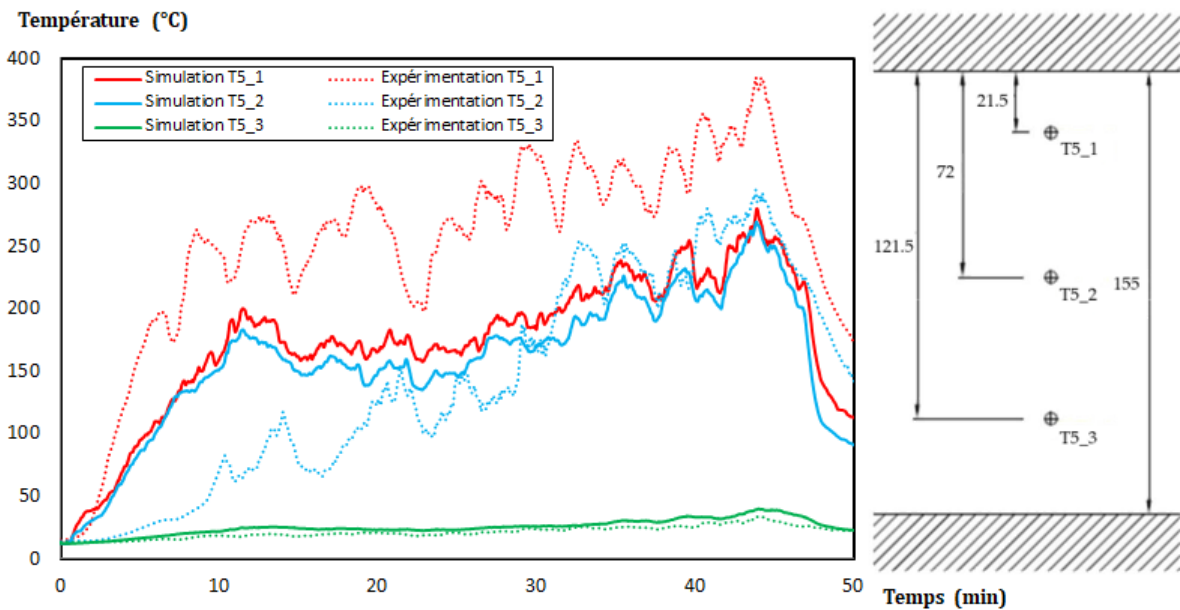
Figure 3.24 – Températures simulées et mesurées par les thermocouples de l'arbre T5. La localisation des thermocouples est indiquée à droite.
