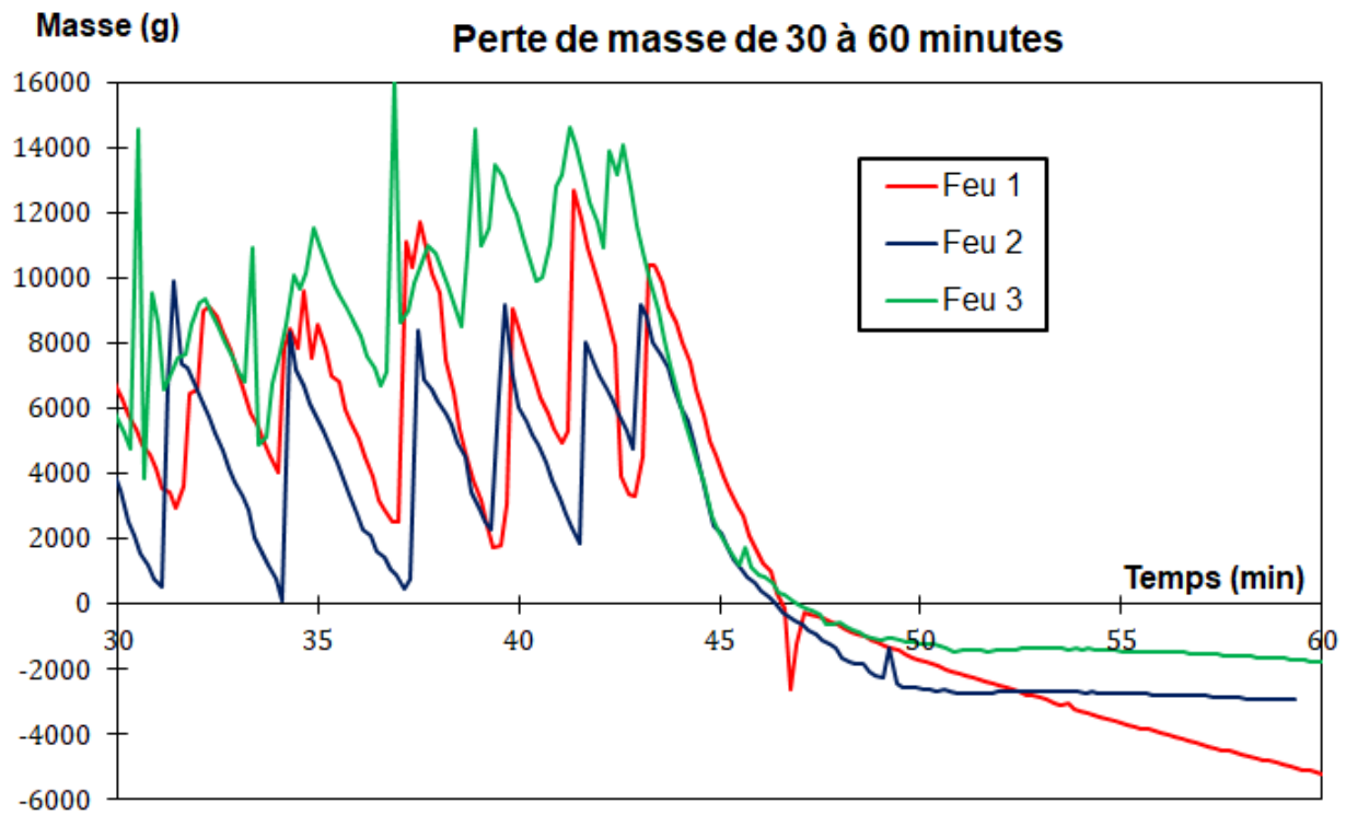
Figure F.2.14 – Perte de masse mesurée sur les 30 dernières minutes des feux.
