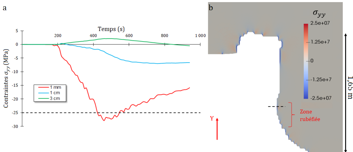
Figure 4.73 – Contraintes mécaniques issues de la simulation de la combustion d'un foyer de 15 kg de bois. a - Courbes temporelles des contraintes mécaniques \sigma_{yy} à plusieurs profondeurs dans la roche (la droite en pointillé correspond à la résistance en compression à 20^{\circ}C ). La localisation verticale des points où les contraintes sont calculées est indiquée par la ligne en pointillé sur la figure b. b - Champ de contrainte \sigma_{yy} 460 secondes après l'allumage dans le plan de coupe orthogonal à l'axe de la galerie et passant par le centre du foyer.
