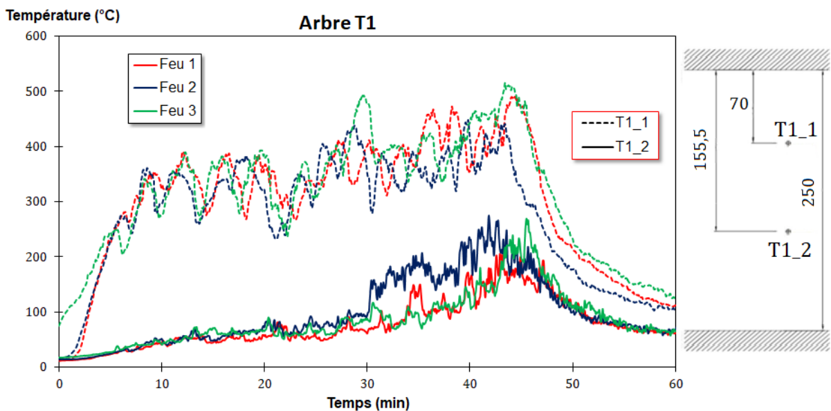
Figure 3.6 – Comparaison des mesures de température effectuées par les thermocouples de l’arbre T1 pour les trois feux. La localisation verticale des thermocouples est indiquée en cm.
