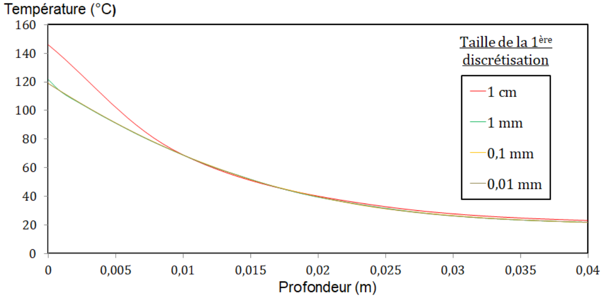
Figure 2.2 – Comparaison du profil de température pour différentes discrétisations spatiales.
