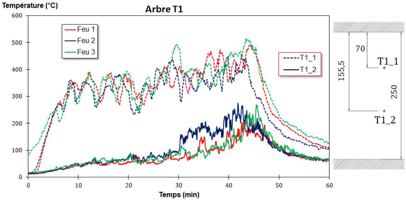
Figure F.2.1 – Mesures de température effectuées par les thermocouples de l'arbre T1. La localisation verticale des thermocouples est indiquée en cm.
