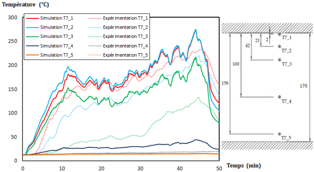
Figure 3.26 – Températures simulées et mesurées par les thermocouples de l'arbre T7. La localisation des thermocouples est indiquée à droite.
