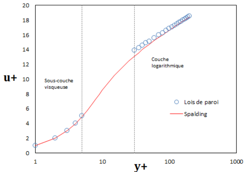
Figure 1.19 – Comparaison des lois de paroi avec la formule de Spalding (1.5.127).
