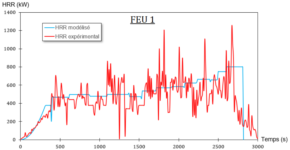
Figure 4.12 – Comparaison des HRR modélisés et expérimentaux pour le premier feu de la carrière de Lugasson.
