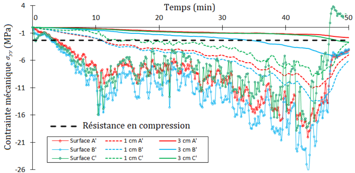
Figure 3.37 – Évolution temporelle de la contrainte mécanique \sigma_{yy} dans les parois de la carrière pour plusieurs profondeurs (surface, 1 cm et 3 cm). Les emplacements des points A', B' et C' sont définis sur la figure 3.31.
