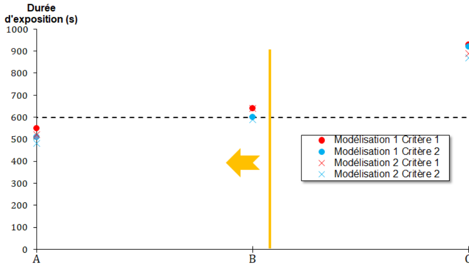
Figure 4.42 – Durée d'exposition de la surface altérée aux températures correspondant aux critères de rubéfaction dans la zone 3 en fonction du protocole considéré. La ligne en pointillé correspond à la durée pour laquelle il y a reproduction des thermo-altérations observables in situ .
