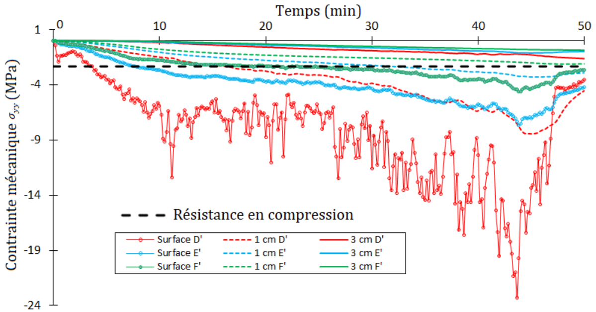
Figure 3.38 – Évolution temporelle de la contrainte mécanique \sigma_{yy} dans les parois de la carrière pour plusieurs profondeurs (surface, 1 cm et 3 cm). Les emplacements des points D', E' et F' sont définis sur la figure 3.31.
