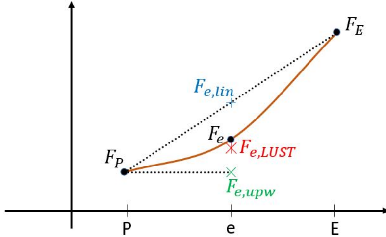
Figure 1.26 – Interpolations de la valeur de la variable au point e par les schémas linéaire, upwind et LUST.
