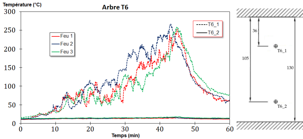
Figure F.2.6 – Mesures de température effectuées par les thermocouples de l’arbre T6. La localisation verticale des thermocouples est indiquée en cm.
