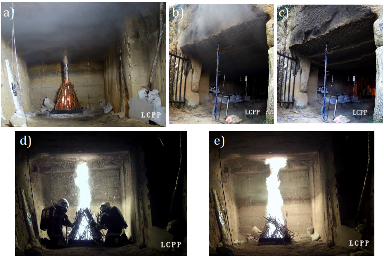
Figure 3.5 – a) Foyer composé des 4 fagots initiaux 70 s après l’allumage. b) Évacuation des fumées par l’entrée de la carrière 152 s après l’allumage. c) Absence de fumées blanches 500 s après l’allumage. d) Alimentation du foyer par les pompiers 6 min 25 s après l’allumage. e) Combustion 7 min 34 après l’allumage.
