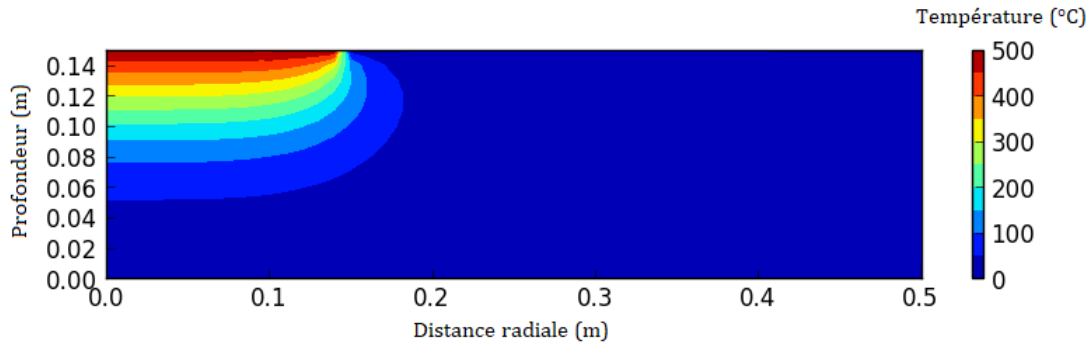
Figure 1.14 – Champ de température dans le sol à la fin du feu.
