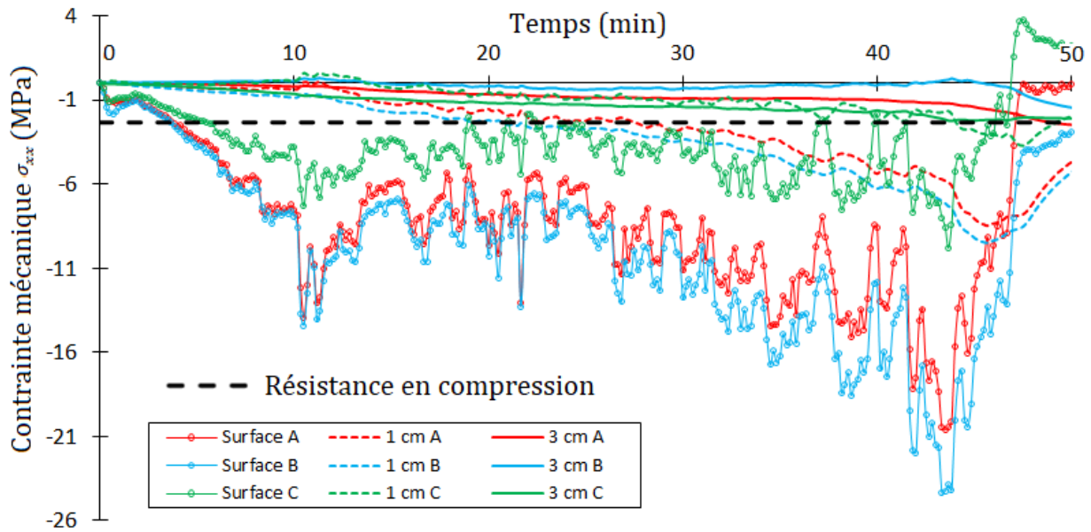
Figure 3.36 – Évolution temporelle de la contrainte mécanique \sigma_{xx} dans les parois de la carrière pour plusieurs profondeurs (surface, 1 cm et 3 cm). Les emplacements des points A, B et C sont définis sur la figure 3.31.
