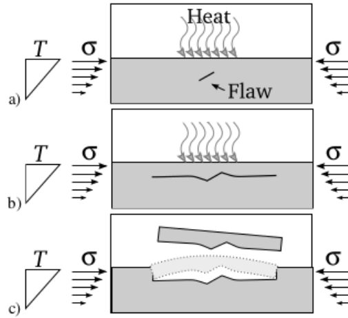
Figure 1.21 – Description schématique des étapes d’un écaillage dû à des contraintes thermo-mécaniques [6].
