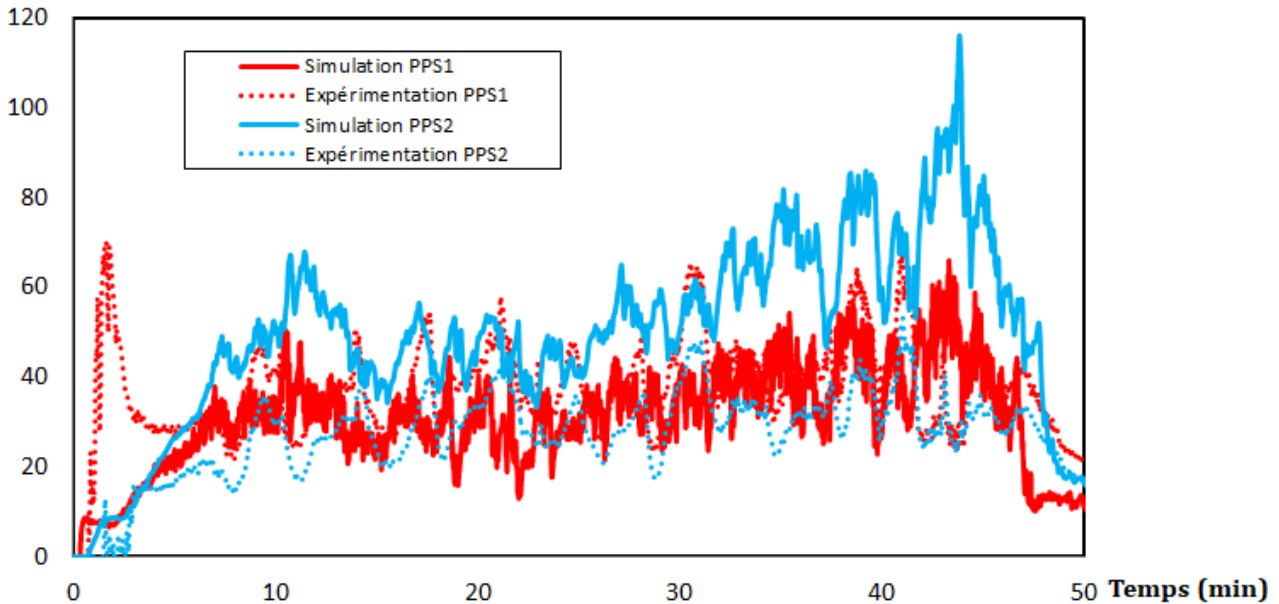
Figure 3.29 – Concentrations des suies simulées et mesurées par les capteurs en S1 et S2.
