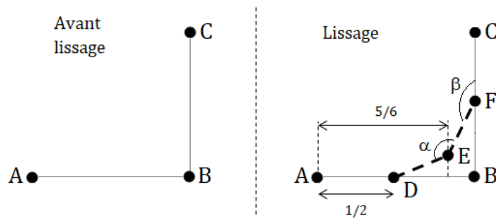
Figure 2.29 – Méthodologie décrivant le procédé de lissage des angles droits.
