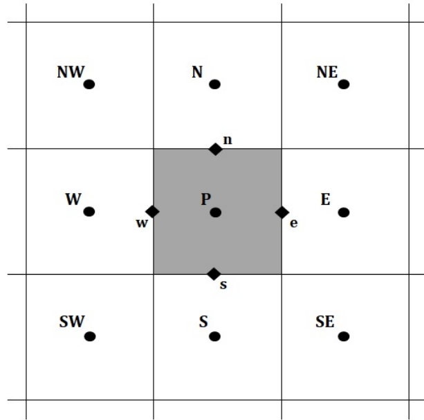
Figure 1.25 – Maillage cartésien en 2 dimensions et notations utilisées.
