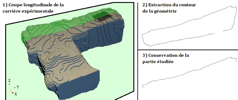
Figure 2.24 – Définition de l'intersection du plan de coupe avec la surface de la géométrie de la carrière. Seule la partie délimitée par l'utilisateur est conservée pour la suite.
