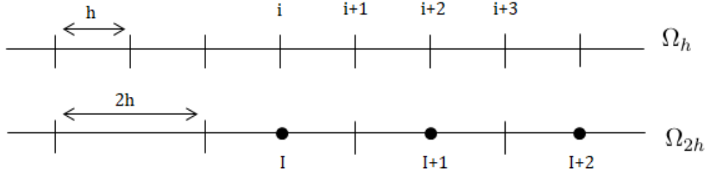
Figure 1.30 – Passage d'une grille fine de pas h à une grille grossière de pas 2h .
