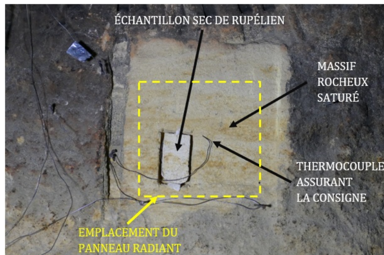
Figure 4.2 – Dispositif expérimental permettant les chauffes isochrones d'un échantillon calcaire sec déconnecté de toute arrivée d'eau et du massif saturé en eau (C. Ferrier).
