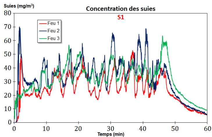
Figure F.2.10 – Mesures des concentrations en particules effectuées en S1.
