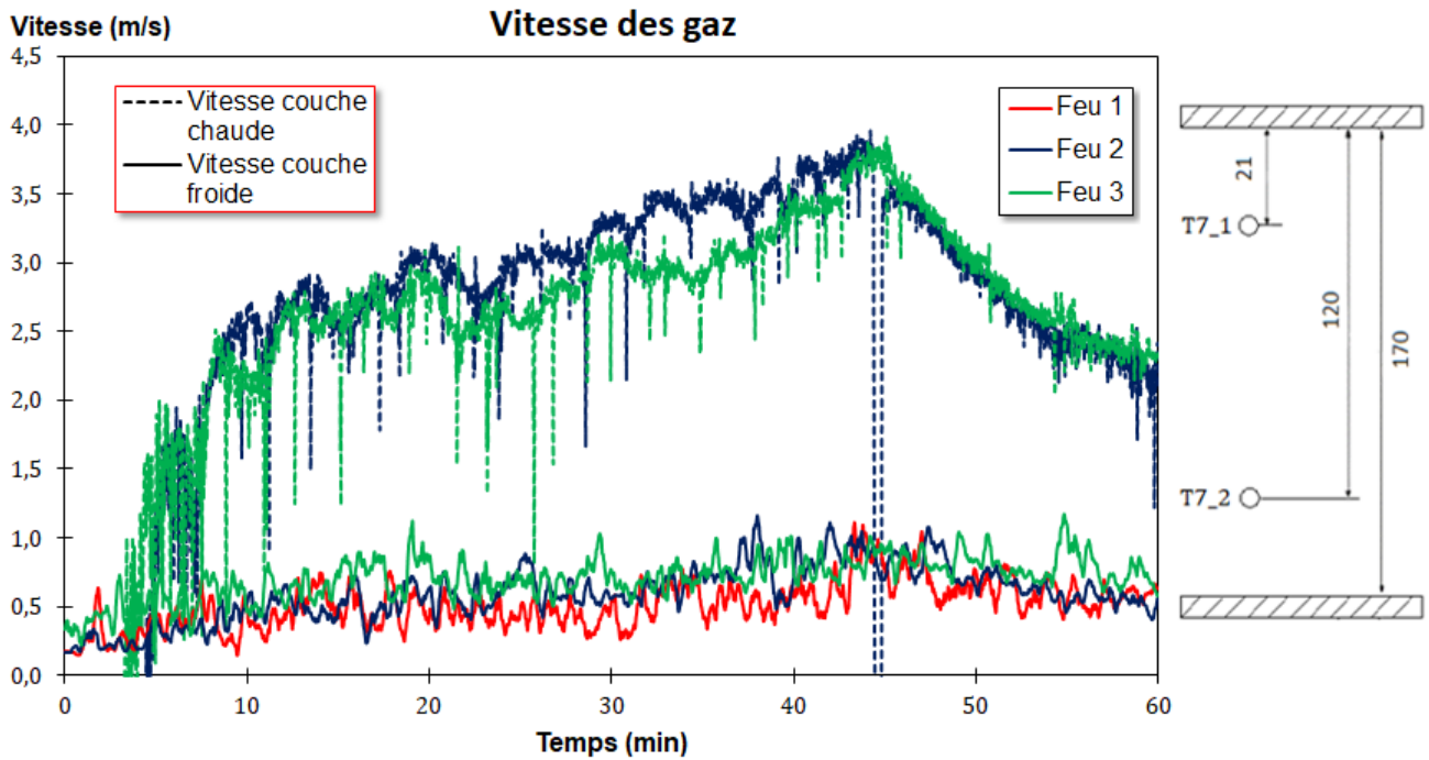
Figure F.2.12 – Mesures des vitesses effectuées sur l'arbre T7. La localisation verticale des sondes est indiquée en cm.
