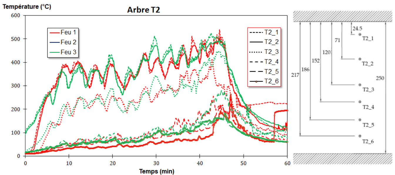
Figure F.2.2 – Mesures de température effectuées par les thermocouples de l'arbre T2. La localisation verticale des thermocouples est indiquée en cm.
