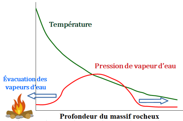
Figure 1.22 – Profil de la pression interstitielle sur les premiers centimètres de la roche exposée au feu.
