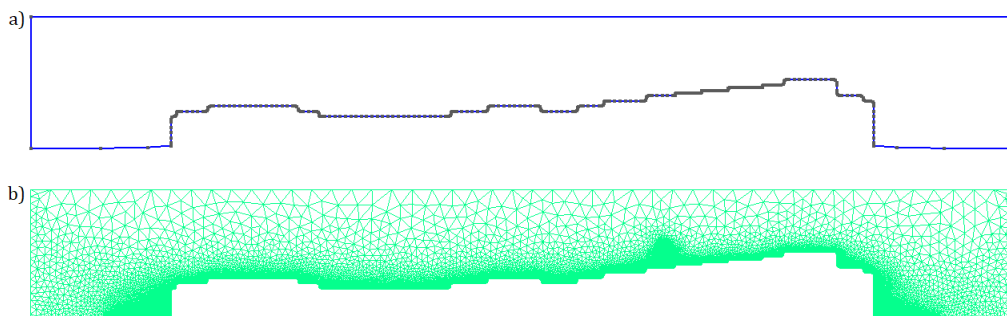
Figure 2.30 – a - Contour de la géométrie lissée utilisée par Cast3m lors de l'étude thermo-mécanique. b - Maillage réalisé grâce à GMSH.
