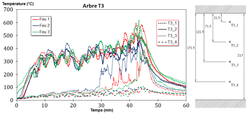
Figure F.2.3 – Mesures de température effectuées par les thermocouples de l’arbre T3. La localisation verticale des thermocouples est indiquée en cm.
