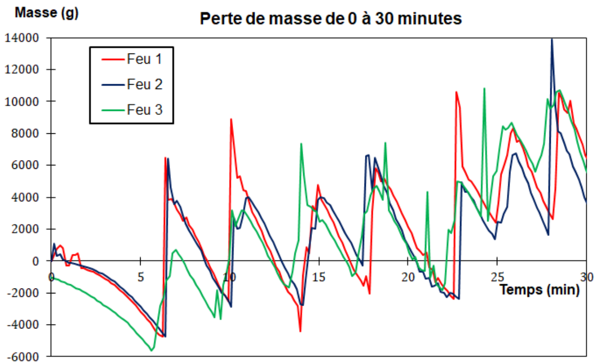
Figure F.2.13 – Perte de masse mesurée sur les 30 premières minutes des feux.
