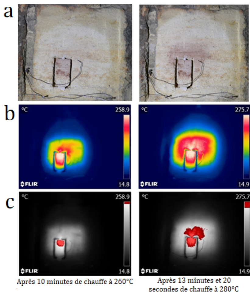
Figure 4.5 – a - Photographies dans le domaine visible (C. Ferrier). b - Photographies dans le domaine infrarouge (J.-C. Mindeguia). c - Champ de température montrant les surfaces dont la température excède 250^{\circ}\text{C} (en rouge).
