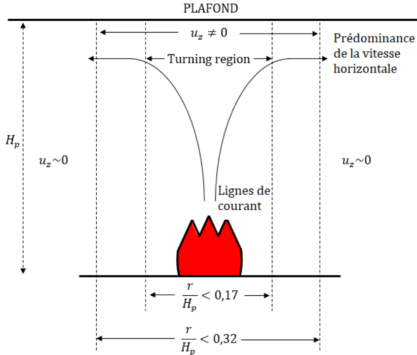
Figure 2.21 – Représentation schématique du passage du mouvement vertical au mouvement horizontal. L'hypothèse de vitesse exclusivement horizontale est seulement appliquée loin du feu.
