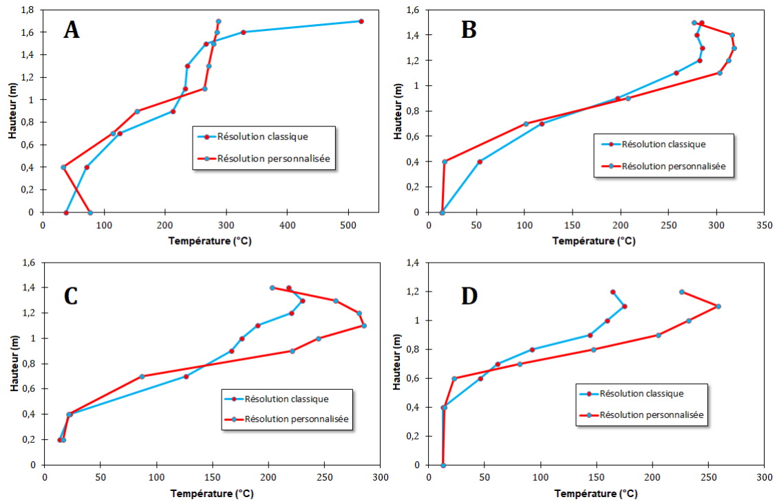
Figure 2.22 – Comparaison des profils de températures des arbres A, B, C et D entre une résolution classique sans l’hypothèse de vitesse exclusivement horizontale et une résolution personnalisée avec l’hypothèse.
