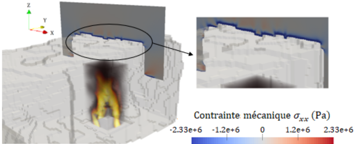
Figure 3.34 – Contrainte mécanique \sigma_{xx} 45 minutes après le début de la combustion. La simulation est effectuée par Cast3m dans le plan xOz (O étant le centre du foyer).
