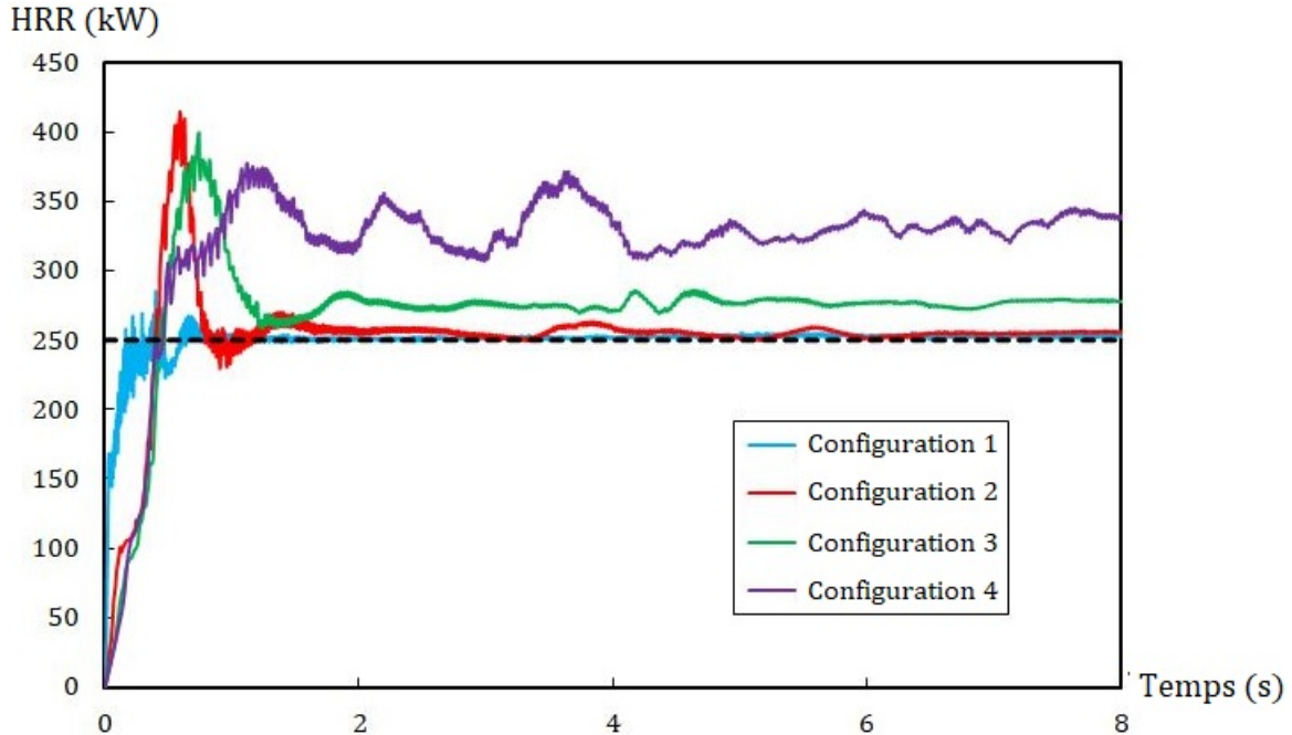
Figure 2.13 – Comparaison entre les HRR numériques pour chaque configuration [9]. La droite horizontale en pointillés noir correspond au HRR théorique.
