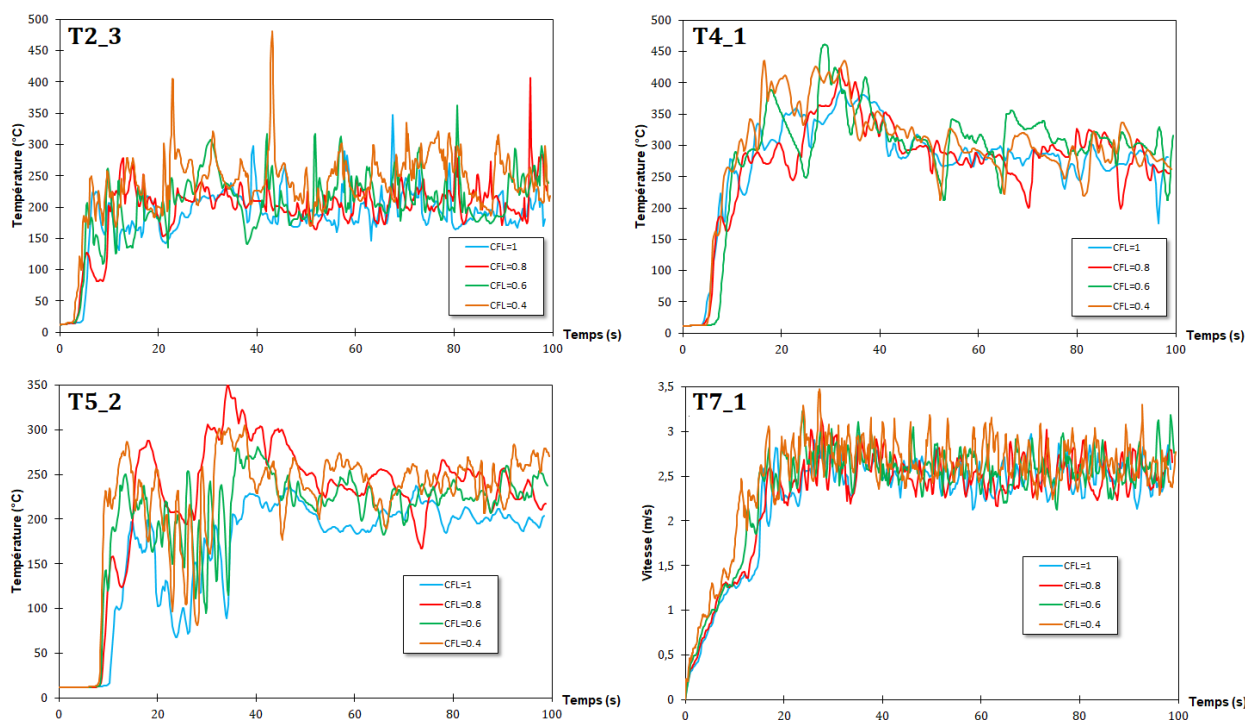
Figure 3.14 – Comparaison des champs de température aux points T2_3, T4_1 et T5_2 ainsi que de la vitesse en T7_1 pour 4 conditions CFL différentes (0,4, 0,6, 0,8 et 1).
