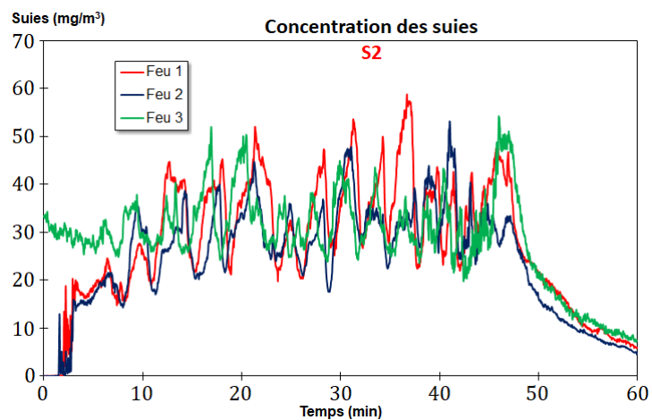
Figure F.2.11 – Mesures des concentrations en particules effectuées en S2.
