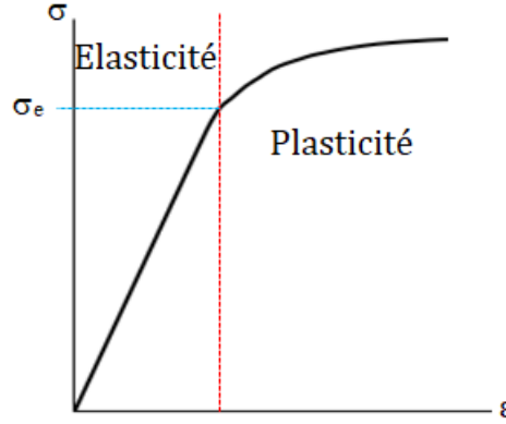
Figure 1.24 – Courbe de traction conventionnelle représentant la contrainte en fonction de la déformation. \sigma_e est la limite d'élasticité.
