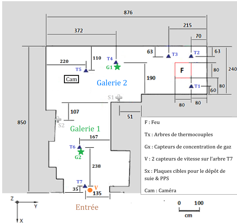
Figure 3.4 – Plan de la carrière indiquant l'emplacement du foyer, des arbres de thermocouples, des capteurs de concentration, des cibles pour les suies, des PPS, des capteurs de vitesse et de la caméra.
