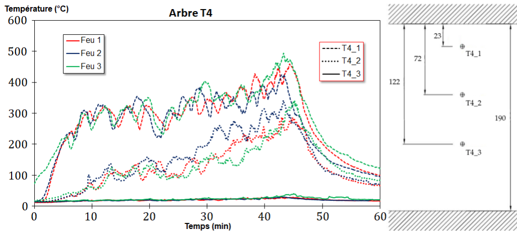
Figure F.2.4 – Mesures de température effectuées par les thermocouples de l’arbre T4. La localisation verticale des thermocouples est indiquée en cm.
