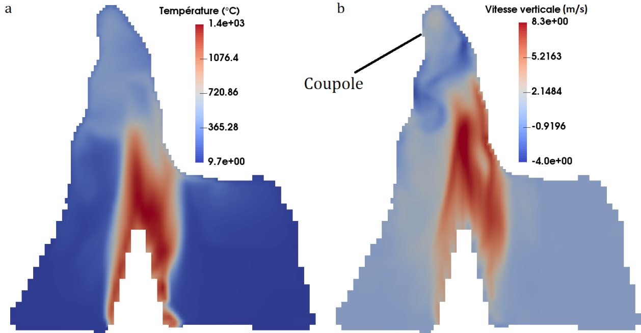
Figure 4.28 – Champs calculé sur une coupe orthogonale à l'axe de la galerie et passant par le centre du foyer 450 s après l'allumage d'un feu de 25 kg de bois. a - Champ de température. b - Champ de vitesse verticale.
