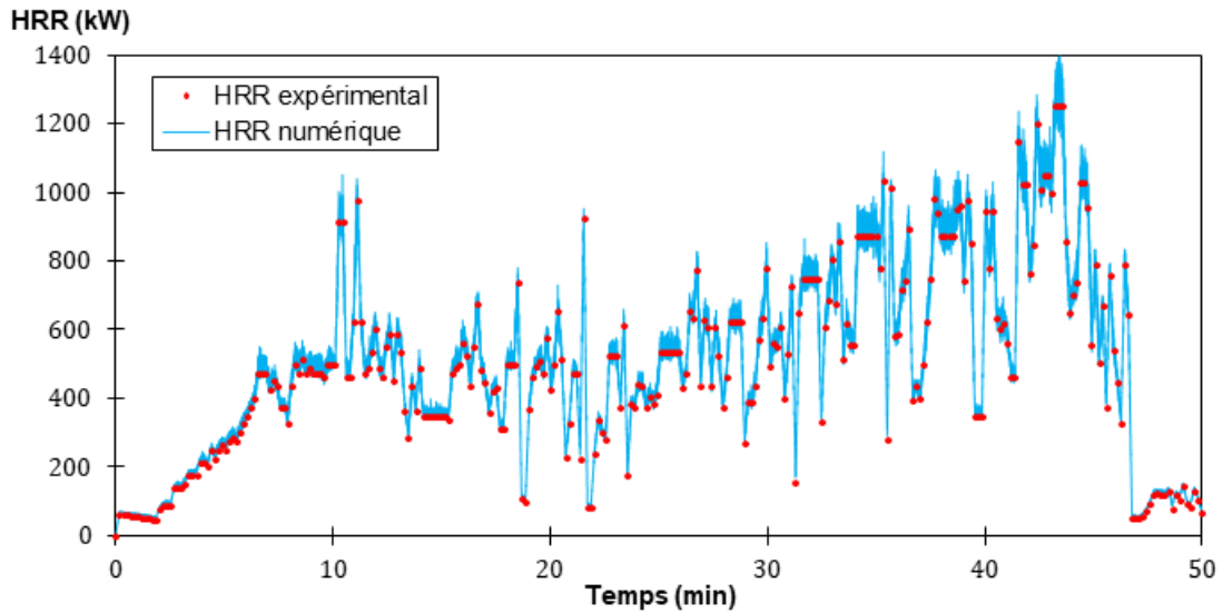
Figure 3.19 – Comparaison entre les HRR simulé et mesuré par la balance en supposant le pouvoir calorifique constant.
