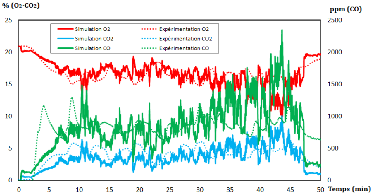
Figure 3.27 – Concentrations simulées et mesurées par les capteurs en C1.
