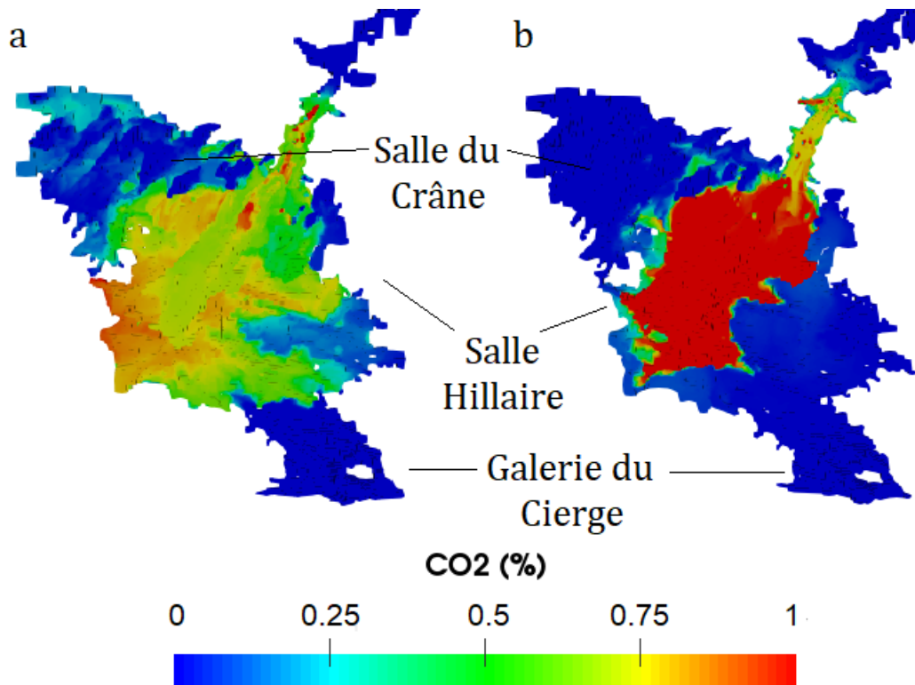
Figure 4.89 – Comparaison de la répartition du CO_2 au plafond de la Salle Hillaire. La géométrie est vue de dessus. a - Pour un foyer de 34 kg à l'emplacement du feu de la zone 2. b - Pour un foyer de 30 kg à l'emplacement du feu de la zone 5.
