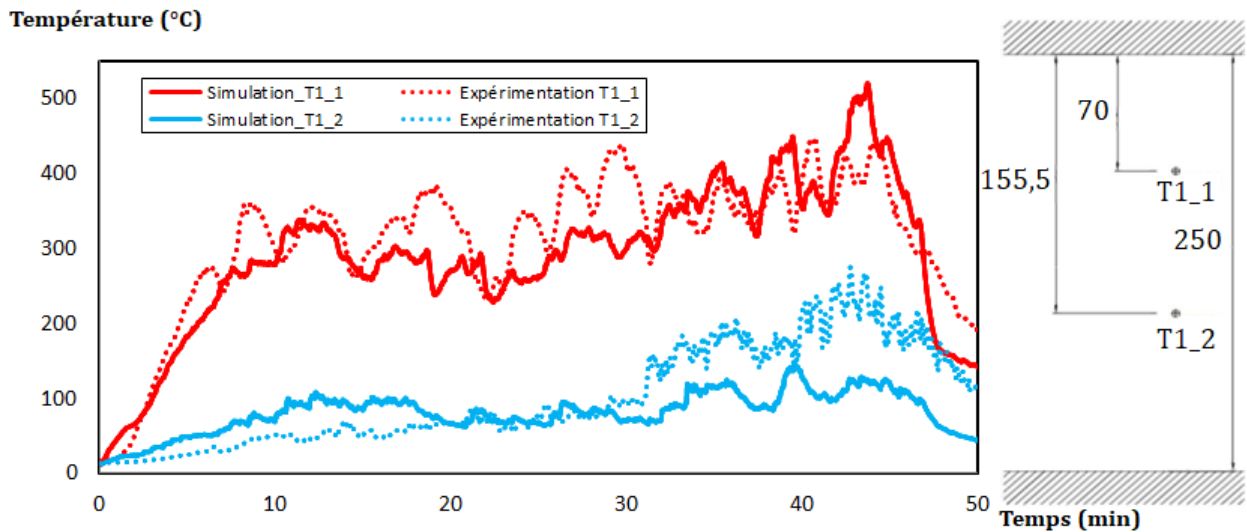
Figure 3.20 – Températures simulées et mesurées par les thermocouples de l'arbre T1. La localisation des thermocouples est indiquée à droite.
