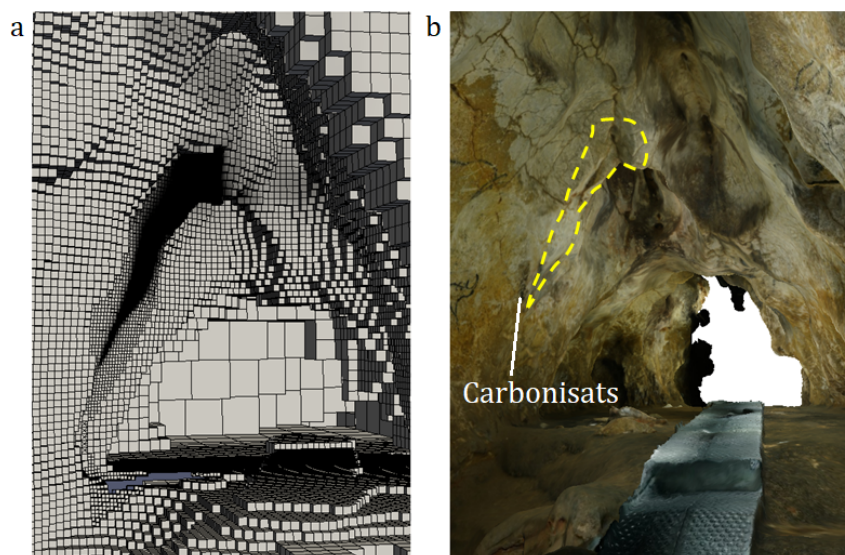
Figure 4.25 – a - Dépôt de suie simulé dans la géométrie numérique de la grotte Chauvet-Pont d’Arc pour un feu de 20 kg de bois dans la zone 1. b - Dépôt de suie numérique issu de la simulation (délimité en jaune) transposé dans la Galerie des Mégacéros (extrait de la photogrammétrique réalisée par T. Sagory / Équipe grotte Chauvet - MC).
