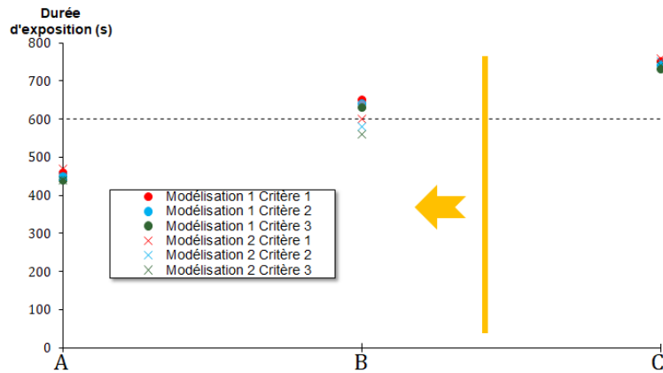
Figure 4.81 – Durée d'exposition de la surface altérée aux températures correspondant aux critères de couleur grise dans la zone 7 en fonction du protocole considéré. La ligne en pointillé correspond à la durée pour laquelle il y a reproduction des thermo-altérations observables in situ .
