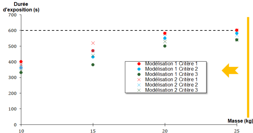
Figure 4.41 – Durée d'exposition de la surface altérée aux températures correspondant aux critères de couleur grise dans la zone 3 en fonction de la masse du foyer considéré. La ligne en pointillé correspond à la durée pour laquelle il y a reproduction des thermo-altérations observables in situ .
