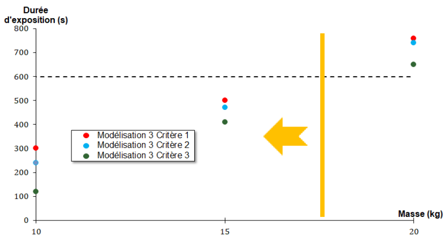
Figure 4.70 – Durée d'exposition de la surface altérée aux températures correspondant aux critères de couleur grise dans la zone 6 en fonction de la masse du foyer considéré. La ligne en pointillé correspond à la durée pour laquelle il y a reproduction des thermo-altérations observables in situ .
