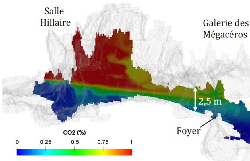
Figure 4.88 – Taux de CO_2 dans la Salle Hillaire à la fin de la combustion d’un foyer de 30 kg situé à l’emplacement du feu de la zone 5.
