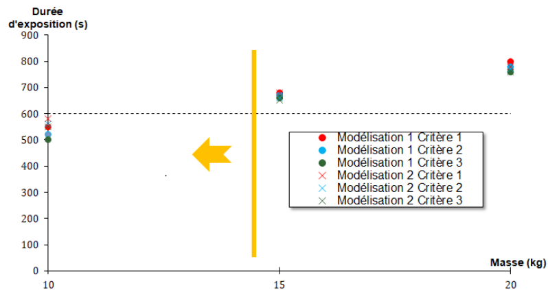
Figure 4.79 – Durée d'exposition de la surface altérée aux températures correspondant aux critères de couleur grise dans la zone 7 en fonction de la masse du foyer considéré. La ligne en pointillé correspond à la durée pour laquelle il y a reproduction des thermo-altérations observables in situ .
