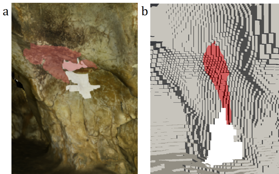
Figure 4.48 – a - Relevé des thermo-altérations de la zone 4 (F. Salmon). b - Changements de coloration simulés sur la paroi de la zone 4 pour un foyer de 10 kg de bois.
