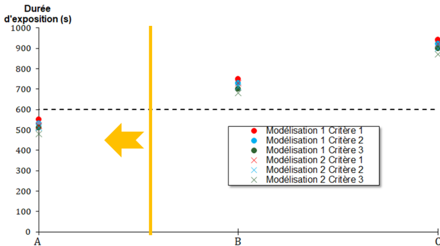
Figure 4.43 – Durée d'exposition de la surface altérée aux températures correspondant aux critères de couleur grise dans la zone 3 en fonction du protocole considéré. La ligne en pointillé correspond à la durée pour laquelle il y a reproduction des thermo-altérations observables in situ .
