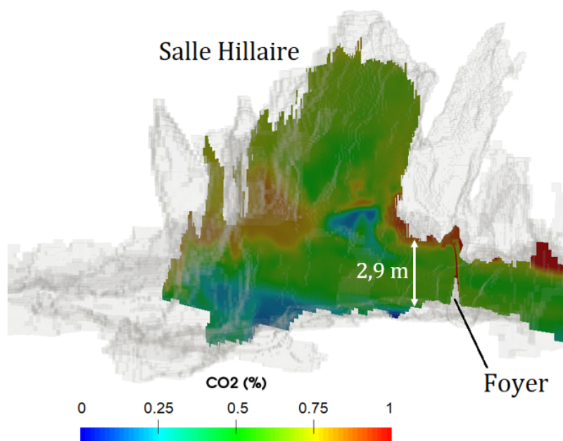
Figure 4.86 – Taux de CO_2 dans la Salle Hillaire à la fin de la combustion d'un foyer de 34 kg situé à l'emplacement du feu de la zone 2.
