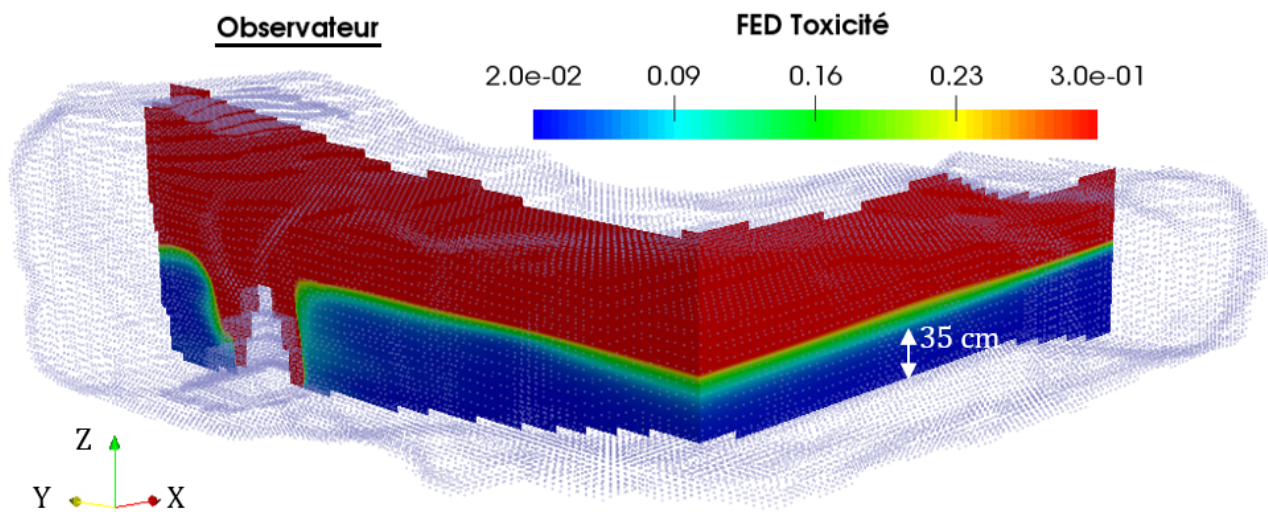
Figure 3.39 – FED relative à la toxicité pour un observateur séjournant dans la carrière pendant toute la combustion.
