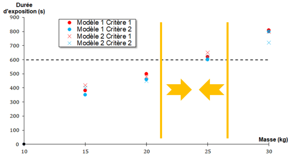
Figure 4.56 – Durée d'exposition de la surface altérée aux températures correspondant aux critères de rubéfaction dans la zone 5 en fonction de la masse du foyer considéré. La ligne en pointillé correspond à la durée pour laquelle il y a reproduction des thermo-altérations observables in situ .
