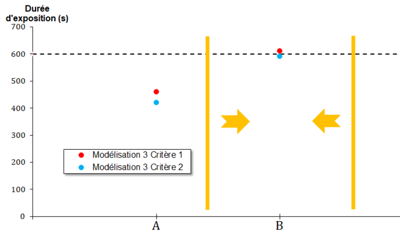
Figure 4.71 – Durée d'exposition de la surface altérée aux températures correspondant aux critères de rubéfaction dans la zone 6 en fonction du protocole considéré. La ligne en pointillé correspond à la durée pour laquelle il y a reproduction des thermo-altérations observables in situ .
