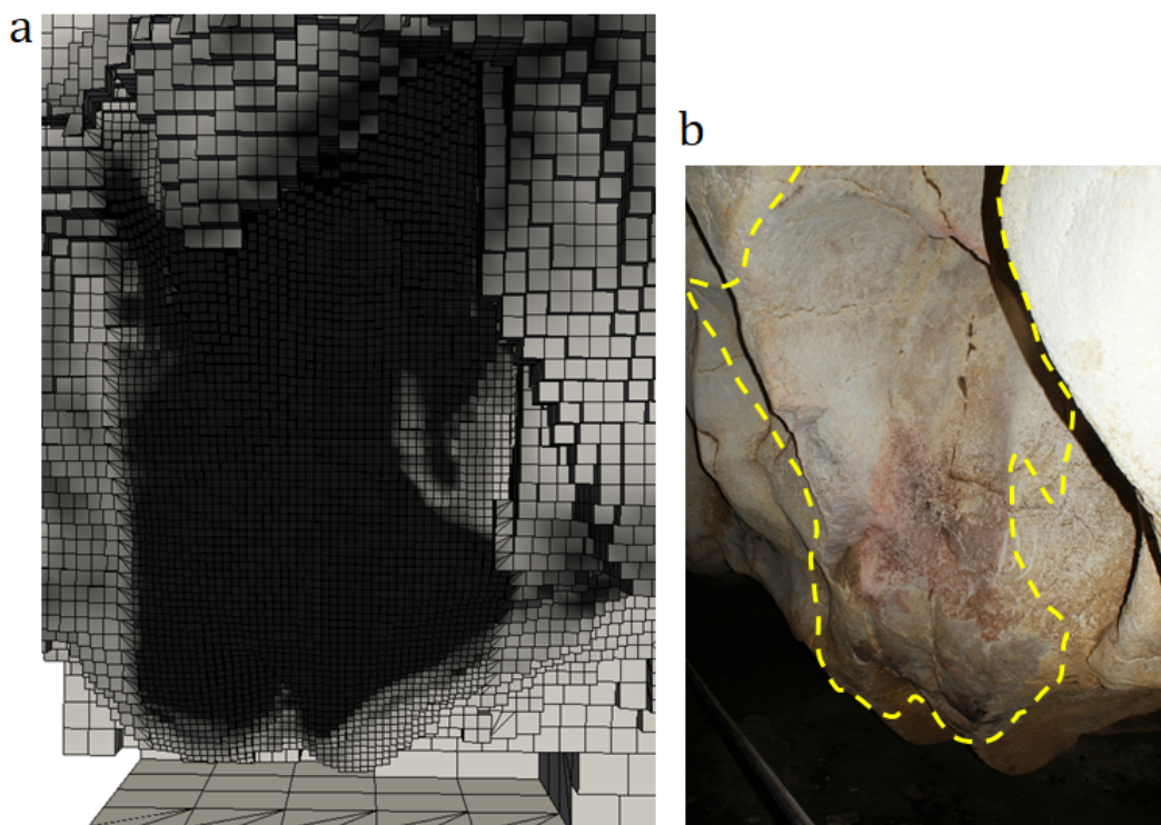
Figure 4.83 – a - Dépôt de suie simulé dans la géométrie numérique de la grotte Chauvet-Pont d'Arc pour un feu de 15 kg de bois dans la zone 7. b - Dépôt de suie numérique issu de la simulation (délimité en jaune) transposé dans la Galerie des Mégacéros (extrait de la photogrammétrie réalisée par T. Sagory / Équipe grotte Chauvet - MC).
