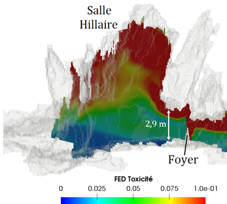
Figure 4.85 – FED relative à la toxicité pour un observateur ayant demeuré dans la Salle Hillaire pendant toute la combustion d'un foyer de 34 kg situé à l'emplacement du feu de la zone 2.
