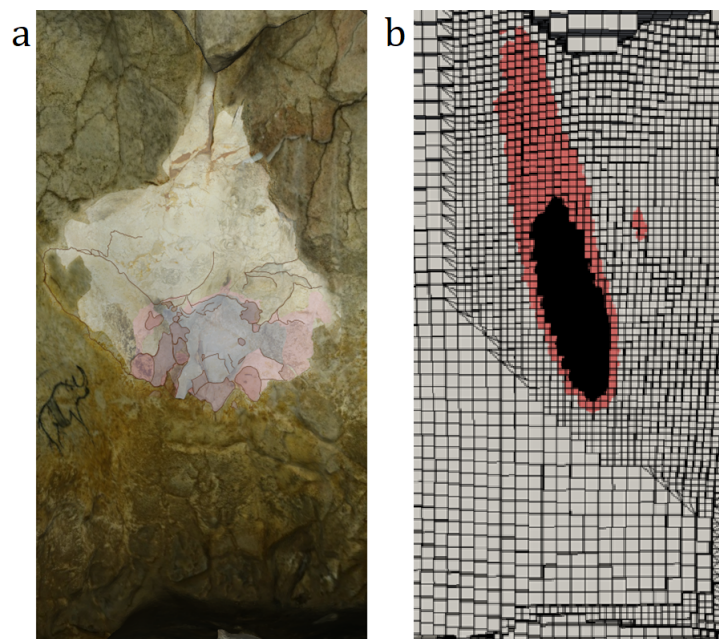
Figure 4.18 – a - Relevé des thermo-altérations (D. Lacanette et J.-C. Leblanc). b - Changements de coloration simulés sur la paroi de la zone 1 pour un foyer de 20 kg de bois.
