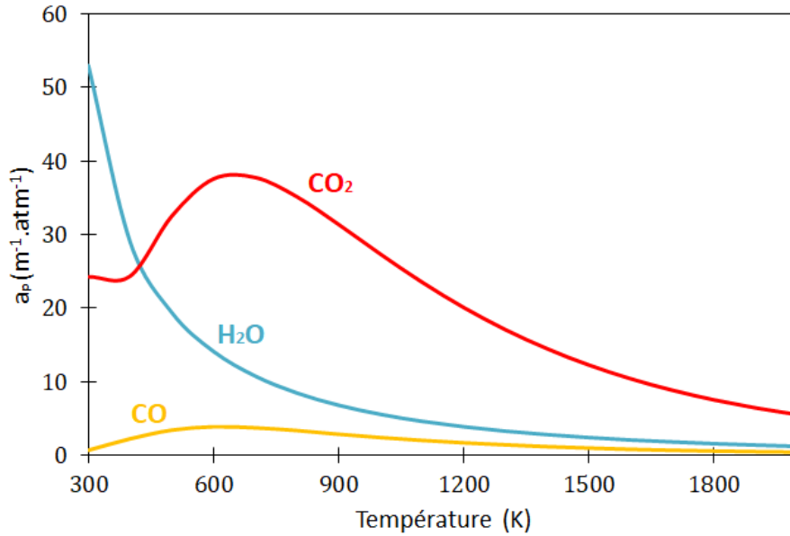
Figure B.1 – Coefficient d'absorption moyen de Planck du dioxyde de carbone, du monoxyde de carbone et de la vapeur d'eau.
