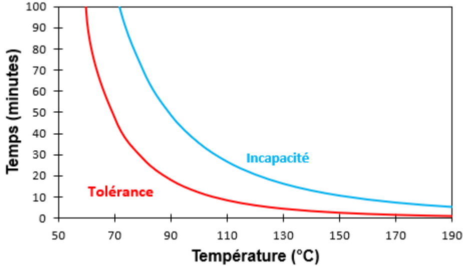
Figure 2.7 – Temps de tolérance (2.1.32) et d'incapacité (2.1.31) sous une température T .
