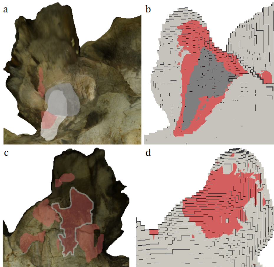
Figure 4.29 – a - Relevé des thermo-altérations de la paroi droite de la zone 2 (F. Salmon). b - Changements de coloration simulés sur la paroi droite de la zone 2 pour un foyer de 28 kg de bois. c - Relevé des thermo-altérations de la paroi gauche de la zone 2 (F. Salmon). d - Changements de coloration simulés sur la paroi gauche de la zone 2 pour un foyer de 28 kg de bois.
