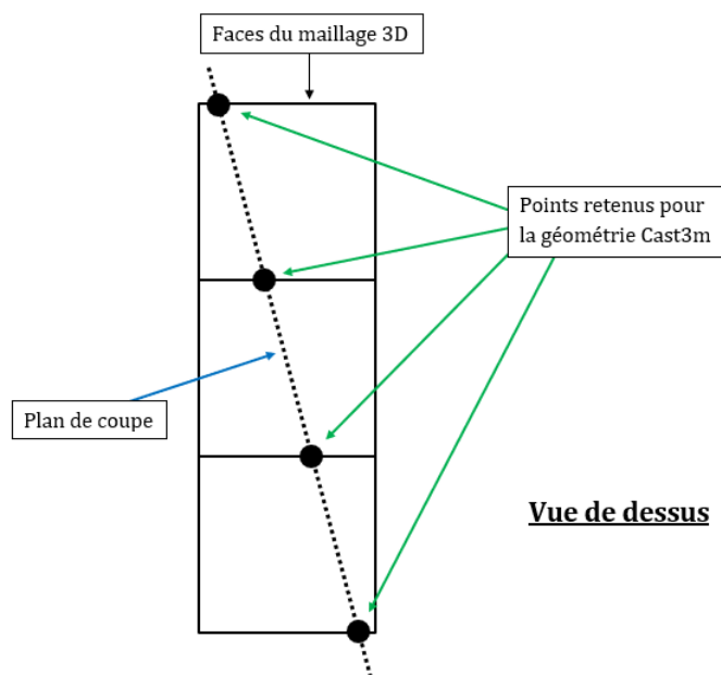
Figure E.1 – Construction des points qui formeront le contour de la géométrie 2D utilisée par Cast3m.
