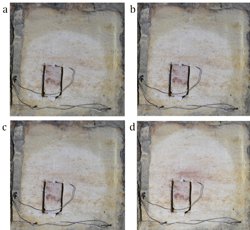
Figure 4.3 – État de la paroi et de l'échantillon ayant subi une chauffe à 260^{\circ}\text{C} (C. Ferrier). a - Après 5 minutes de chauffe. b - Après 10 minutes de chauffe. c - Après 20 minutes de chauffe. d - Après 50 minutes de chauffe.
