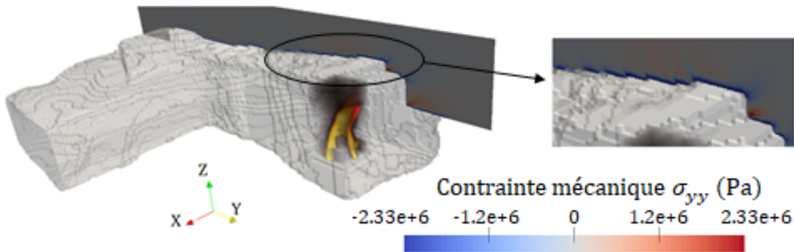
Figure 3.35 – Contrainte mécanique \sigma_{yy} 45 minutes après le début de la combustion. La simulation est effectuée par Cast3m dans le plan yOz (O étant le centre du foyer).
