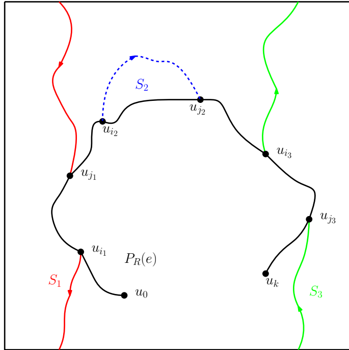
Figure .24 – Situation of Lemma 1.10.
