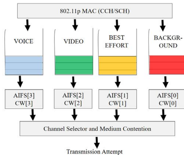
FIGURE 3.2 – Quatre catégories d'accès dans le standard IEEE 802.11p.
