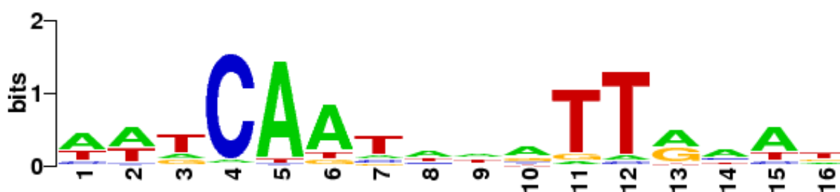
Figure 37: Séquence consensus du site de fixation à la protéine IHF, régulateur global.
