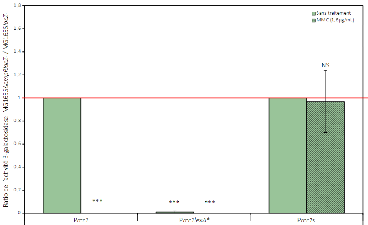
Figure 43: Influence de la protéine OmpR sur l'activité du Pcr1
