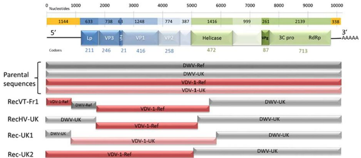
Figure 26 : Schémas des recombinaisons détectées entre des virus DWV et VdV-1 chez 4 souches recombinantes (Dalmon et al., 2017)
