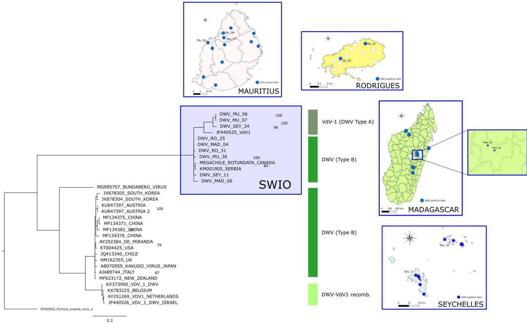
Figure 47 : Arbre bayésien de diversité des séquences de DWV obtenues dans le SOOI. L'arbre est construit avec 9 séquences (2 de Madagascar, 3 de Maurice, 2 de Rodrigues et 2 des Seychelles). Les nombres placés sur les nœuds indiquent la probabilité a posteriori d'appartenir à tel nœud. Le modèle choisi pour construire l'arbre est le modèle suivant : GTR+I+G.
