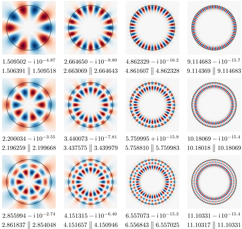
FIGURE 5.1 – Représentations graphiques des parties réelles de u(r, \theta) = w_m(r)e^{im\theta} , avec p = +1 , dans un disque de rayon R = 1 et d'indice optique n_0 = 5 . De gauche à droite les valeurs de m sont 5, 10, 20 et 40. De haut en bas les valeurs de j sont 0, 1 et 2. Sous chaque figure, on donne la résonance complexe calculée en résolvant l'équation modale (5.3). Sur la deuxième ligne, on donne la valeur réelle de l'asymptotique à cinq termes (5.4) et, séparé par ||, notre asymptotique à douze termes de la section 6.6.1.2 page 167.
