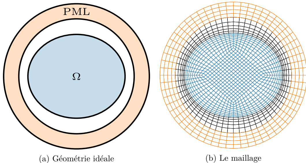
FIGURE 9.1 – À gauche : représentation de la géométrie idéale du domaine de calcul. À droite : représentation du maillage.
