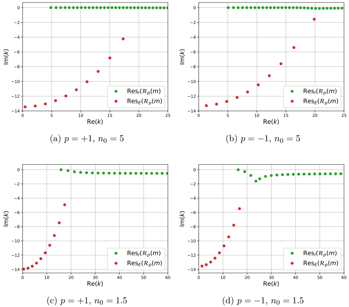
FIGURE 3.2 – Représentation graphique des zéros de la fonction modale \mathcal{D}_{p;m} défini en (3.5) pour m = 20 . La colonne de gauche représente p = +1 et celle de droite représente p = -1 . La ligne du haut représente n_0 = 5 et celle du bas représente n_0 = 1.5 .
