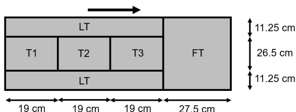
FIGURE 2.7 – Schéma des trappes situées à l'aval du canal d'expérience. La flèche indique le sens de l'écoulement.
