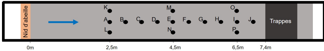
FIGURE 2.9 – Schéma du canal en vue de dessus montrant la position des profils de vitesses indexés de A à P.
