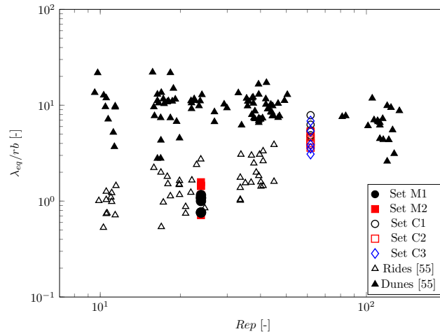
FIGURE 3.8 – Longueur d’onde à l’équilibre divisée par le rayon hydraulique en fonction du nombre de Reynolds particulaire. Représentation originale de Colombini et Stocchino 2011 [33].
