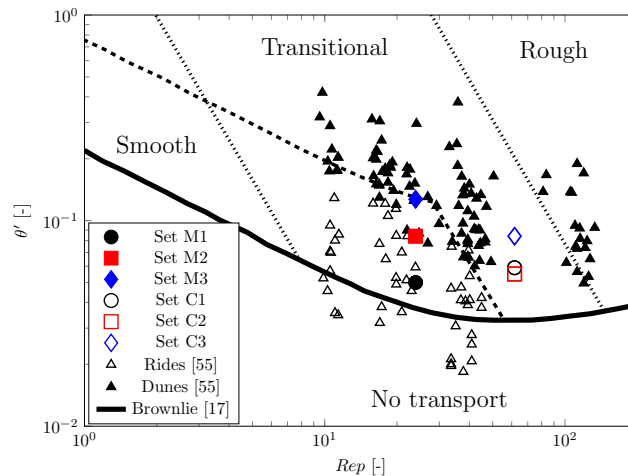
FIGURE 3.9 – Nombre de Shields effectif en fonction du nombre de Reynolds particulaire. Lignes issues de Brownlie 1981 [17]. Représentation originale de Colombini et Stocchino 2011 [33].
