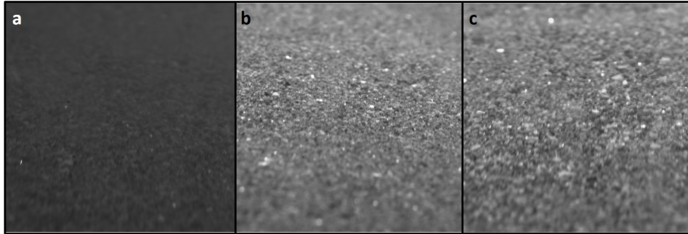
FIGURE 5.12 – Images prises lors des tests réalisés avec le sable S_{353/0,39} pour une épaisseur de \delta = 10mm avec les rugosités suivantes au fond : a) dépoli ; b) granité 4mm ; c) imprimé 77.
