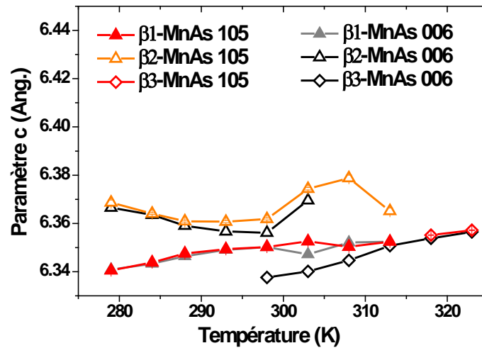
FIGURE 5.28 – Paramètres de maille c en fonction de la température mesuré à partir des positions des pics 105 et 006.
