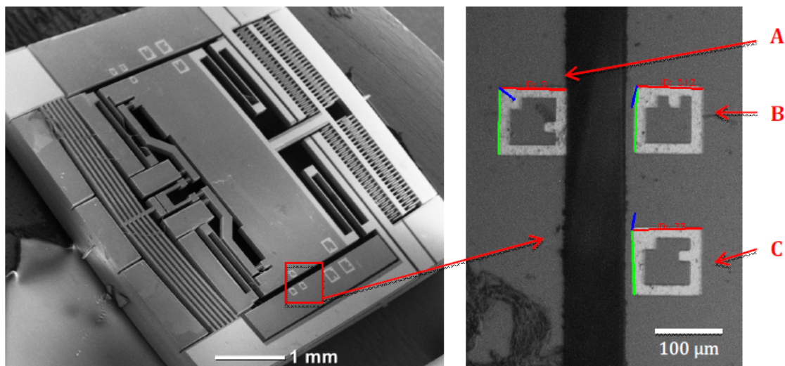
FIGURE 1.6 – Système micro-mécatronique présentant des mire utilisées comme marqueurs [24].
