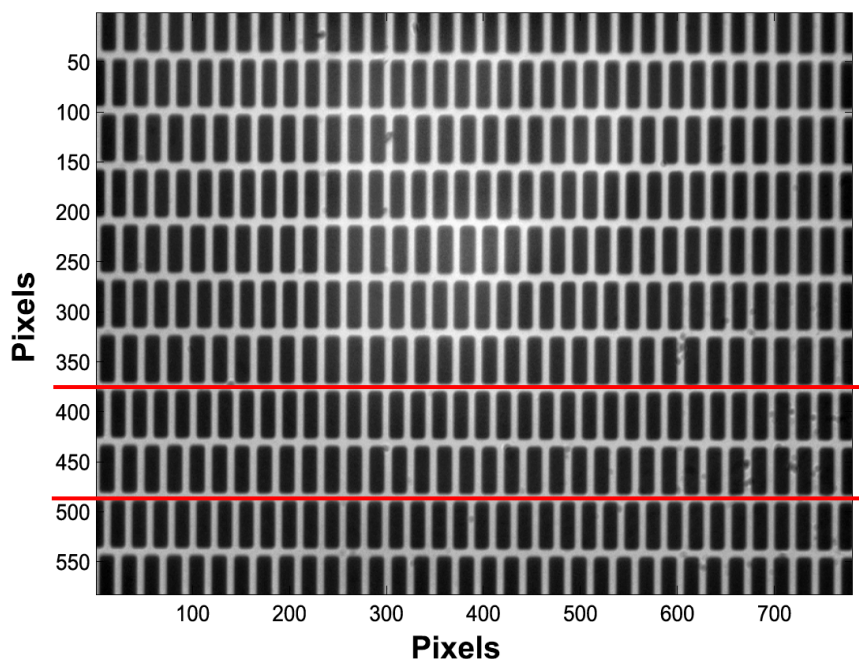
FIGURE 3.8 – Mire de Vernier 1D fabriquée en salle blanche par photolithographie d'aluminium sur du verre, telle qu'observée sur le dispositif expérimental. \lambda_1 = 8 \mu\text{m} , \lambda_2 = 8.4 \mu\text{m} , \Lambda = 168 \mu\text{m} .
