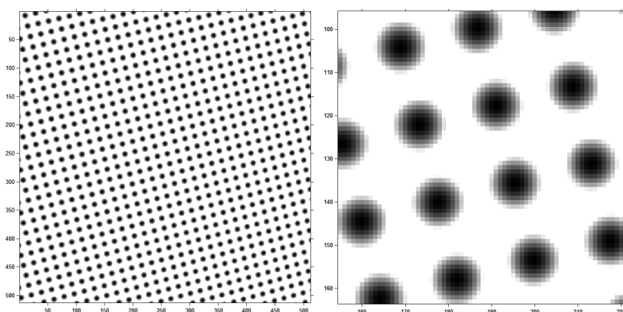
FIGURE 6.6 – Mire périodique 2D ( \lambda = 1 mm) simulée pour un modèle sténopé ( \bar{f} = 20 mm; \bar{n}_0 = \bar{m}_0 = 3.2 mm; \bar{k}_n = \bar{k}_m = 100 mm -1 ; dimension 640 × 640 pixels).
