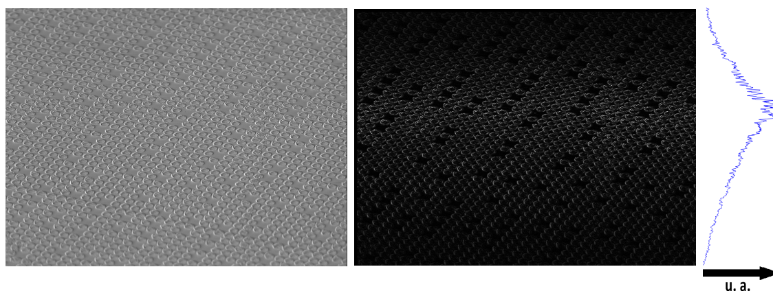
FIGURE 6.1 – Illustration du flou présent sur une image de mire pseudo-périodique réalisée par un MEB (donc ici en projection parallèle). A gauche, l'image d'origine ; au centre, une cartographie du flou (en clair les pixels nets, en foncé les pixels flous) basée sur l'écart d'intensité entre un pixel et ses voisins ; à gauche, représentation graphique du flou vertical (moyenne horizontale des intensités), avec une échelle arbitraire.
