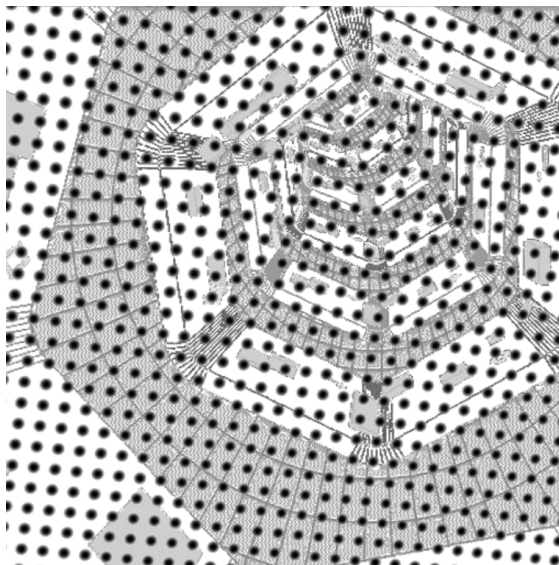
FIGURE E.2 – Mire périodique 2D ( \lambda = 1 mm) simulée pour un modèle sténopé ( f = 20 mm ; n_0 = m_0 = 3.2 mm ; k_n = k_m = 100 mm -1 ; dimension 640 × 640 pixels) soumis à un bruit variable.
