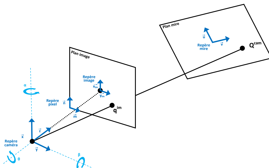
FIGURE 6.4 – Repères utilisés pour la mesure 6 DDL. Les paramètres extrinsèques à évaluer sont définis dans le repère caméra.
