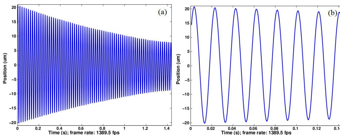
FIGURE 3.11 – Déplacement de la navette du dispositif compliant après impulsion, tel que mesuré par vision avec une vitesse d'acquisition de 1389.5 fps. (a) vue large ; (b) zoom.
