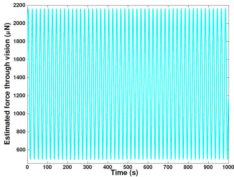
FIGURE D.2 – Résultat expérimental : mesure de force par vision suivant le temps, pour un déplacement sinusoïdal de l'actionneur.
