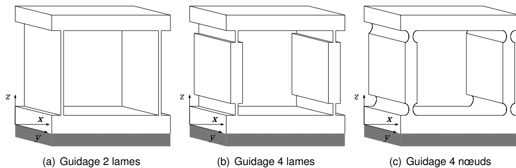
FIGURE D.8 – Les trois types de guidage flexibles considérés. On retiendra la liaison par 4 lames, fournissant un bon compromis face aux instabilités et aux contraintes mécaniques.
