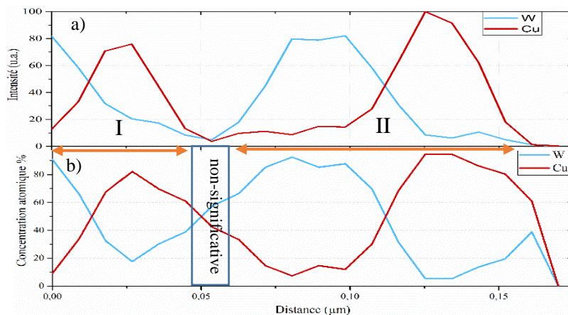
Figure 4.18. a) Profils montrant la variation de l'intensité et b) de la concentration atomique du W et du Cu mesurés le long de la zone définie par la ligne orange présentée sur la figure 4.17.
