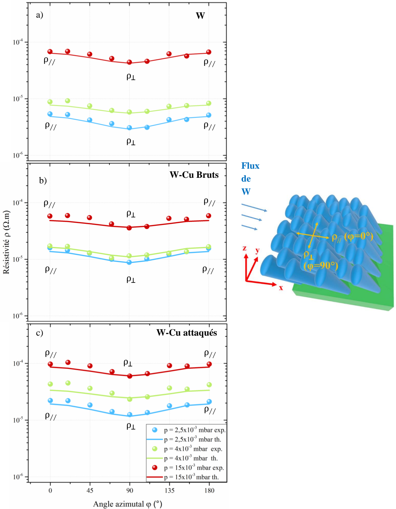
Figure 5.13. Variation de la résistivité électrique en fonction de l'angle azimutal \varphi pour a) les films de W, b) les films de W-Cu bruts et c) les films de W-Cu gravés. d) Représentation schématique indiquant les directions des résistivités électriques.
