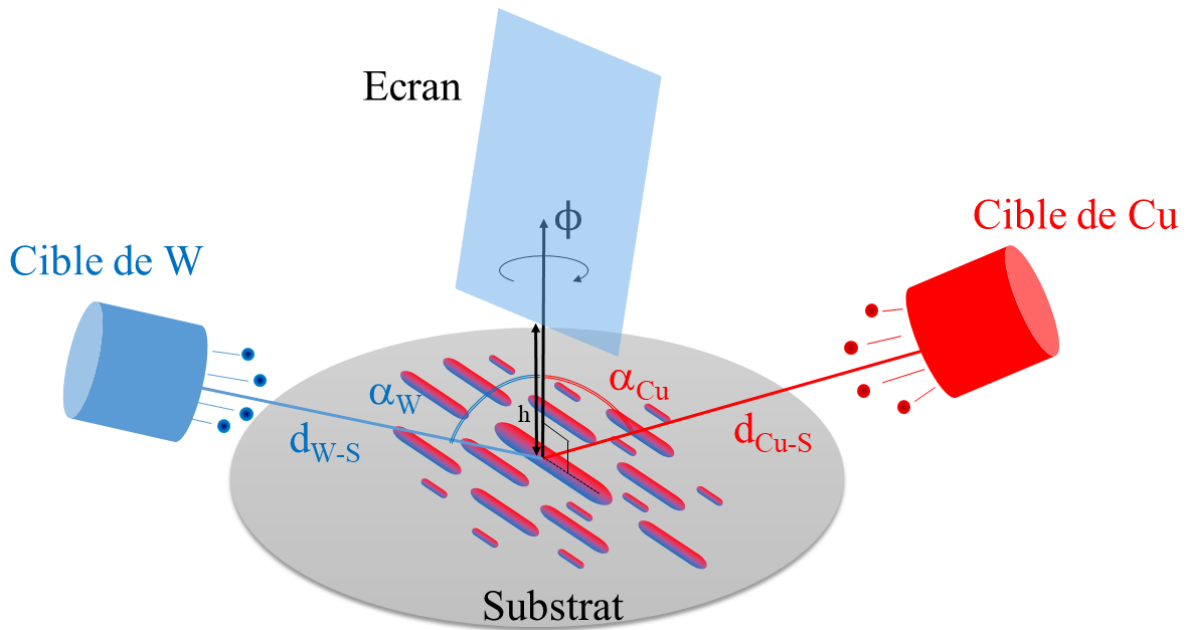
Figure 2.3. Schéma de principe de co-pulvérisation cathodique en ajoutant un écran.
