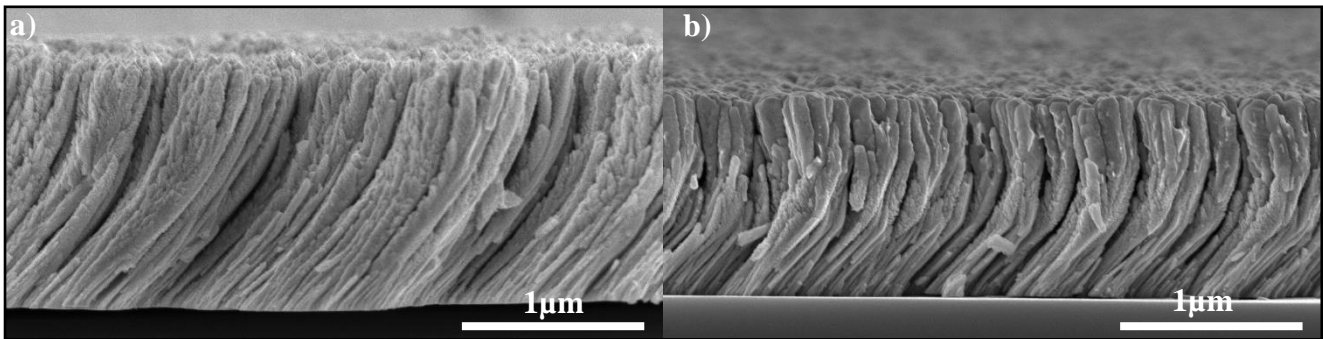
Figure 1 Films minces de W-Cu architecturés a) déposé à pression croissante et b) déposé à différentes pressions et différentes intensités du courant pour les deux cibles.
