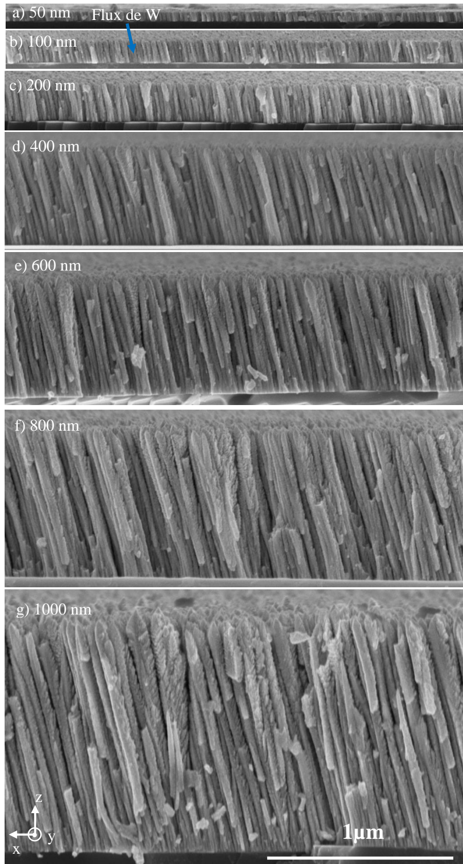
Figure 3.6. Observations MEB en électrons secondaires de la tranche des films de W déposés à p = 15 \times 10^{-3} mbar avec I_w = 140 mA. Ces films ont différentes épaisseurs : a) 50 nm, b) 100 nm, c) 200 nm, d) 400 nm, e) 600 nm, f) 800 nm et g) 1000 nm.
