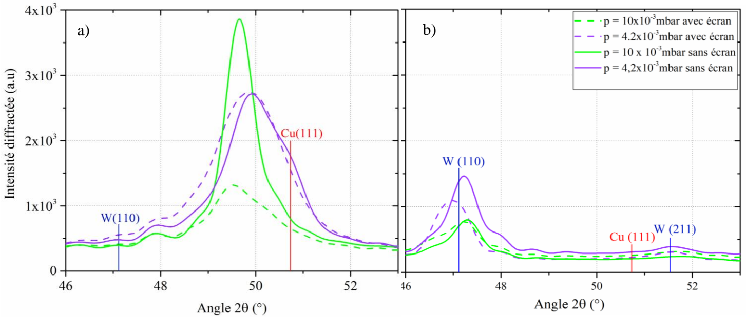
Figure 4.28. Diffractogrammes de rayons X de films W-Cu pour deux différentes pressions de pulvérisation, avec et sans écran. a) I_W = 50 \text{ mA} et I_{Cu} = 140 \text{ mA} . b) I_W = 140 \text{ mA} et I_{Cu} = 50 \text{ mA} .
