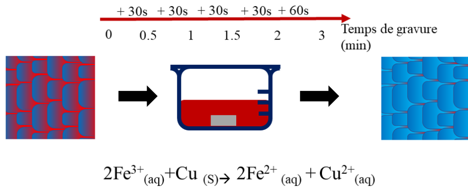
Figure 2.12. Représentation schématique de l'étude du temps de gravure chimique humide.
