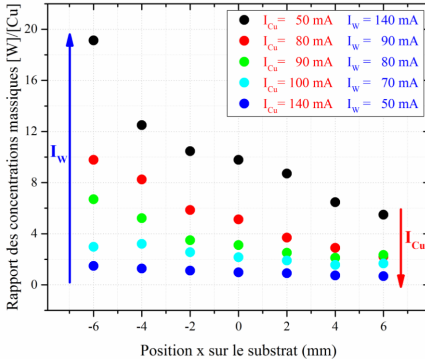
Figure 4.4. Rapport des concentrations massiques de W et de Cu [W]/[Cu] en fonction de la position x sur le substrat et pour différentes intensités de courant des cibles de W et Cu. Les mesures de concentrations massiques sont effectuées à sept endroits différents. Le centre du substrat correspond à x = 0 mm ; x = -6 mm est le côté gauche (proche de la cible en W) et x = +6 mm est le côté droit (proche de la cible en Cu).
