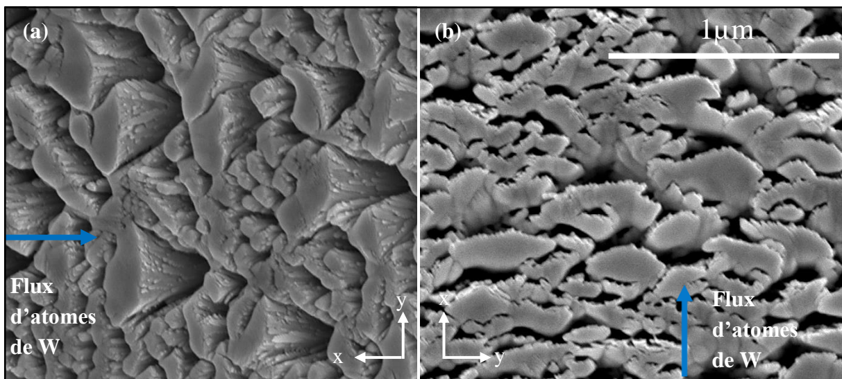
Figure 3.1. Images MEB en électrons secondaires (a) de la surface d'un film de W, (b) de la surface du même échantillon mais après une rotation de -90^\circ et une inclinaison de 35^\circ .
