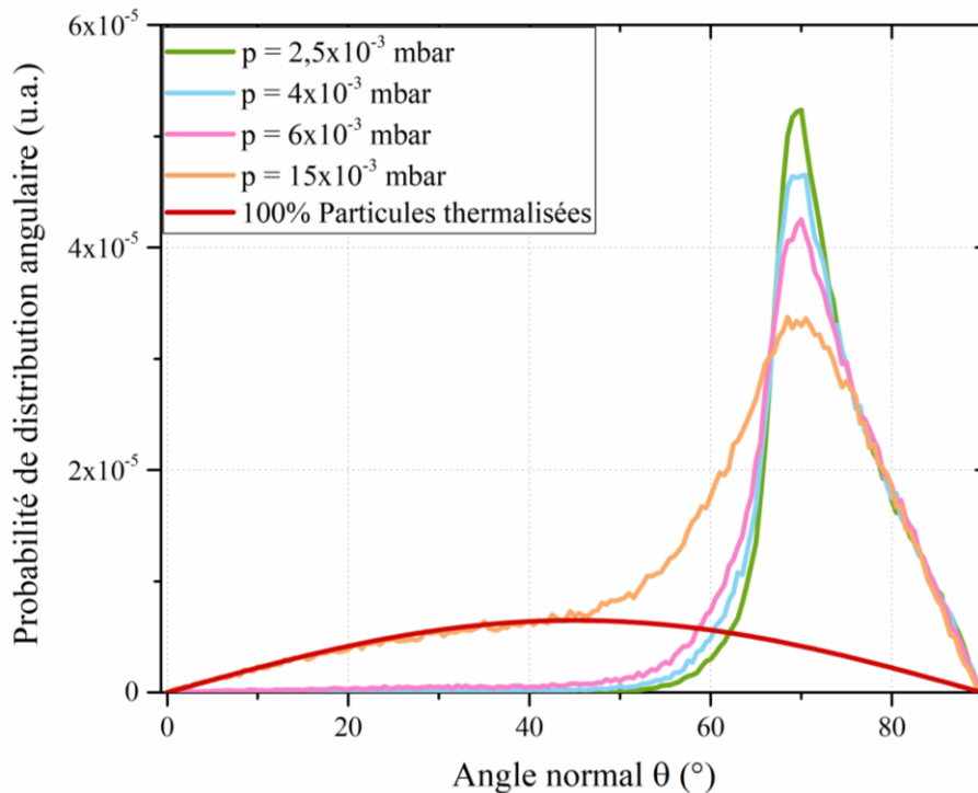
Figure 3.17. Variation de la probabilité de distribution angulaire des particules pulvérisées en fonction de la pression de travail.
