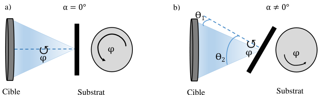
Figure 2.4. Variation de la distribution angulaire des particules pulvérisées en fonction de l'angle azimutal \varphi du substrat, a) pour \alpha = 0^\circ et b) pour \alpha \neq 0^\circ .
