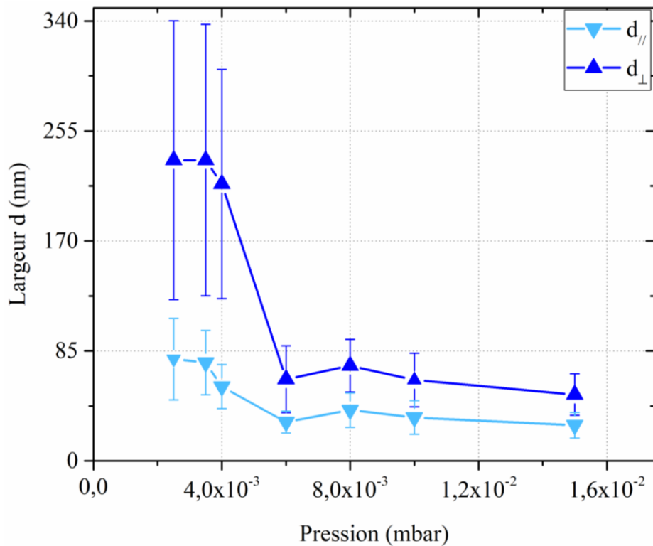
Figure 3.13. Variation des largeurs perpendiculaires d_{\perp} et parallèles d_{\parallel} au flux de W pour la série de films minces déposés pour différentes pressions de travail.
