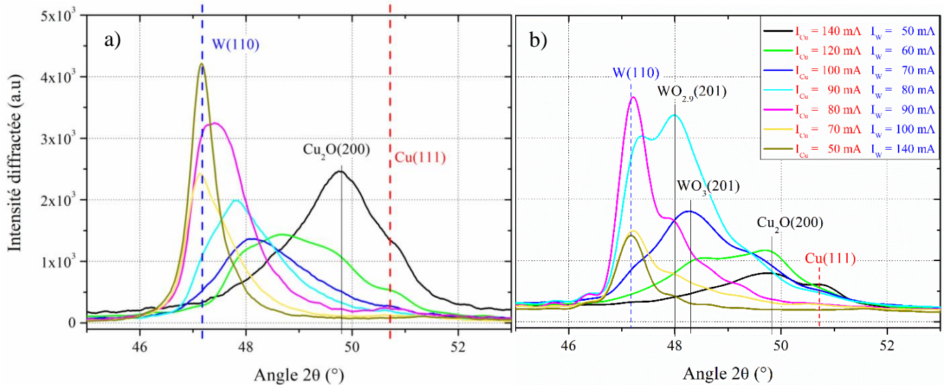
Figure 4.5. Diffractogrammes des rayons X des dépôts de W-Cu préparés en variant les intensités de courant des deux cibles : a) mesures prises avant recuit ; b) mesures prises après recuit à T = 473 K pendant 5 heures à l'air.
