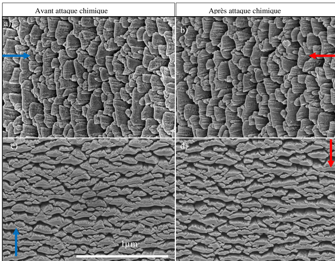
Figure 5.5. Images MEB en électrons secondaires de la surface d'un film de W-Cu a) avant et b) après gravure du Cu, sans rotation et sans inclinaison, c) avant d) après gravure du Cu avec rotation de -90° et inclinaison de 35°.
