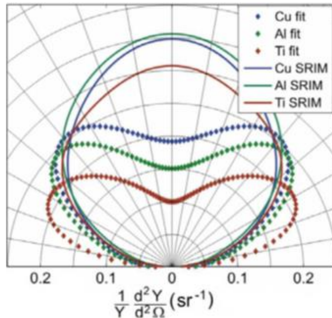
Figure 1.3. Lois de répartition angulaire des atomes arrivant sur le substrat pour le cuivre, l'aluminium et le titane [21, 22].
