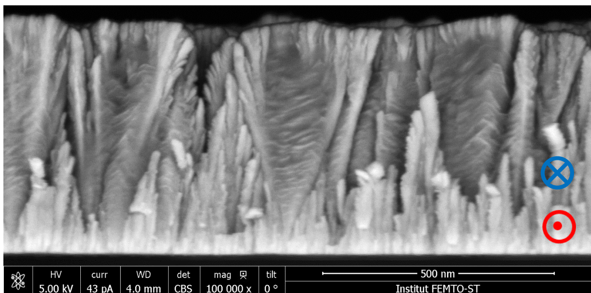
Figure 4.21. Observation MEB avec des électrons rétrodiffusés de la vue du côté de la cible de Cu du film de W-Cu déposé à 3,5 \times 10^{-3} mbar.
