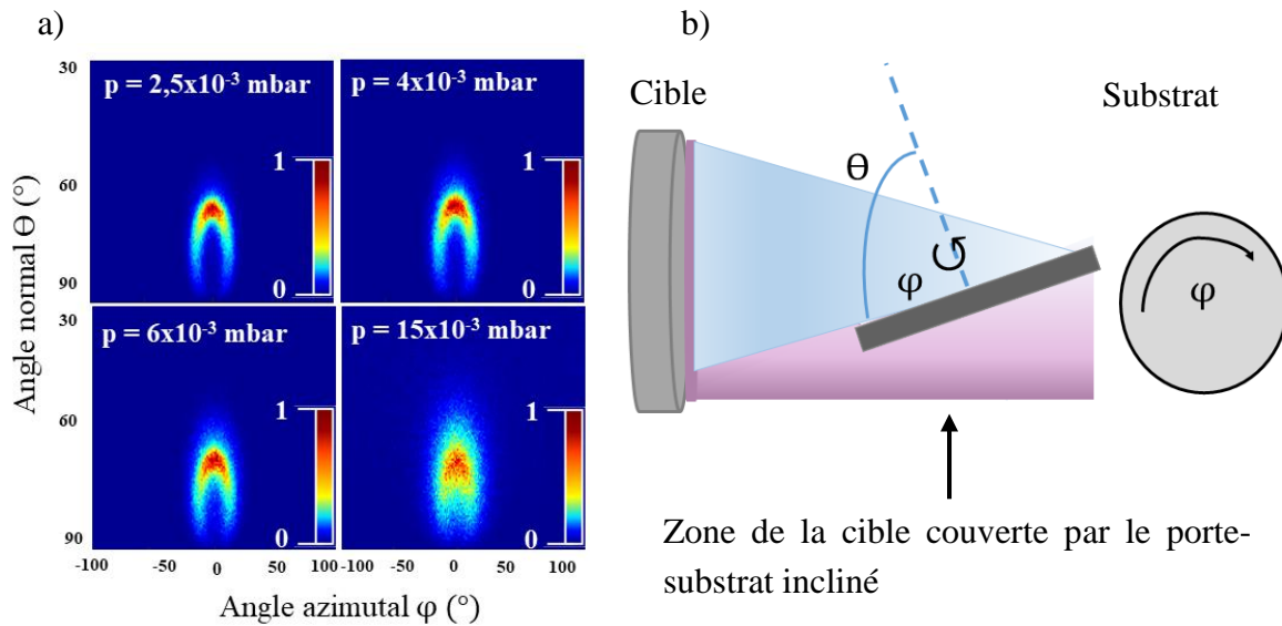
Figure 3.16. a) Angle normal \Theta des particules de W arrivant sur le substrat en fonction de l'angle azimutal \varphi calculé avec le logiciel SIMTRA [16] pour les films de W déposés à des pressions de 2,5 - 4 - 6 et 15 \times 10^{-3} mbar. b) Représentation schématique de la projection de la distribution des particules sortant de la cible pour arriver au substrat.
