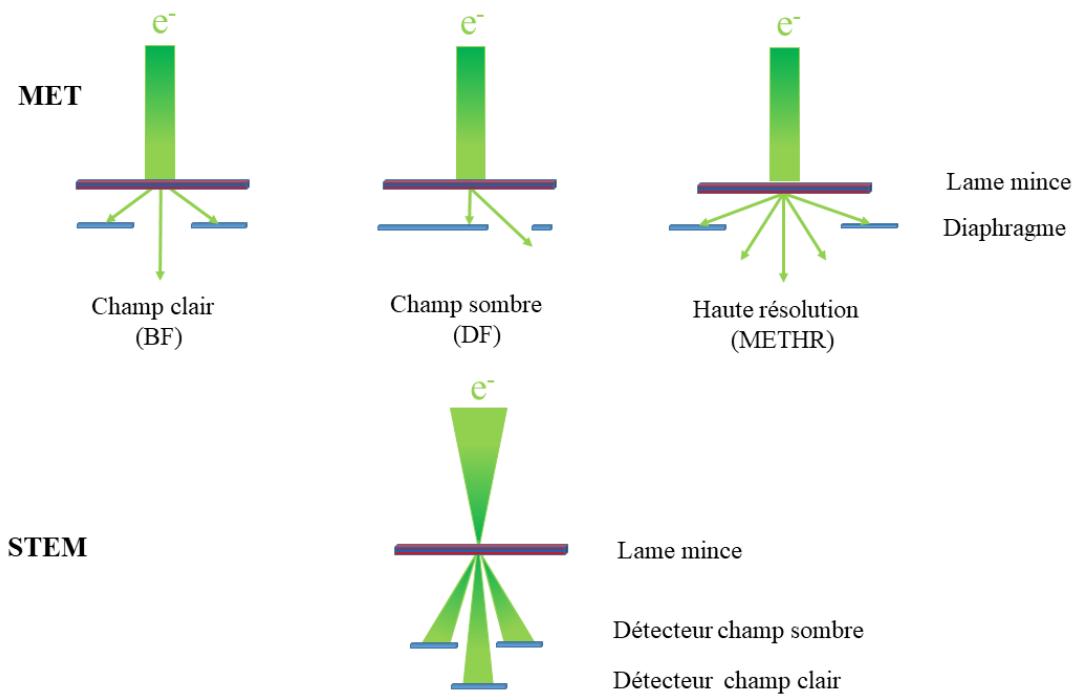
Figure 2.8. Représentation schématique du contraste en imagerie MET et STEM.
