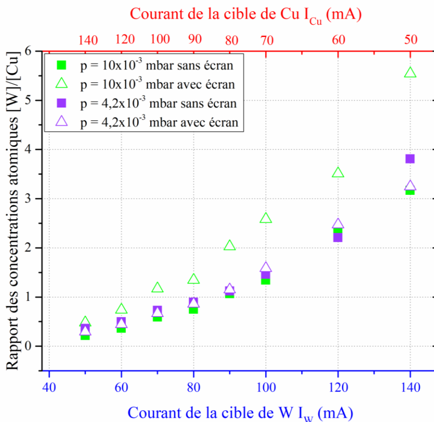
Figure 4.27. Variation des rapports des concentrations atomiques [W]/[Cu] en fonction des intensités de courant des cibles W et Cu. Ces rapports sont mesurés pour les deux séries déposées à basse pression avec et sans écran ainsi que pour les deux séries déposées à pression élevée avec et sans écran.
