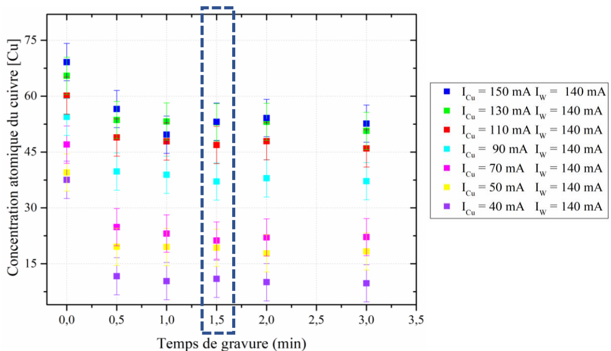
Figure 2.13. Variation de la concentration atomique du Cu en fonction du temps d'attaque chimique.
