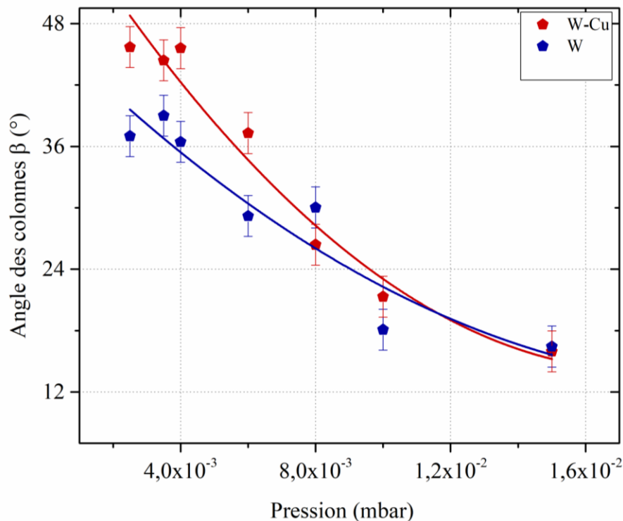
Figure 4.23. Angle des colonnes en fonction de la pression de travail utilisée pour préparer des films de W et de W-Cu. Les films de W-Cu sont déposés à I_W = 140 mA et à I_{Cu} = 40 mA. Les films de W sont déposés à I_W de 140 mA.
