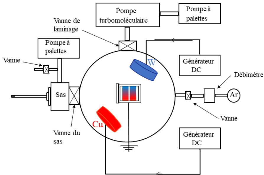
Figure 2.2. Schéma de l'enceinte de pulvérisation cathodique.
