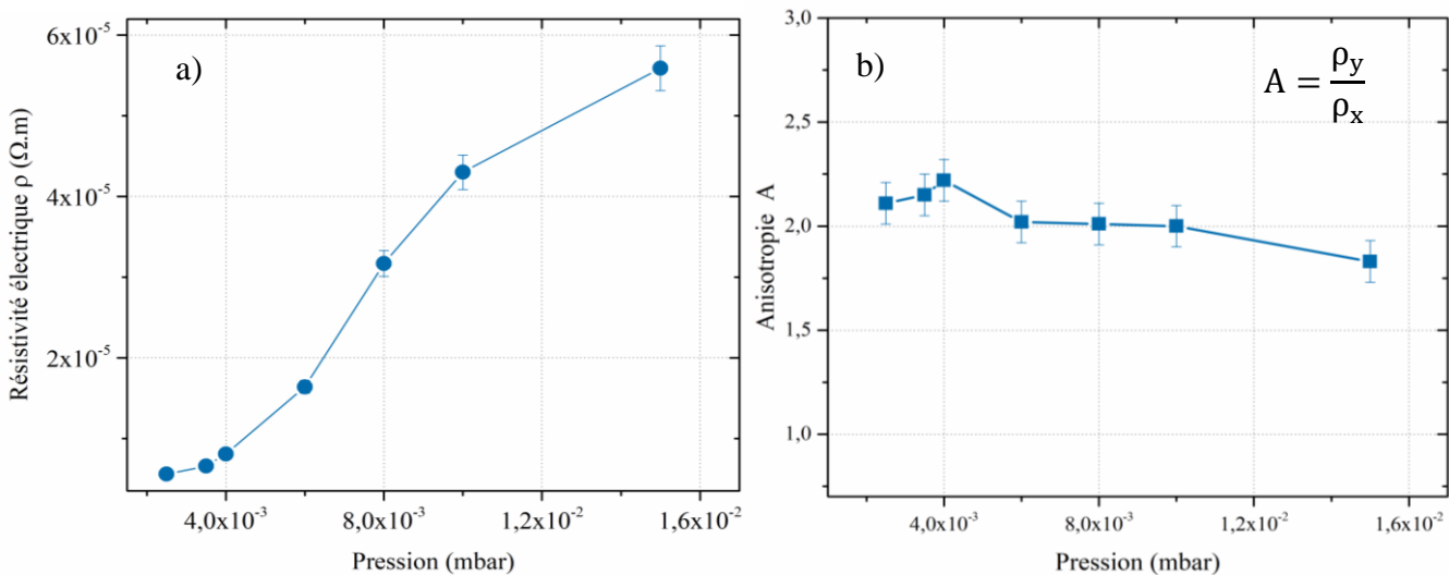
Figure 3.19. Variation a) de la résistivité électrique et b) de l'anisotropie électrique en fonction de la pression de travail.
