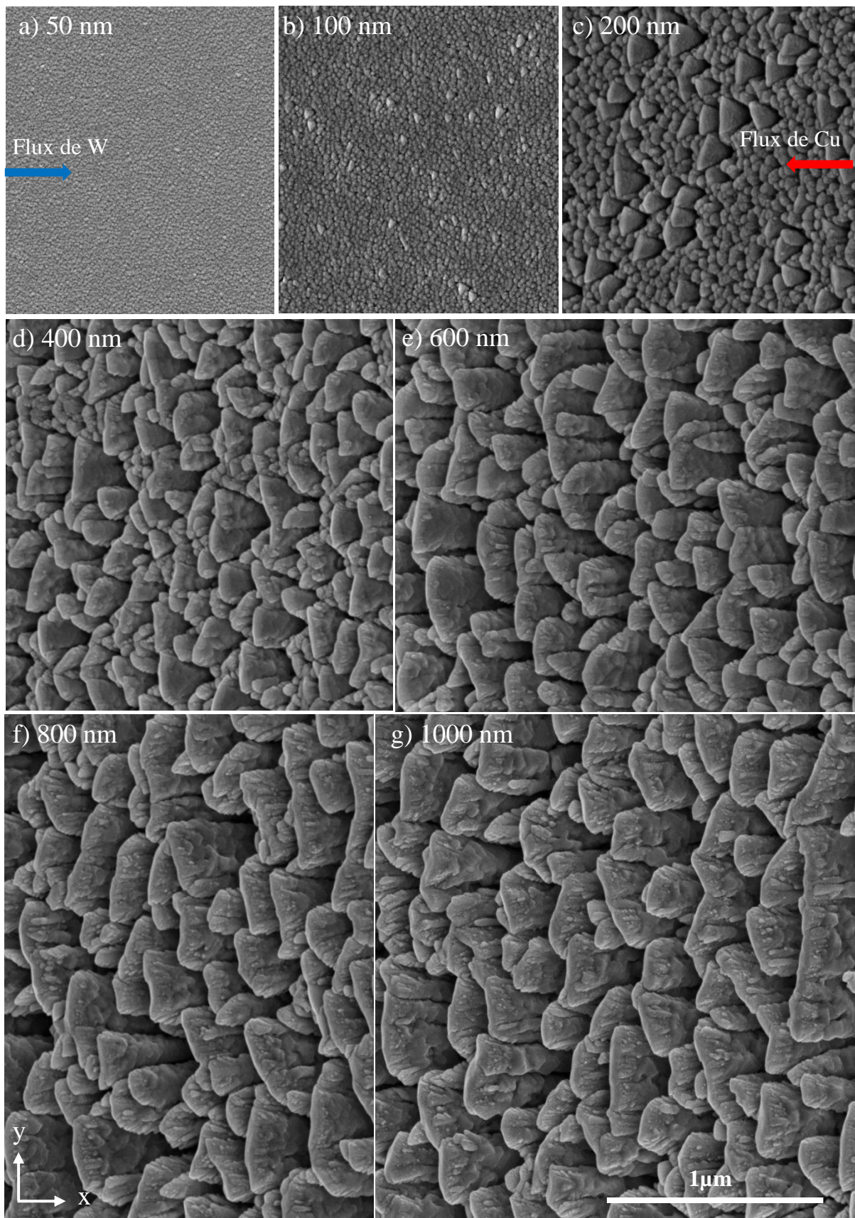
Figure 4.7. Observations MEB en électrons secondaires de la surface des films de W-Cu déposés à p = 4 \times 10^{-3} mbar avec I_W = 140 mA et I_{Cu} = 40 mA. Ces films ont différentes épaisseurs : a) 50 nm, b) 100 nm, c) 200 nm, d) 400 nm, e) 600 nm, f) 800 nm et g) 1000 nm.
