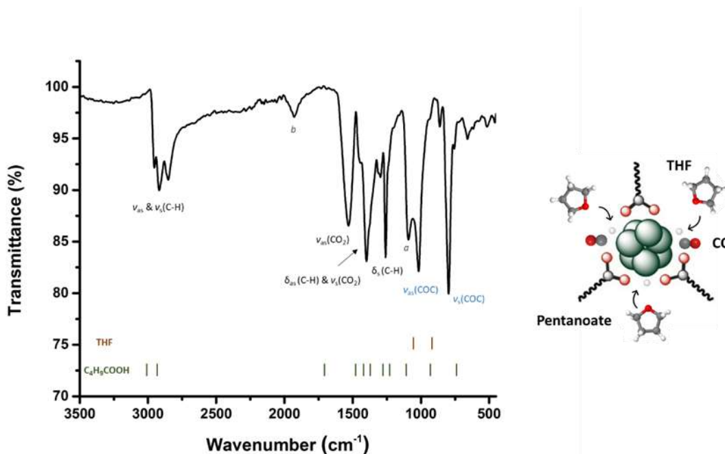
Illustration 9. Spectre IRFT de Ru_x(C_4H_9COO)_{0.4} NPs et indication des principaux pics. Les pics caractéristiques de l'acide pentanoïque (barres vertes, C_4H_9COOH ) et du THF (barres jaunes) sont également indiqués. N : étirement ; \delta : flexion ; s : symétrique ; as : asymétrique. Les pics attribués au THF coordonné à la surface des RuNPs sont également indiqués (bleu). Le signal noté -a- est assigné au PolyTHF et celui noté -b- au CO. Un schéma de la composition de surface des RuNPs est également montré.
