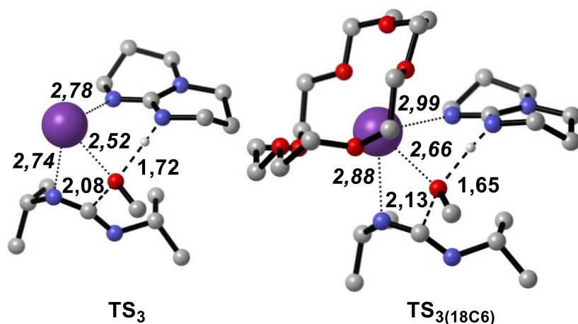
Figure V-27 États de transition calculés avec TBDK en présence ou en l'absence d'éther couronne 18-C-6. Les longueurs de liaison dans la sphère de coordination de K + sont en italique. Distances en Angstrom (Å) Représentation graphique grâce à CYLview [55]
